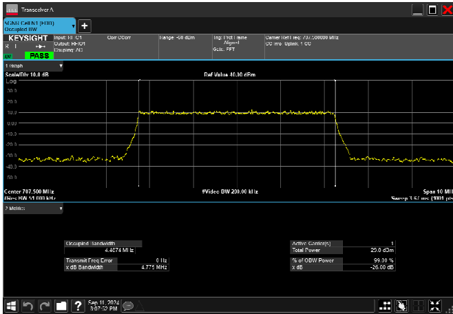
n12_5MHz_15kHz_707.5MHz_CP-OFDM QPSK_RB25@0 4.466MHz
