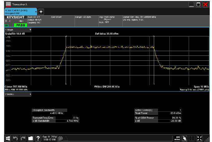
n12_5MHz_15kHz_707.5MHz_CP-OFDM 16 QAM_RB25@0 4.465MHz
