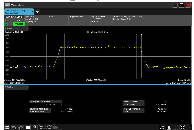
n12_5MHz_15kHz_713.5MHz_CP-OFDM QPSK_RB25@0 4.466MHz
