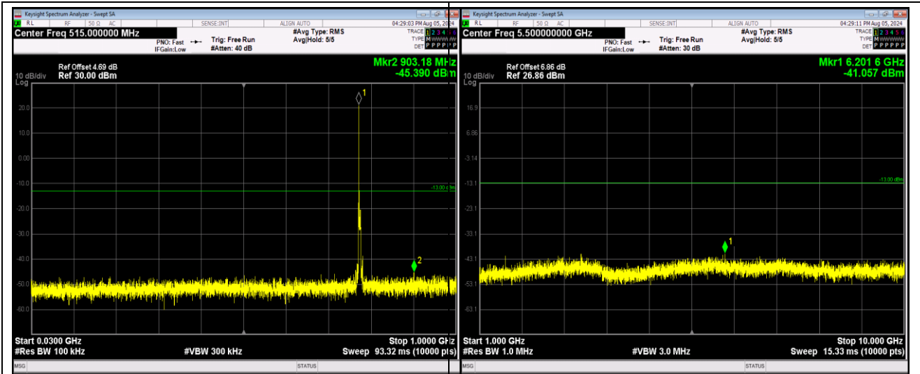
Band13-5MHz-QPSK-23230-1RB#0-Range1:30~1000MHz
