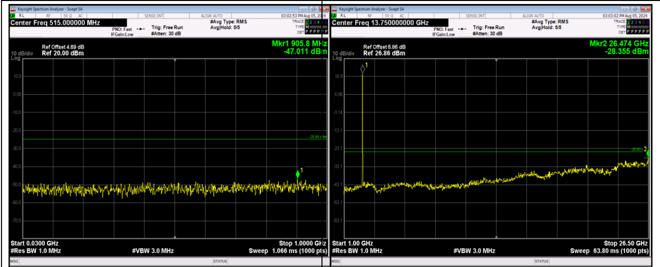
Band12-1.4MHz-QPSK-23017-1RB#0-Range1:30~1000MHz
