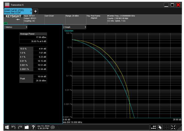
10MHz_15kHz_2535MHz_DFT-s-OFDM 64 QAM_RB50@0&9.23 dB
