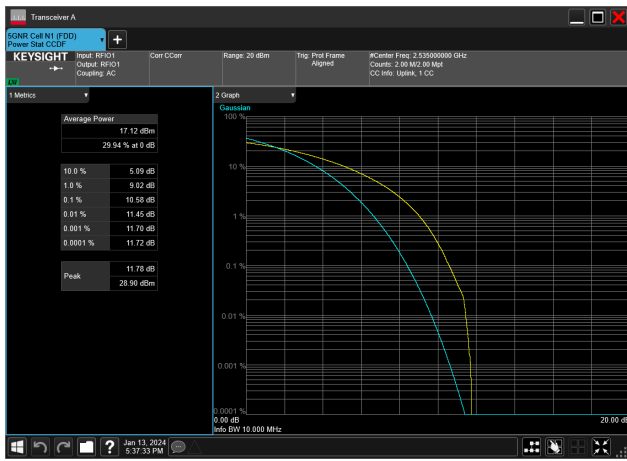
10MHz_15kHz_2535MHz_CP-OFDM QPSK_RB52@0&10.58 dB
