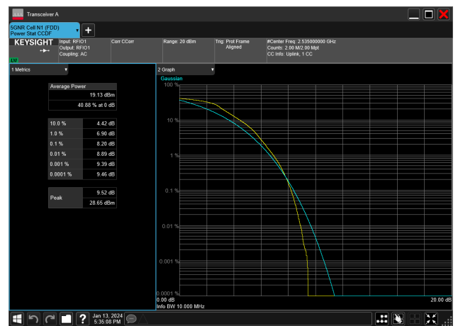
10MHz_15kHz_2535MHz_DFT-s-OFDM QPSK_RB50@0&8.20 dB
