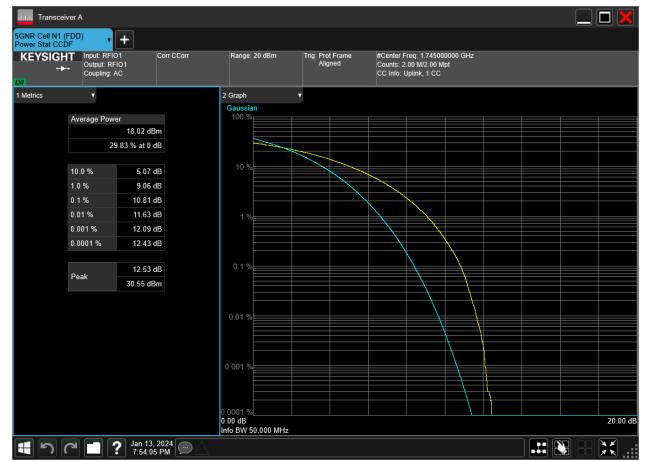
40MHz_15kHz_1745MHz_CP-OFDM QPSK_RB216@0&10.81 dB
