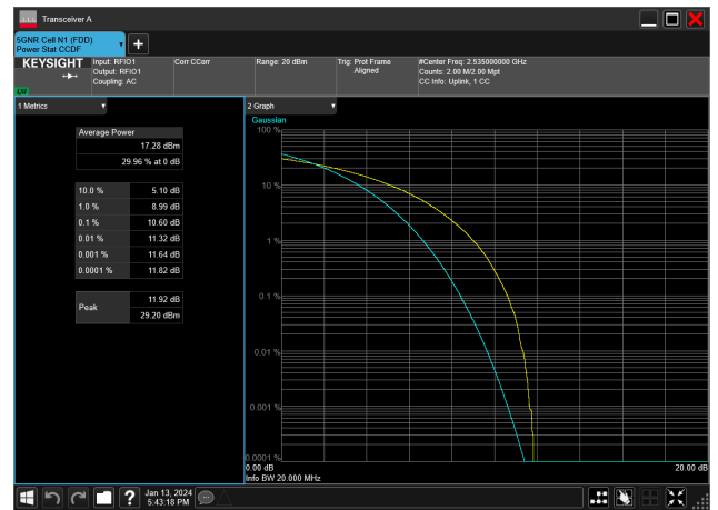
15MHz_15kHz_2535MHz_CP-OFDM QPSK_RB79@0&10.60 dB
