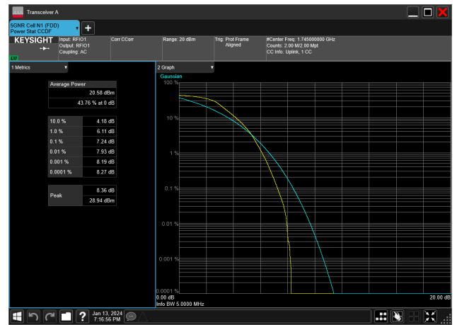
5MHz_15kHz_1745MHz_DFT-s-OFDM PI/2 BPSK_RB25@0&7.24 dB
