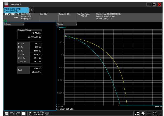
20MHz_15kHz_2535MHz_CP-OFDM 64 QAM_RB106@0&11.00 dB
