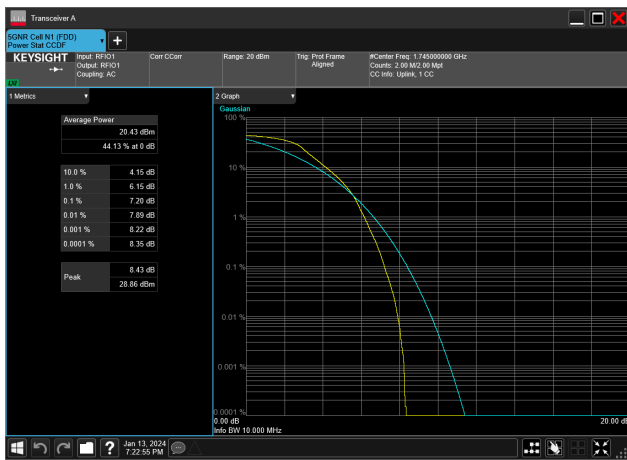
10MHz_15kHz_1745MHz_DFT-s-OFDM PI/2 BPSK_RB50@0&7.20 dB
