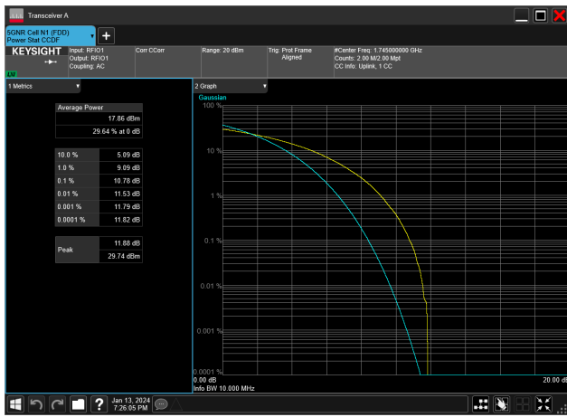
10MHz_15kHz_1745MHz_CP-OFDM QPSK_RB52@0&10.78 dB
