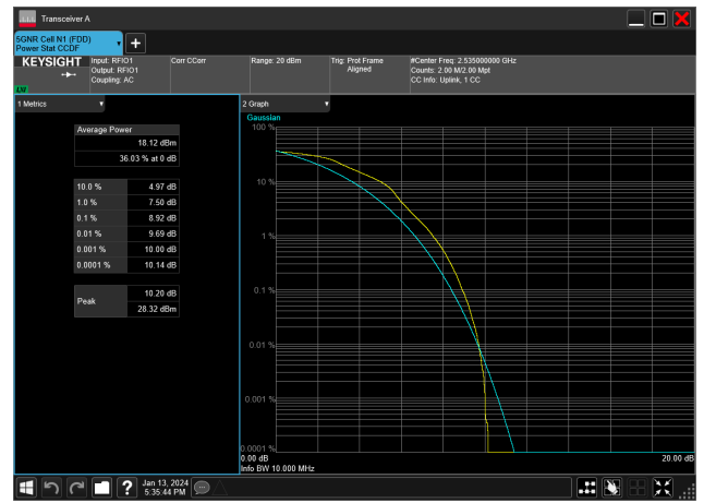
10MHz_15kHz_2535MHz_DFT-s-OFDM 16 QAM_RB50@0&8.92 dB
