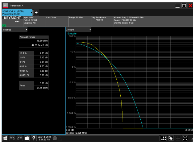
10MHz_15kHz_2535MHz_DFT-s-OFDM PI/2 BPSK_RB50@0&7.05 dB
