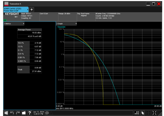
5MHz_15kHz_2535MHz_DFT-s-OFDM PI/2 BPSK_RB25@0&7.12 dB
