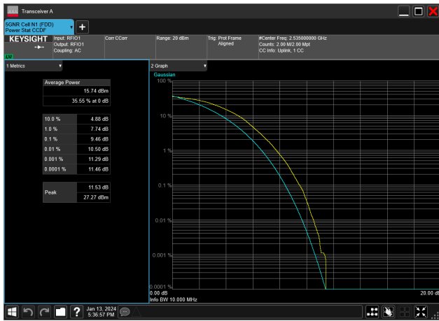
10MHz_15kHz_2535MHz_DFT-s-OFDM 256 QAM_RB50@0&9.46 dB
