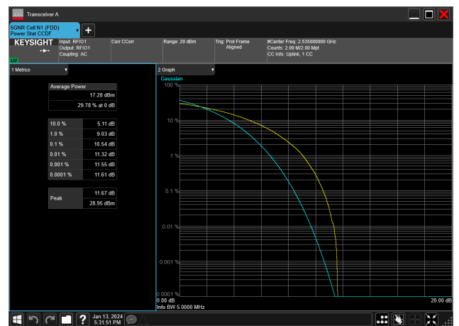
5MHz_15kHz_2535MHz_CP-OFDM QPSK_RB25@0&10.54 dB
