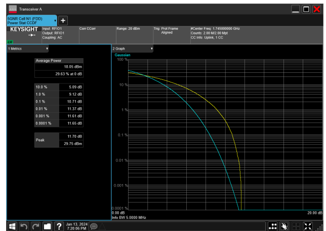
5MHz_15kHz_1745MHz_CP-OFDM QPSK_RB25@0&10.71 dB
