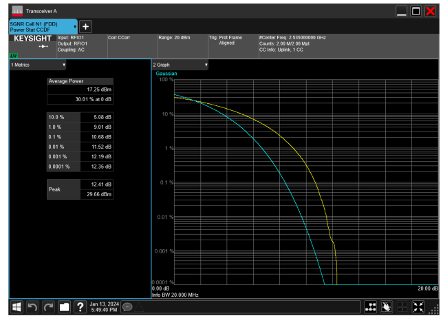
20MHz_15kHz_2535MHz_CP-OFDM 16 QAM_RB106@0&10.68 dB
