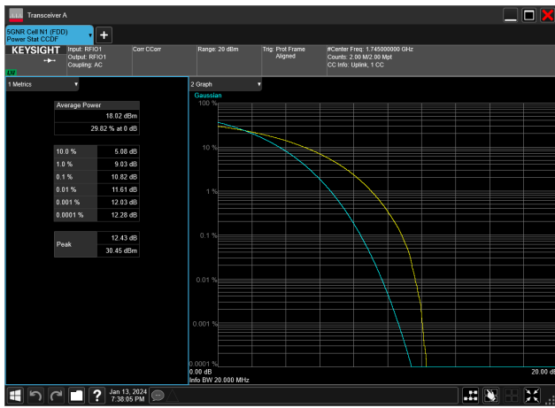
20MHz_15kHz_1745MHz_CP-OFDM QPSK_RB106@0&10.82 dB
