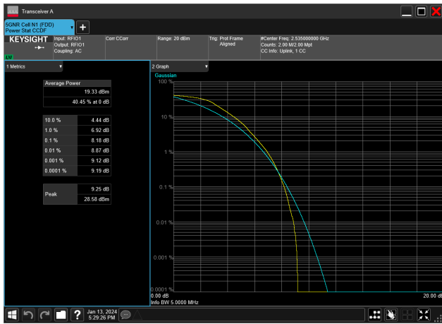
5MHz_15kHz_2535MHz_DFT-s-OFDM QPSK_RB25@0&8.18 dB
