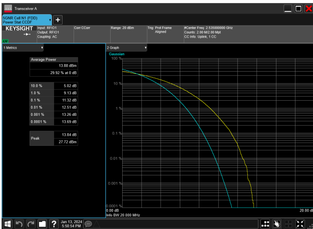
20MHz_15kHz_2535MHz_CP-OFDM 256 QAM_RB106@0&11.32 dB
