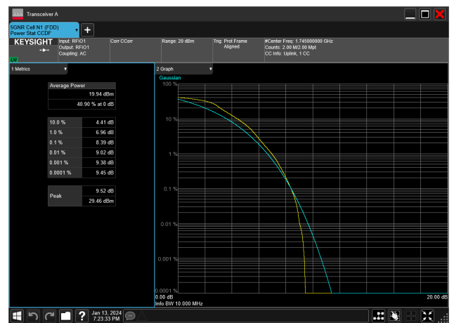
10MHz_15kHz_1745MHz_DFT-s-OFDM QPSK_RB50@0&8.39 dB
