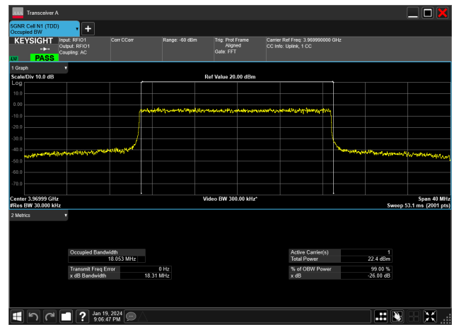
20MHz_30kHz_3970MHz_DFT-s-OFDM QPSK_RB50@0&18.053 MHz
