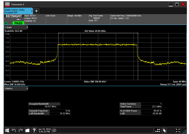
20MHz_30kHz_3840MHz_DFT-s-OFDM PI/2 BPSK_RB50@0&18.017 MHz
