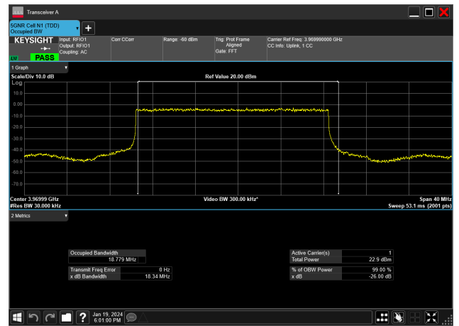
20MHz_15kHz_3970MHz_DFT-s-OFDM PI/2 BPSK_RB100@0&18.779 MHz
