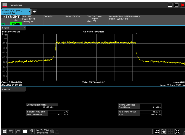
20MHz_30kHz_3970MHz_DFT-s-OFDM 256 QAM_RB50@0&18.018 MHz
