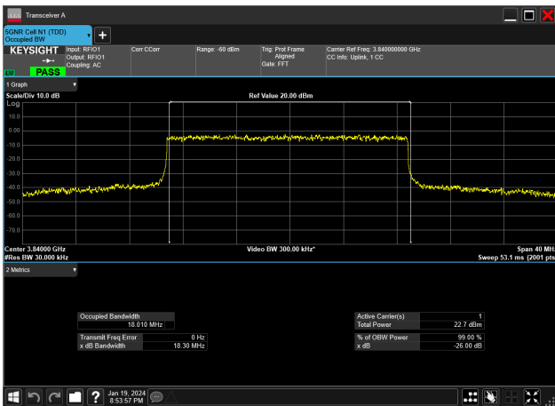
20MHz_30kHz_3840MHz_DFT-s-OFDM QPSK_RB50@0&18.010 MHz
