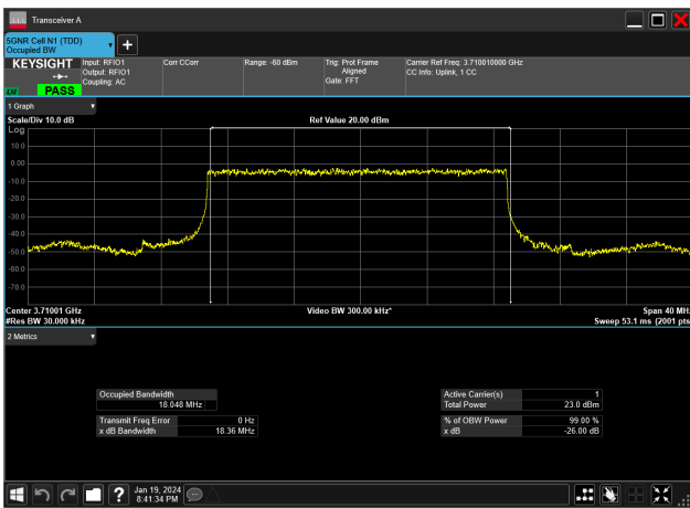
20MHz_30kHz_3710MHz_DFT-s-OFDM PI/2 BPSK_RB50@0&18.048 MHz
