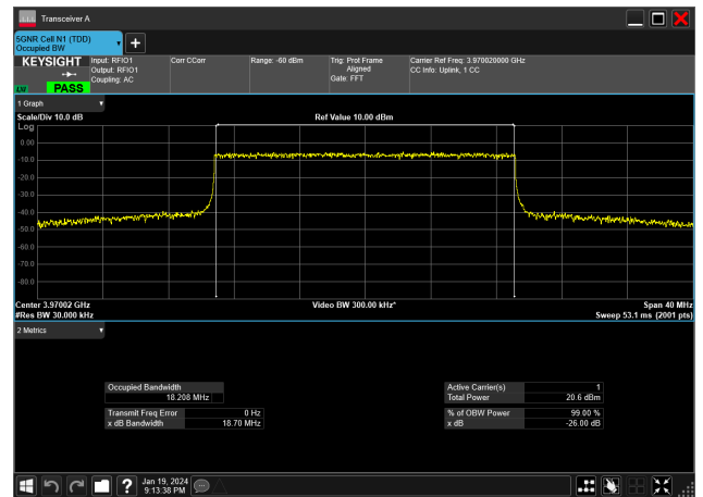
20MHz_30kHz_3970MHz_CP-OFDM 16 QAM_RB51@0&18.208 MHz
