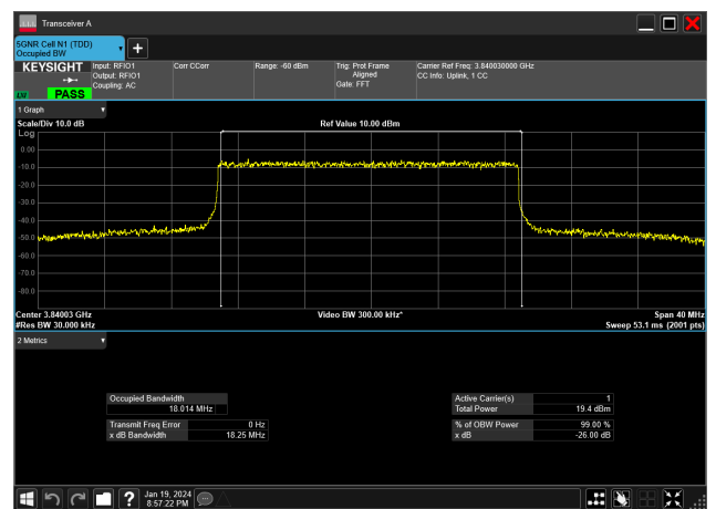
20MHz_30kHz_3840MHz_DFT-s-OFDM 256 QAM_RB50@0&18.014 MHz
