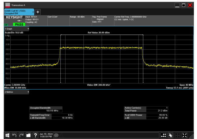
20MHz_30kHz_3970MHz_DFT-s-OFDM 64 QAM_RB50@0&18.018 MHz
