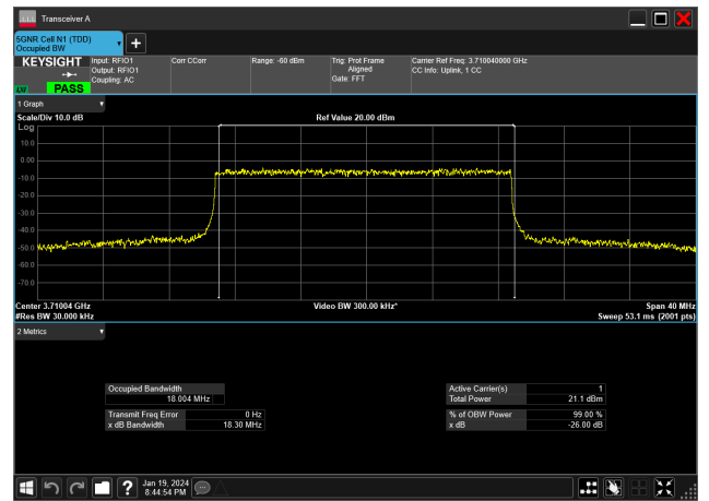
20MHz_30kHz_3710MHz_DFT-s-OFDM 64 QAM_RB50@0&18.004 MHz
