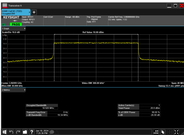
20MHz_15kHz_3970MHz_CP-OFDM 64 QAM_RB106@0&18.920 MHz
