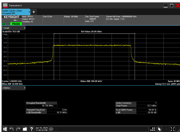
20MHz_15kHz_3970MHz_DFT-s-OFDM QPSK_RB100@0&18.736 MHz
