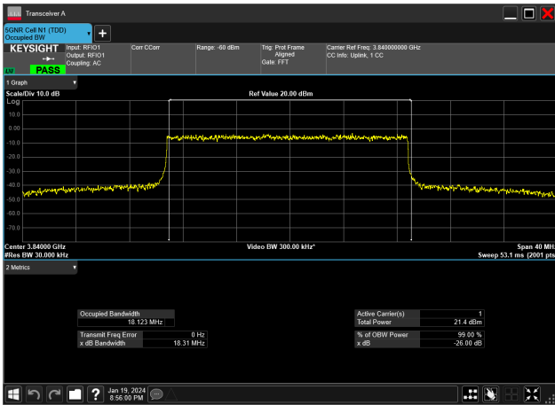
20MHz_30kHz_3840MHz_DFT-s-OFDM 64 QAM_RB50@0&18.123 MHz
