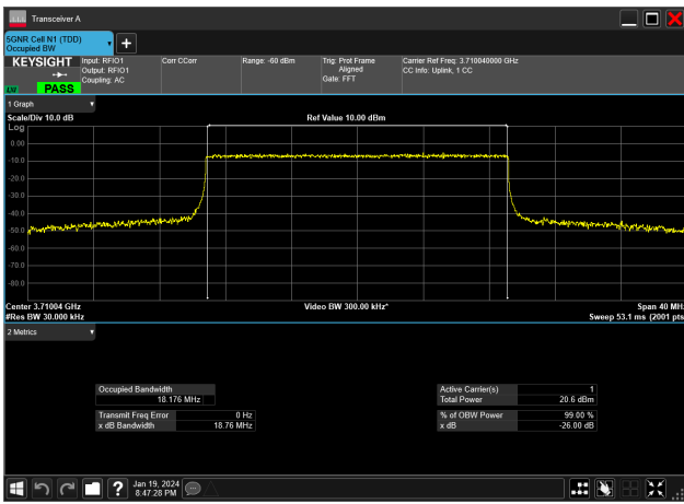
20MHz_30kHz_3710MHz_CP-OFDM QPSK_RB51@0&18.176 MHz
