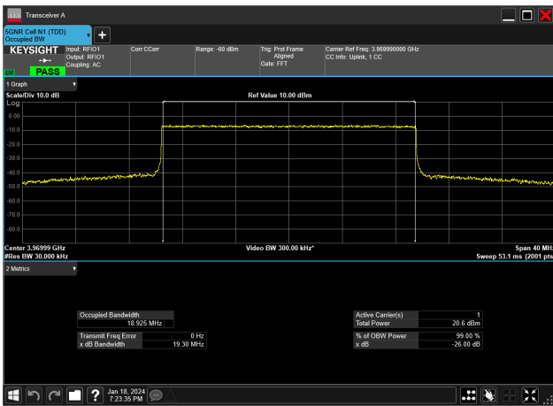
20MHz_15kHz_3970MHz_CP-OFDM 16 QAM_RB106@0&18.925 MHz
