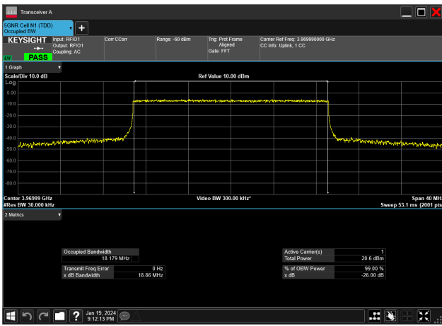
20MHz_30kHz_3970MHz_CP-OFDM QPSK_RB51@0&18.179 MHz
