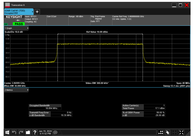
20MHz_15kHz_3970MHz_CP-OFDM 256 QAM_RB106@0&18.894 MHz
