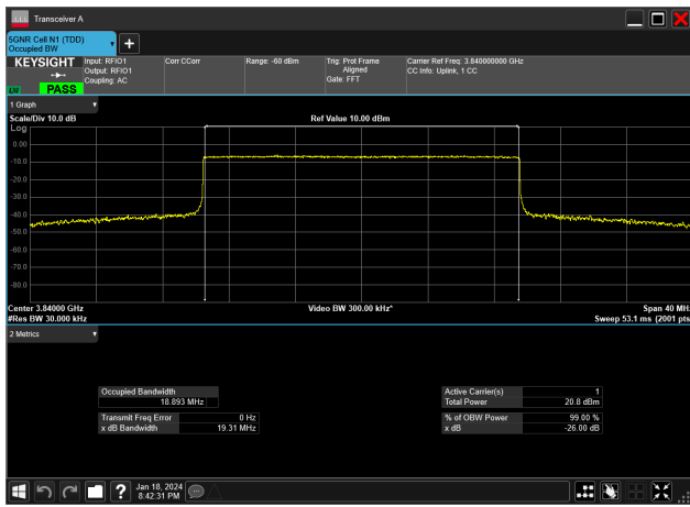
20MHz_15kHz_3840MHz_CP-OFDM QPSK_RB106@0&18.893 MHz
