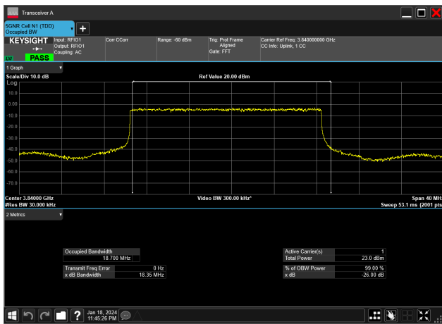
20MHz_15kHz_3840MHz_DFT-s-OFDM PI/2 BPSK_RB100@0&18.700 MHz
