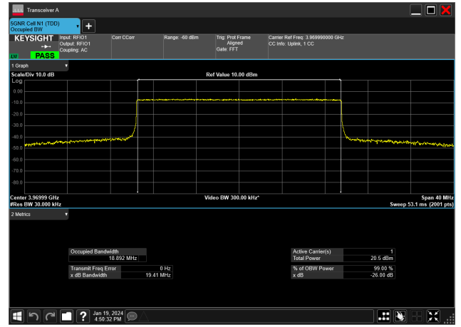
20MHz_15kHz_3970MHz_CP-OFDM QPSK_RB106@0&18.892 MHz
