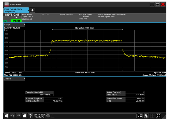
20MHz_30kHz_3970MHz_DFT-s-OFDM 16 QAM_RB50@0&18.010 MHz
