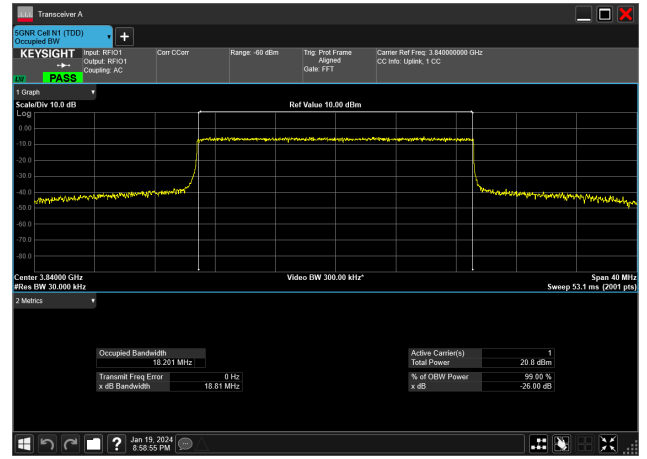
20MHz_30kHz_3840MHz_CP-OFDM QPSK_RB51@0&18.201 MHz
