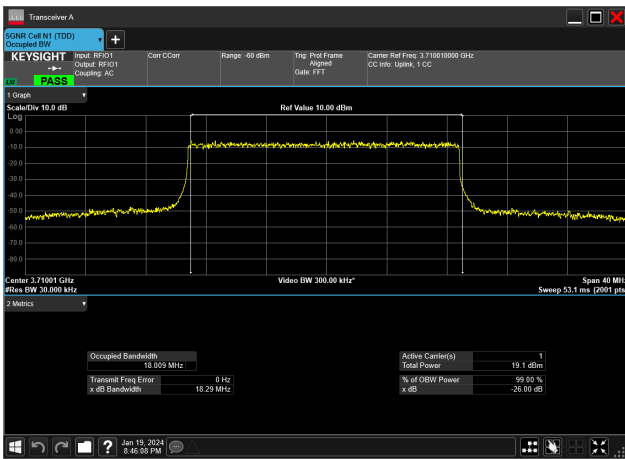
20MHz_30kHz_3710MHz_DFT-s-OFDM 256 QAM_RB50@0&18.009 MHz
