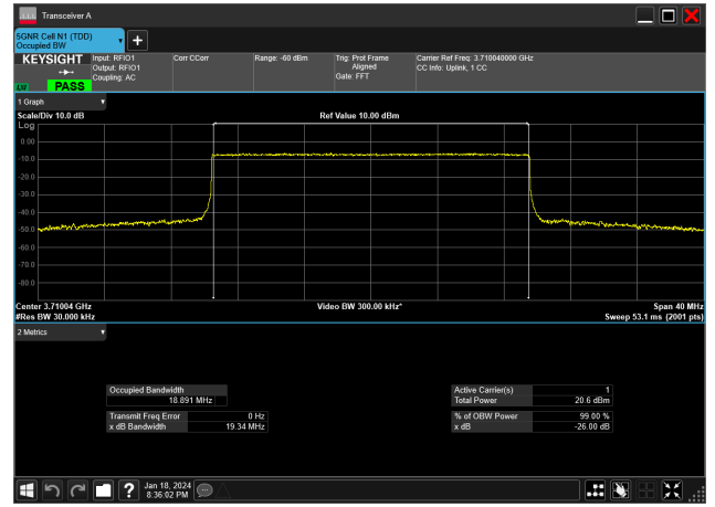
20MHz_15kHz_3710MHz_CP-OFDM QPSK_RB106@0&18.891 MHz
