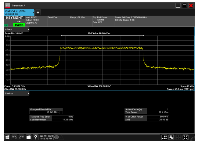
20MHz_30kHz_3710MHz_DFT-s-OFDM QPSK_RB50@0&18.045 MHz
