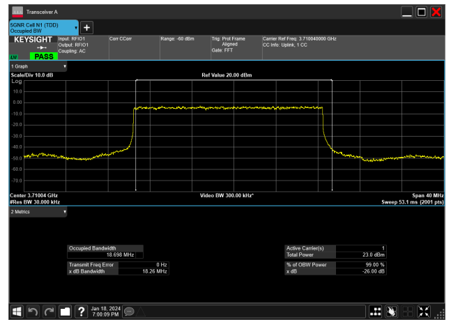
20MHz_15kHz_3710MHz_DFT-s-OFDM PI/2 BPSK_RB100@0&18.698 MHz
