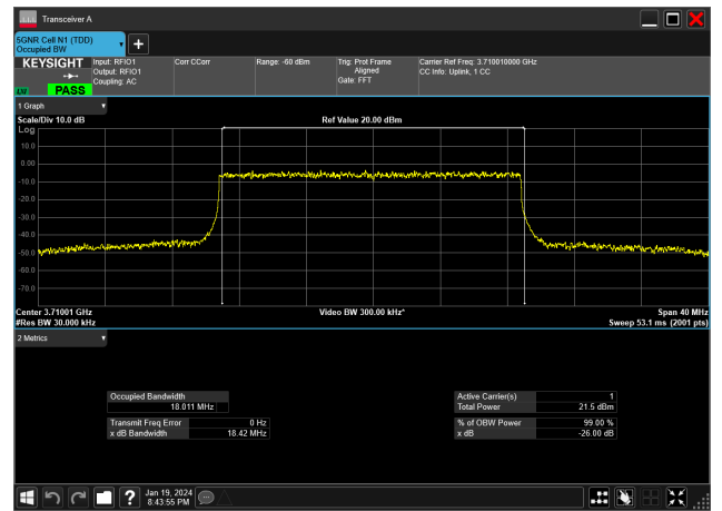
20MHz_30kHz_3710MHz_DFT-s-OFDM 16 QAM_RB50@0&18.011 MHz
