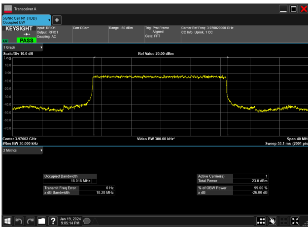
20MHz_30kHz_3970MHz_DFT-s-OFDM PI/2 BPSK_RB50@0&18.018 MHz
