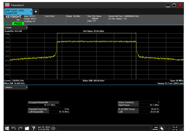
20MHz_30kHz_3970MHz_CP-OFDM 64 QAM_RB51@0&18.171 MHz
