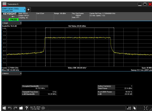
20MHz_15kHz_3710MHz_DFT-s-OFDM QPSK_RB100@0&18.763 MHz
