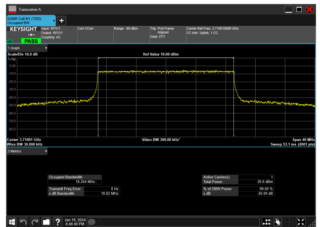
20MHz_30kHz_3710MHz_CP-OFDM 16 QAM_RB51@0&18.204 MHz
