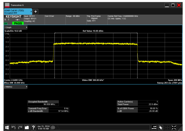
100MHz_30kHz_2640MHz_DFT-s-OFDM QPSK_RB270@0&96.059 MHz
