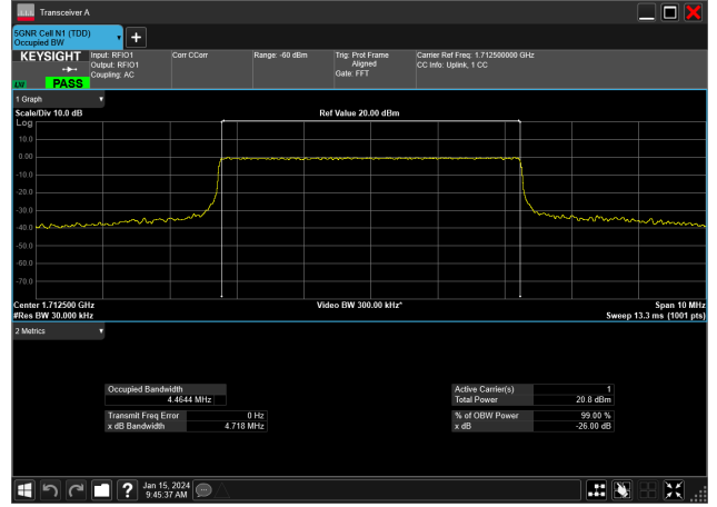
5MHz_15kHz_1712.5MHz_CP-OFDM QPSK_RB25@0&4.464 MHz
