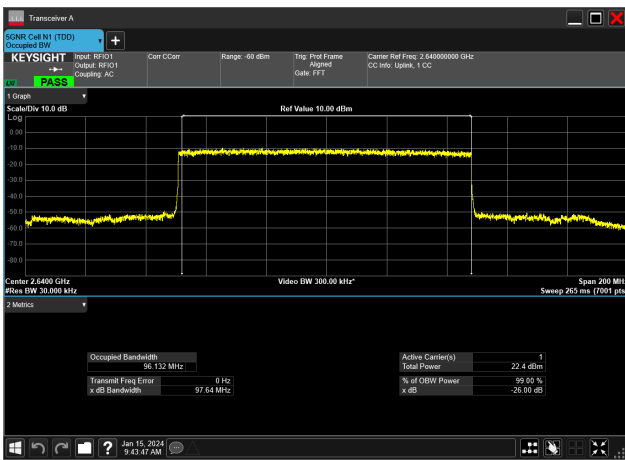
100MHz_30kHz_2640MHz_DFT-s-OFDM PI/2 BPSK_RB270@0&96.132 MHz
