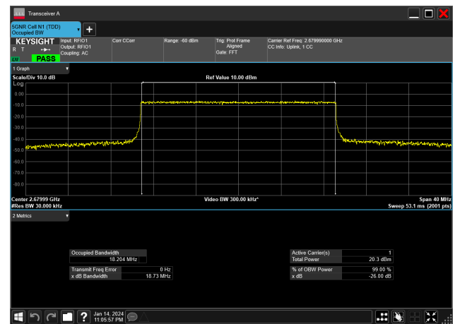
20MHz_30kHz_2679.99MHz_CP-OFDM QPSK_RB51@0&18.204 MHz
