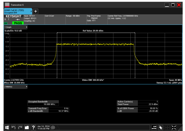
20MHz_30kHz_2679.99MHz_DFT-s-OFDM PI/2 BPSK_RB50@0&18.088 MHz
