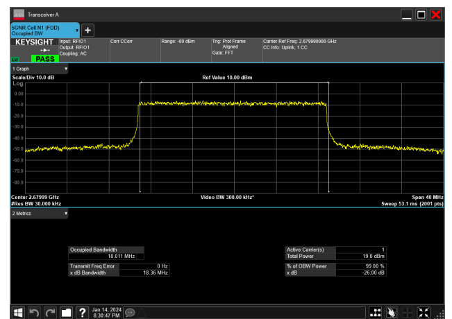
20MHz_30kHz_2679.99MHz_DFT-s-OFDM 256 QAM_RB50@0&18.011 MHz
