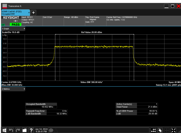
20MHz_30kHz_2679.99MHz_DFT-s-OFDM 16 QAM_RB50@0&18.052 MHz
