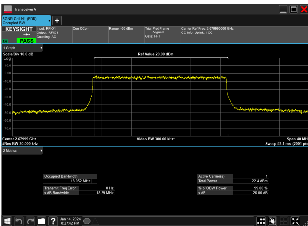
20MHz_30kHz_2679.99MHz_DFT-s-OFDM QPSK_RB50@0&18.052 MHz
