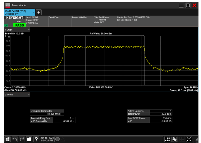
10MHz_30kHz_2355MHz_DFT-s-OFDM PI/2 BPSK_RB24@0&8.540 MHz
