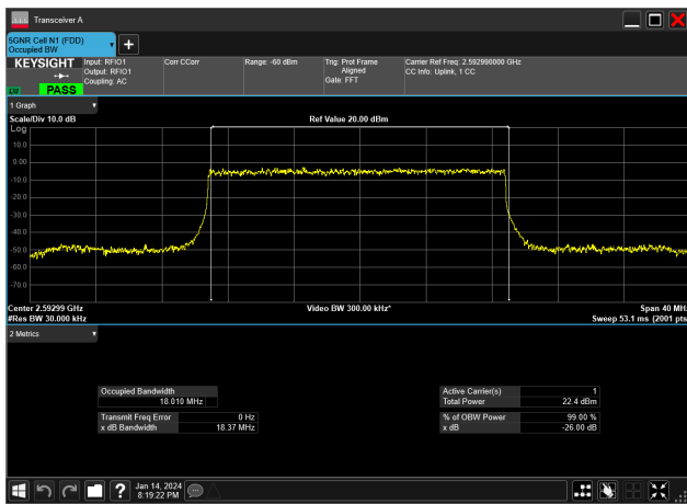
20MHz_30kHz_2592.99MHz_DFT-s-OFDM PI/2 BPSK_RB50@0&18.010 MHz
