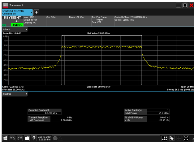
10MHz_30kHz_2355MHz_DFT-s-OFDM QPSK_RB24@0&8.570 MHz
