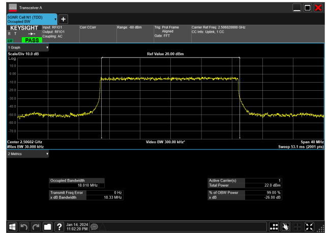
20MHz_30kHz_2506.02MHz_DFT-s-OFDM 16 QAM_RB50@0&18.010 MHz
