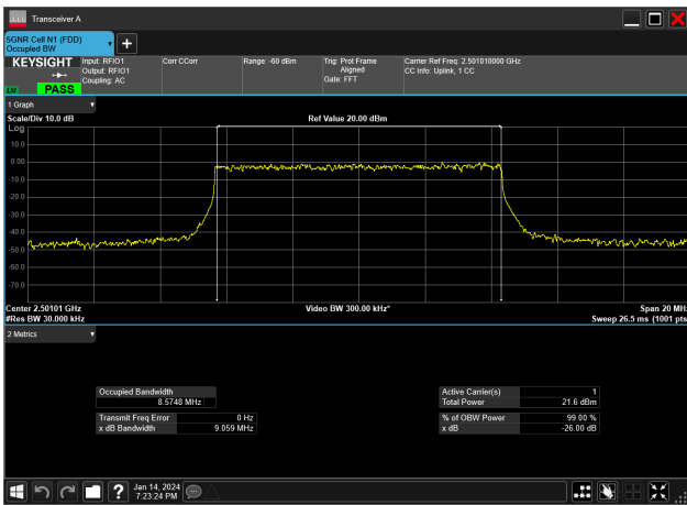
10MHz_30kHz_2501.01MHz_DFT-s-OFDM QPSK_RB24@0&8.575 MHz
