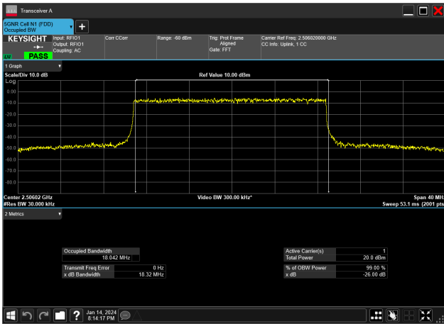
20MHz_30kHz_2506.02MHz_DFT-s-OFDM 64 QAM_RB50@0&18.042 MHz
