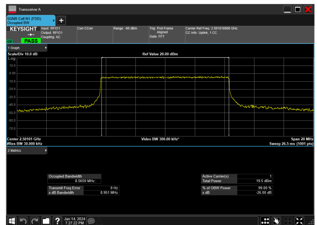
10MHz_30kHz_2501.01MHz_CP-OFDM QPSK_RB24@0&amp;8.566 MHz
