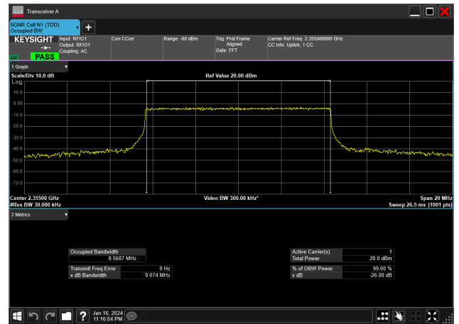
10MHz_30kHz_2355MHz_CP-OFDM QPSK_RB24@0&8.569 MHz
