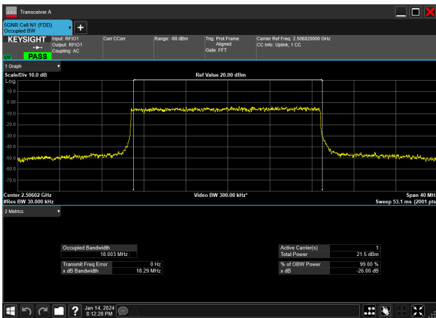
20MHz_30kHz_2506.02MHz_DFT-s-OFDM QPSK_RB50@0&18.003 MHz
