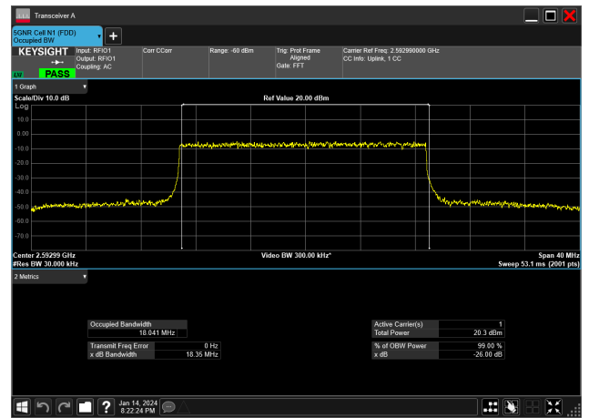
20MHz_30kHz_2592.99MHz_DFT-s-OFDM 64 QAM_RB50@0&18.041 MHz
