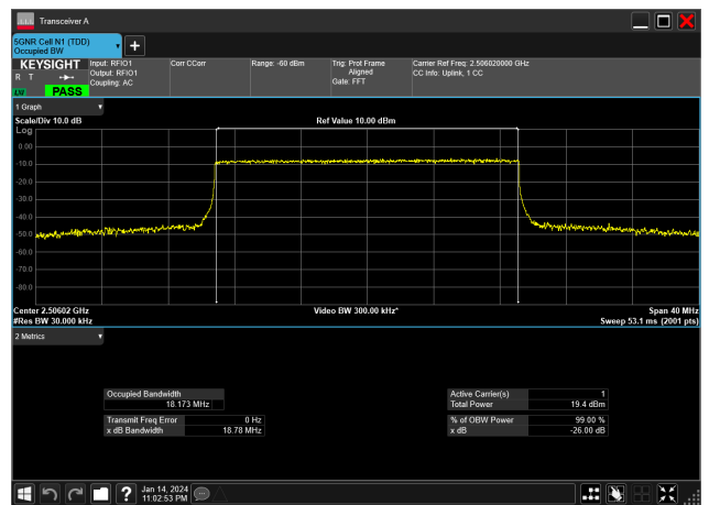
20MHz_30kHz_2506.02MHz_CP-OFDM QPSK_RB51@0&18.173 MHz
