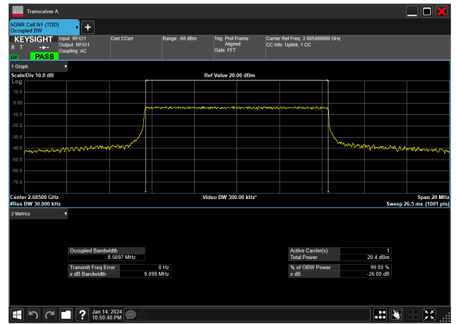
10MHz_30kHz_2685MHz_CP-OFDM QPSK_RB24@0&8.570 MHz
