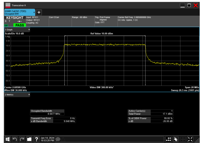
10MHz_30kHz_2685MHz_CP-OFDM 256 QAM_RB24@0&8.568 MHz
