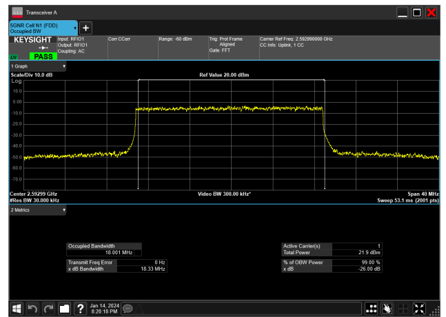
20MHz_30kHz_2592.99MHz_DFT-s-OFDM QPSK_RB50@0&18.001 MHz
