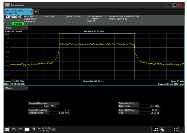
10MHz_30kHz_2595MHz_DFT-s-OFDM QPSK_RB24@0&8.573 MHz
