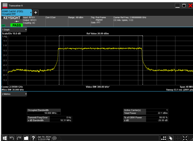
20MHz_30kHz_2595MHz_DFT-s-OFDM PI/2 BPSK_RB50@0&18.000 MHz
