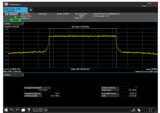
20MHz_30kHz_2610MHz_DFT-s-OFDM 256 QAM_RB50@0&17.975 MHz
