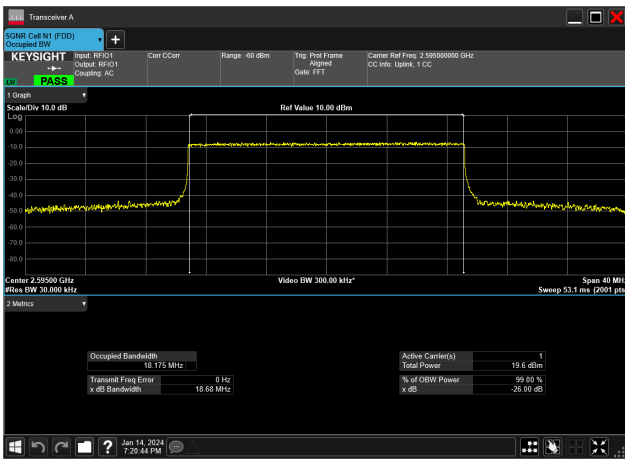
20MHz_30kHz_2595MHz_CP-OFDM QPSK_RB51@0&18.175 MHz
