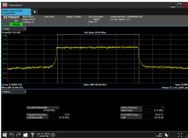
20MHz_30kHz_2580MHz_DFT-s-OFDM QPSK_RB50@0&18.000 MHz
