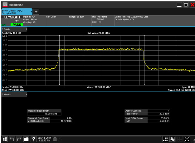
20MHz_30kHz_2580MHz_DFT-s-OFDM 64 QAM_RB50@0&18.050 MHz
