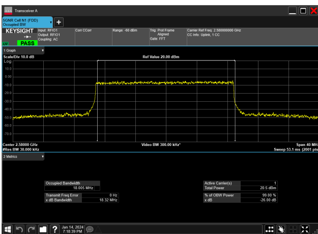
20MHz_30kHz_2580MHz_DFT-s-OFDM 16 QAM_RB50@0&18.005 MHz
