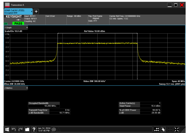
20MHz_30kHz_2610MHz_CP-OFDM 256 QAM_RB51@0&18.200 MHz
