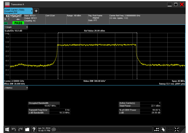
20MHz_30kHz_2580MHz_DFT-s-OFDM PI/2 BPSK_RB50@0&18.057 MHz
