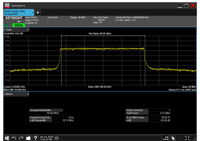
20MHz_30kHz_2595MHz_DFT-s-OFDM QPSK_RB50@0&18.004 MHz
