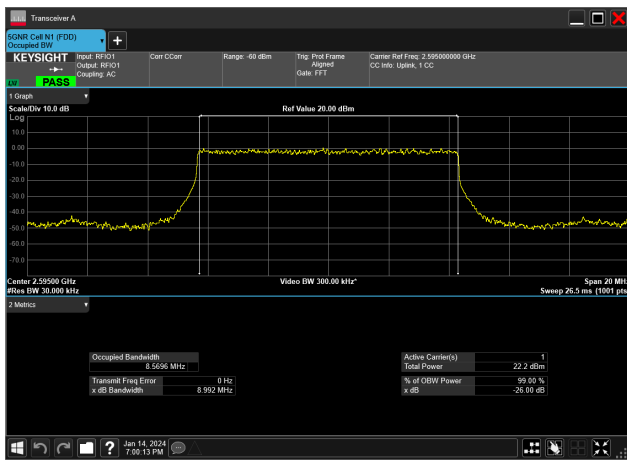
10MHz_30kHz_2595MHz_DFT-s-OFDM PI/2 BPSK_RB24@0&8.570 MHz
