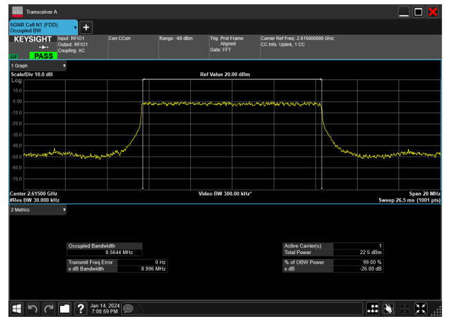
10MHz_30kHz_2615MHz_DFT-s-OFDM PI/2 BPSK_RB24@0&8.564 MHz
