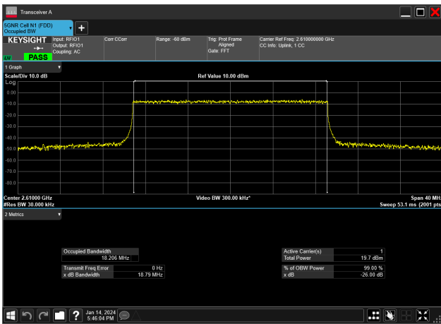
20MHz_30kHz_2610MHz_CP-OFDM 16 QAM_RB51@0&18.206 MHz
