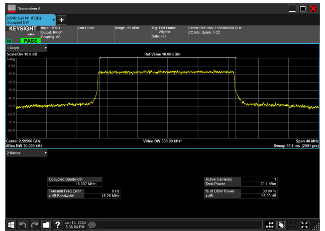
20MHz_30kHz_2595MHz_DFT-s-OFDM 64 QAM_RB50@0&18.007 MHz
