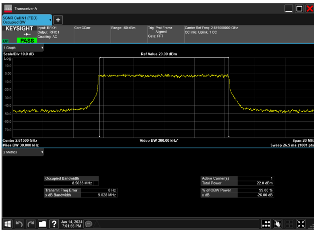
10MHz_30kHz_2615MHz_DFT-s-OFDM QPSK_RB24@0&8.563 MHz
