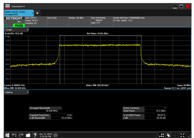
20MHz_30kHz_2580MHz_DFT-s-OFDM 256 QAM_RB50@0&18.008 MHz
