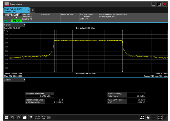
10MHz_30kHz_2615MHz_CP-OFDM QPSK_RB24@0&8.571 MHz
