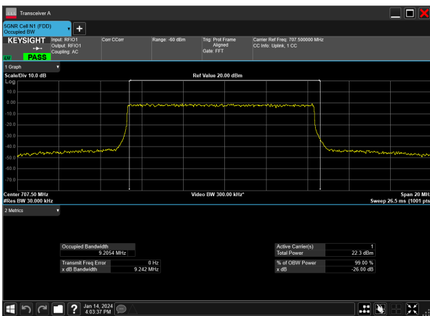
10MHz_15kHz_707.5MHz_DFT-s-OFDM QPSK_RB50@0&9.205 MHz
