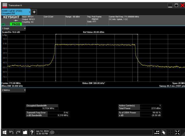
10MHz_15kHz_711MHz_DFT-s-OFDM PI/2 BPSK_RB50@0&9.215 MHz
