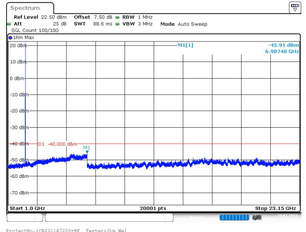
10MHz_30kHz_2310MHz_DFT-s-OFDM QPSK_RB1@0 -45.91 dBm
