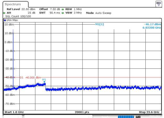
10MHz_30kHz_2355MHz_DFT-s-OFDM QPSK_RB1@0 -46.17 dBm
