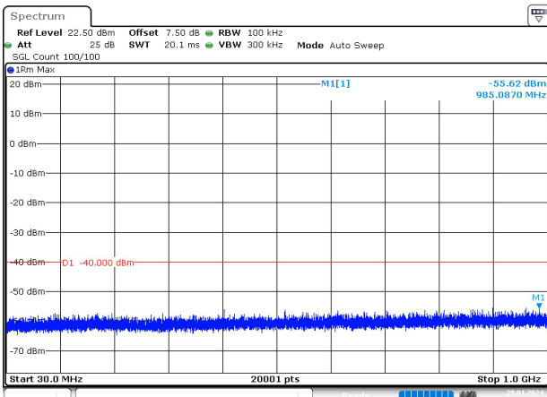
10MHz_30kHz_2355MHz_DFT-s-OFDM QPSK_RB24@0 -55.62 dBm
