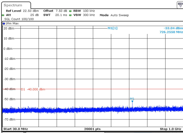
10MHz_30kHz_2355MHz_DFT-s-OFDM QPSK_RB1@23 -53.04 dBm
