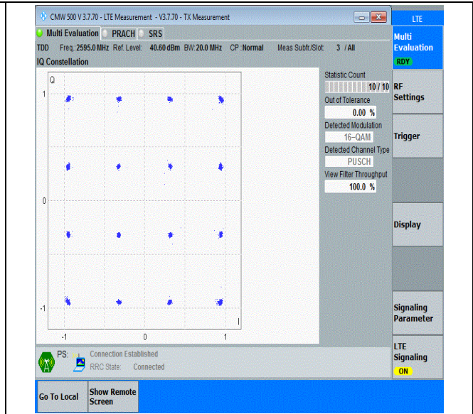
41(2535-2655)-20MHz-16QAM-40640-100RB#0-PASS
