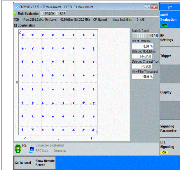
41(2535-2655)-20MHz-64QAM-40640-100RB#0-PASS
