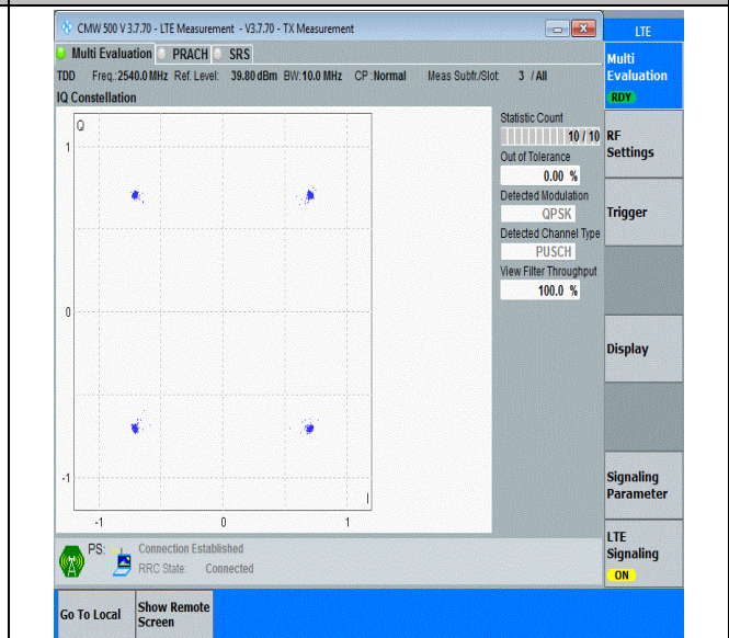
41(2535-2655)-10MHz-QPSK-40090-50RB#0-PASS
