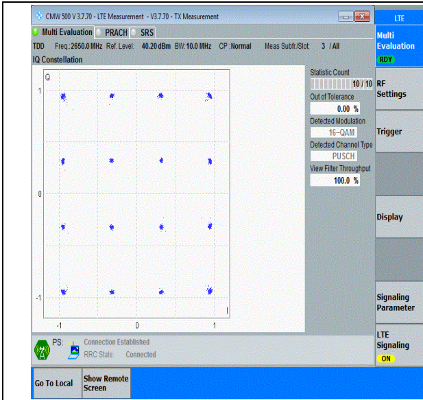
41(2535-2655)-10MHz-16QAM-41190-50RB#0-PASS
