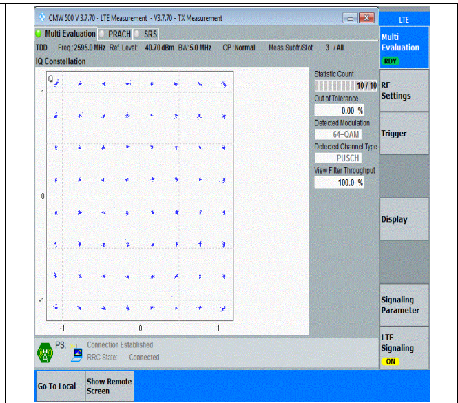
41(2535-2655)-5MHz-64QAM-40640-25RB#0-PASS
