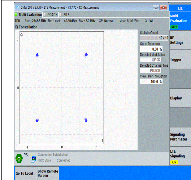
41(2535-2655)-15MHz-QPSK-41165-75RB#0-PASS
