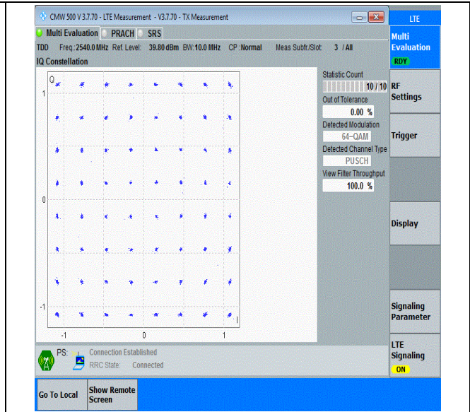
41(2535-2655)-10MHz-64QAM-40090-50RB#0-PASS
