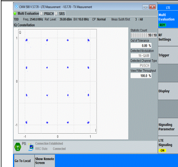
41(2535-2655)-10MHz-16QAM-40090-50RB#0-PASS
