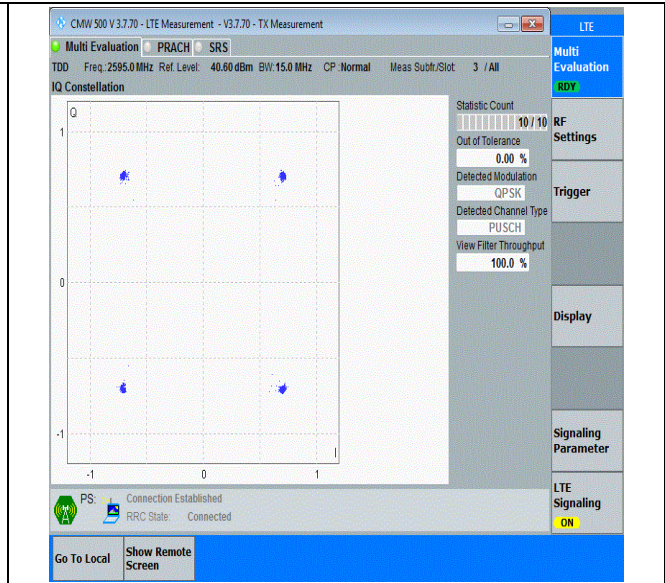
41(2535-2655)-15MHz-QPSK-40640-75RB#0-PASS
