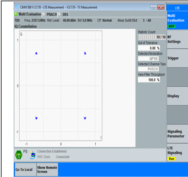
40(2350-2360)-5MHz-QPSK-39225-25RB#0-PASS
