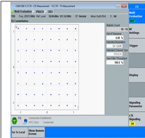
41(2535-2655)-5MHz-64QAM-40065-25RB#0-PASS
