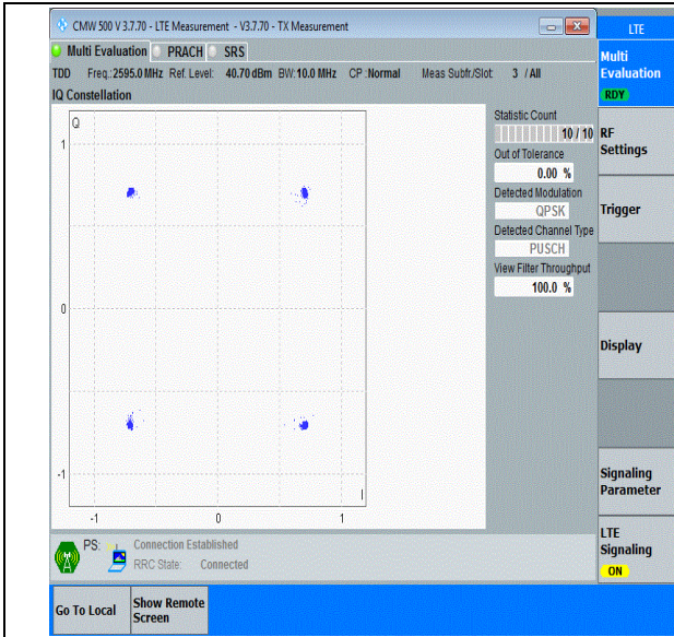
41(2535-2655)-10MHz-QPSK-40640-50RB#0-PASS
