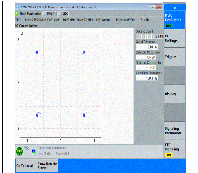
41(2535-2655)-10MHz-QPSK-41190-50RB#0-PASS
