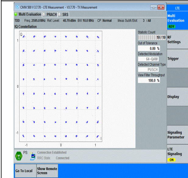
41(2535-2655)-10MHz-64QAM-40640-50RB#0-PASS
