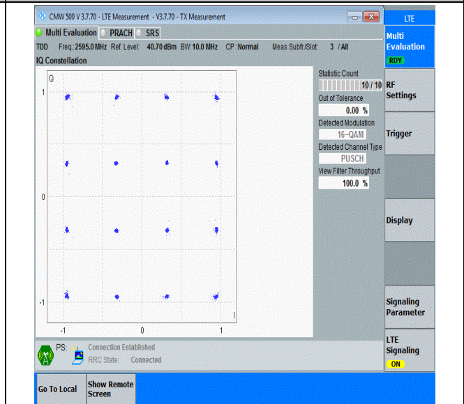
41(2535-2655)-10MHz-16QAM-40640-50RB#0-PASS
