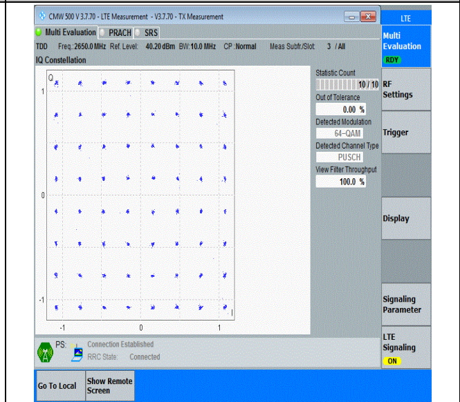
41(2535-2655)-10MHz-64QAM-41190-50RB#0-PASS
