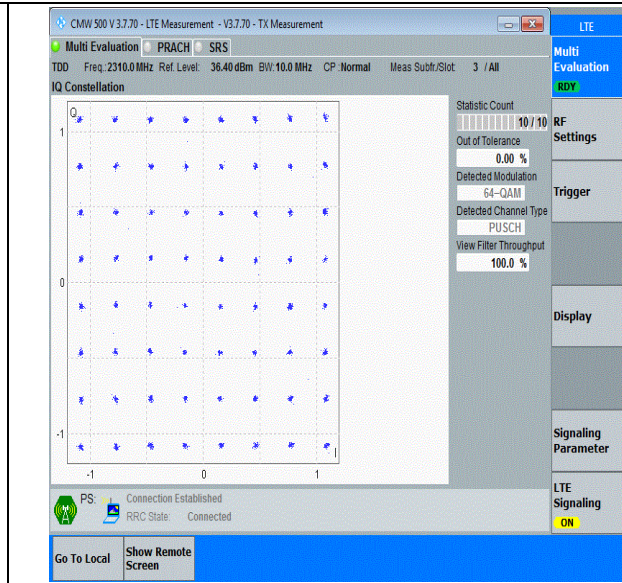
40(2305-2315)-10MHz-64QAM-38750-50RB#0-PASS
