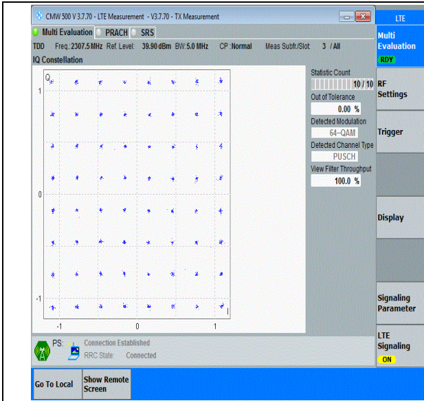
40(2305-2315)-5MHz-64QAM-38725-25RB#0-PASS
