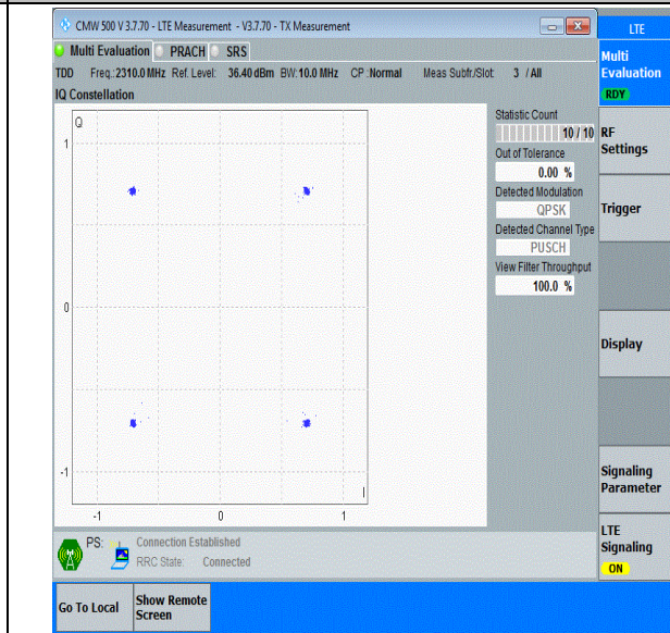
40(2305-2315)-10MHz-QPSK-38750-50RB#0-PASS
