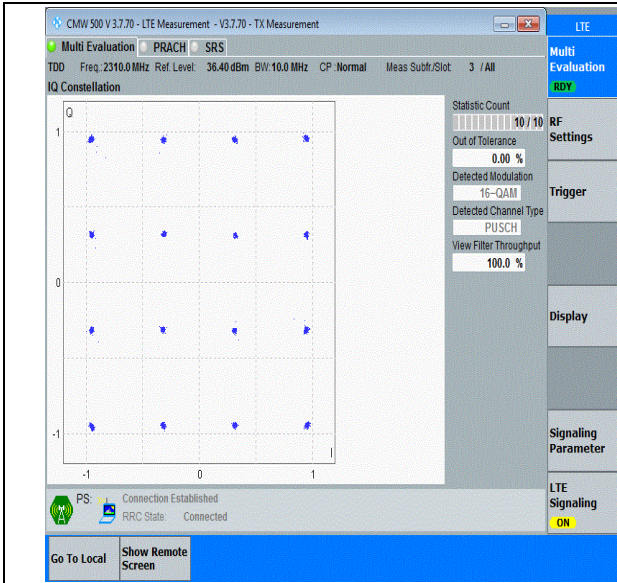
40(2305-2315)-10MHz-16QAM-38750-50RB#0-PASS
