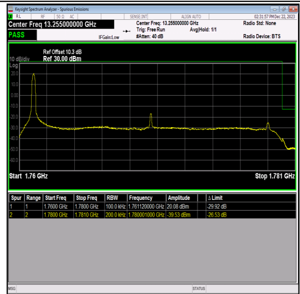
Band66_20MHz_QPSK_132572_1RB#0
