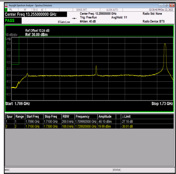
Band66_20MHz_QPSK_132072_1RB#99
