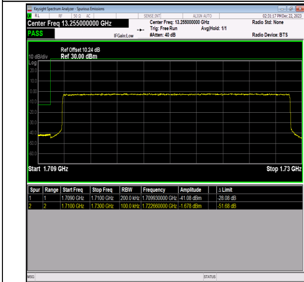
Band66_20MHz_QPSK_132072_100RB#0
