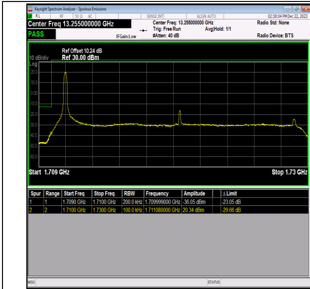
Band66_20MHz_QPSK_132072_1RB#0
