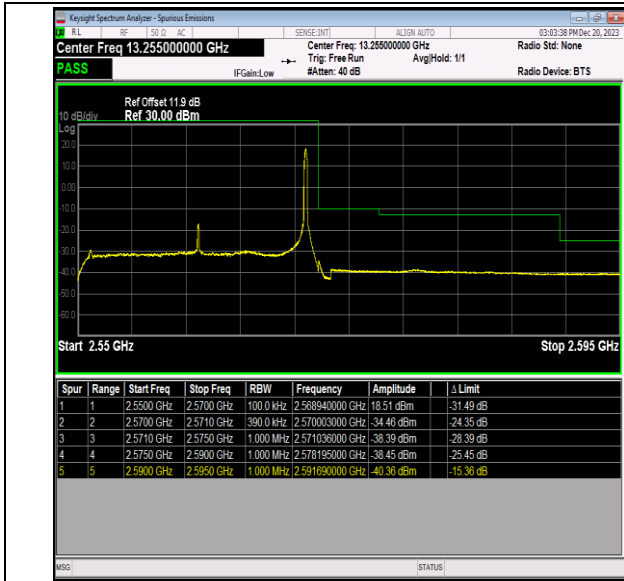
Band7_20MHz_16QAM_21350_1RB#99
