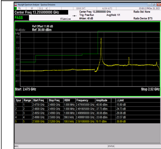
Band7_20MHz_QPSK_20850_1RB#0
