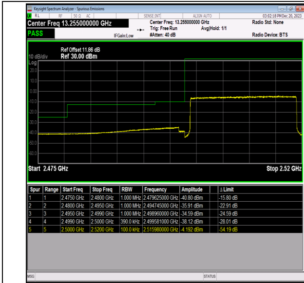
Band7_20MHz_64QAM_20850_100RB#0
