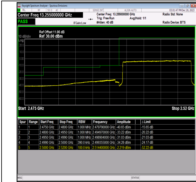
Band7_20MHz_QPSK_20850_100RB#0
