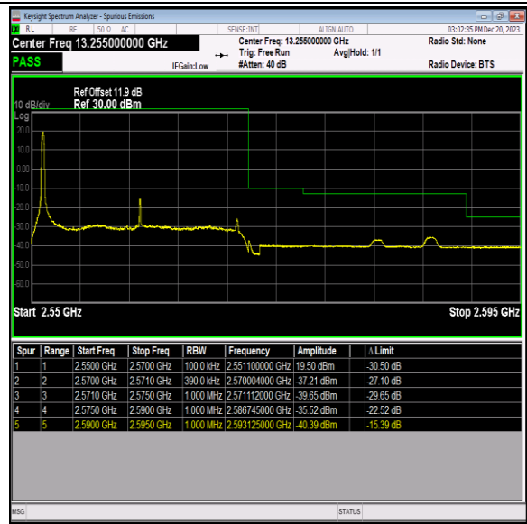
Band7_20MHz_QPSK_21350_1RB#0
