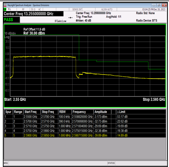
Band7_20MHz_16QAM_21350_100RB#0
