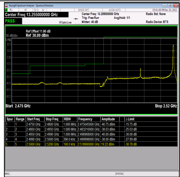
Band7_20MHz_QPSK_20850_1RB#99
