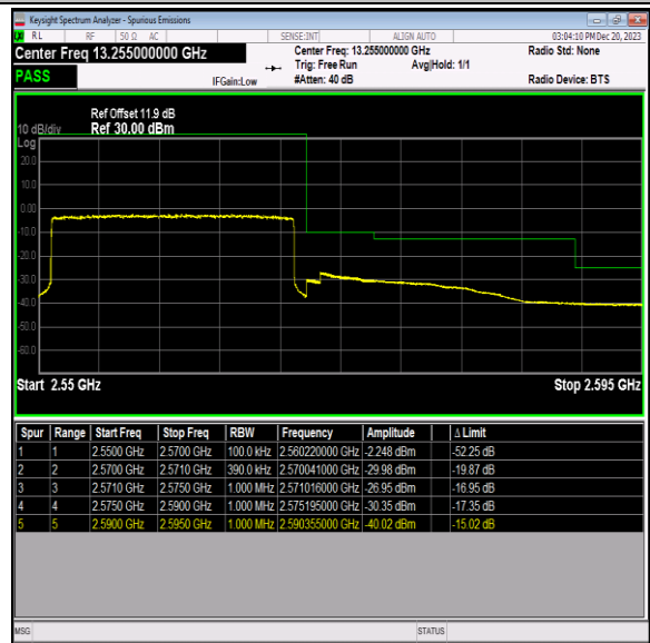
Band7_20MHz_QPSK_21350_100RB#0
