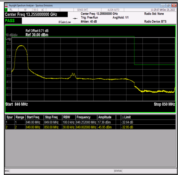
Band5_3MHz_64QAM_20635_1RB#0
