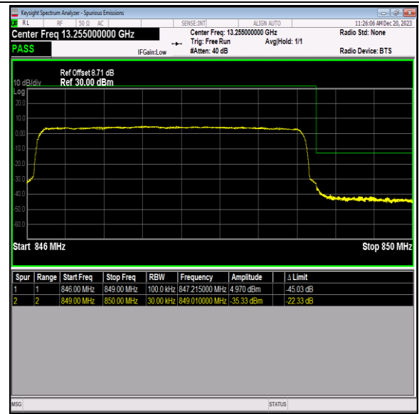
Band5_3MHz_16QAM_20635_15RB#0
