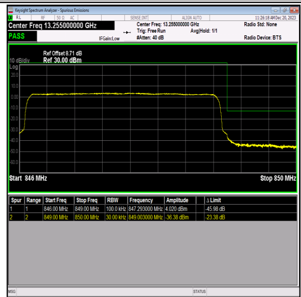
Band5_3MHz_64QAM_20635_15RB#0
