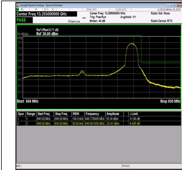
Band5_3MHz_16QAM_20635_1RB#14
