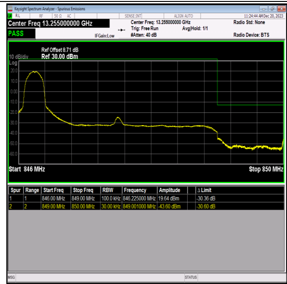
Band5_3MHz_QPSK_20635_1RB#0
