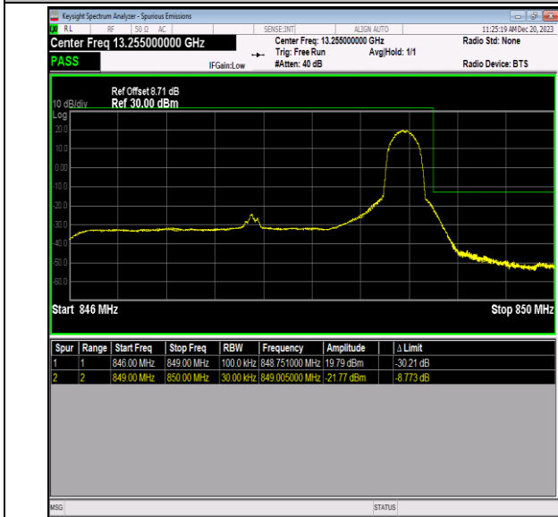
Band5_3MHz_QPSK_20635_1RB#14
