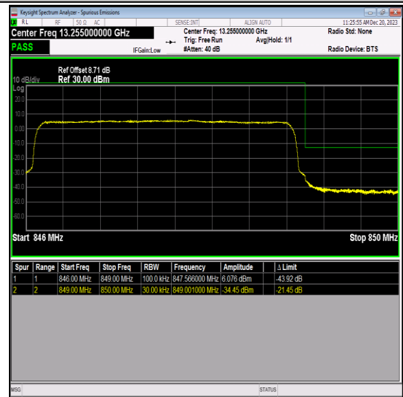
Band5_3MHz_QPSK_20635_15RB#0
