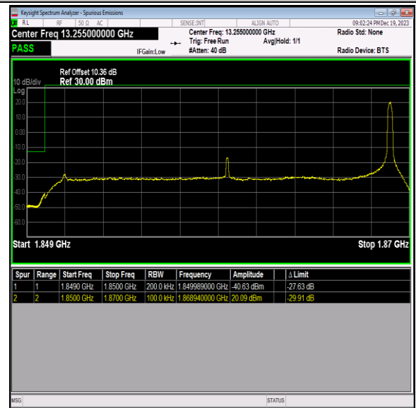
Band2_20MHz_QPSK_18700_1RB#99
