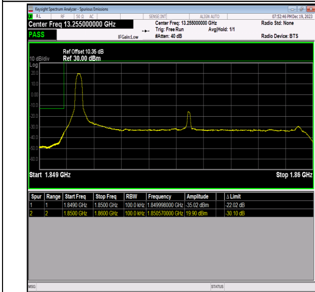
Band2_10MHz_QPSK_18650_1RB#0
