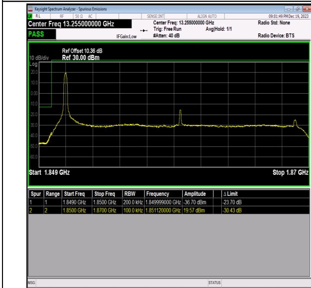
Band2_20MHz_QPSK_18700_1RB#0
