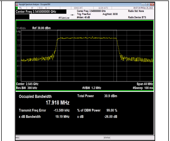
41(2535-2655)-20MHz-QPSK-40140-100RB#0-PASS
