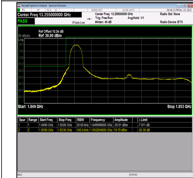
Band2_3MHz_QPSK_18615_1RB#0
