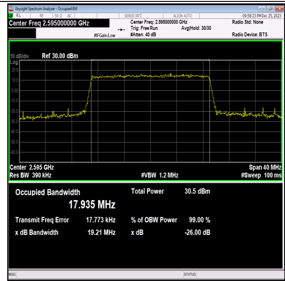
41(2535-2655)-20MHz-16QAM-40640-100RB#0-PASS
