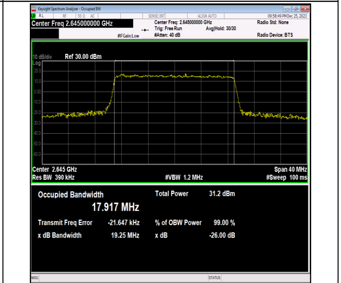
41(2535-2655)-20MHz-QPSK-41140-100RB#0-PASS
