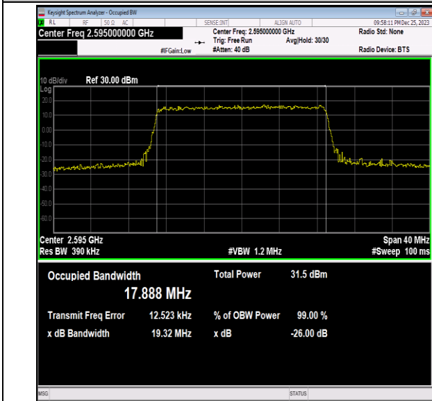
41(2535-2655)-20MHz-QPSK-40640-100RB#0-PASS
