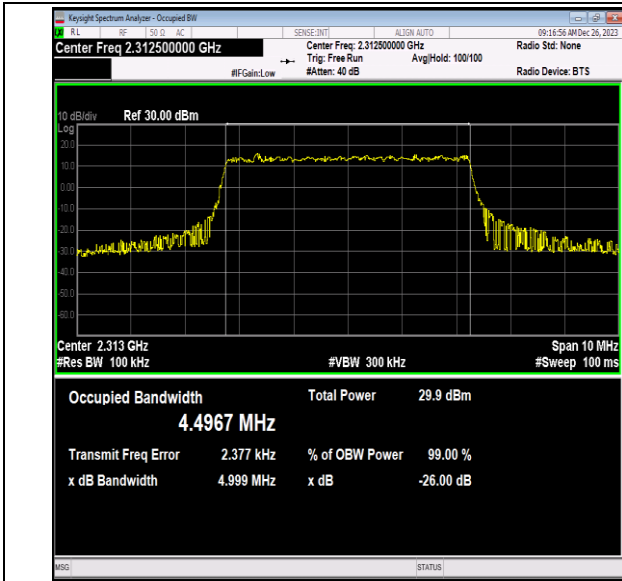
40(2305-2315)-5MHz-QPSK-38775-25RB#0-PASS
