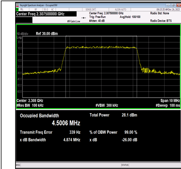
40(2305-2315)-5MHz-64QAM-38725-25RB#0-PASS
