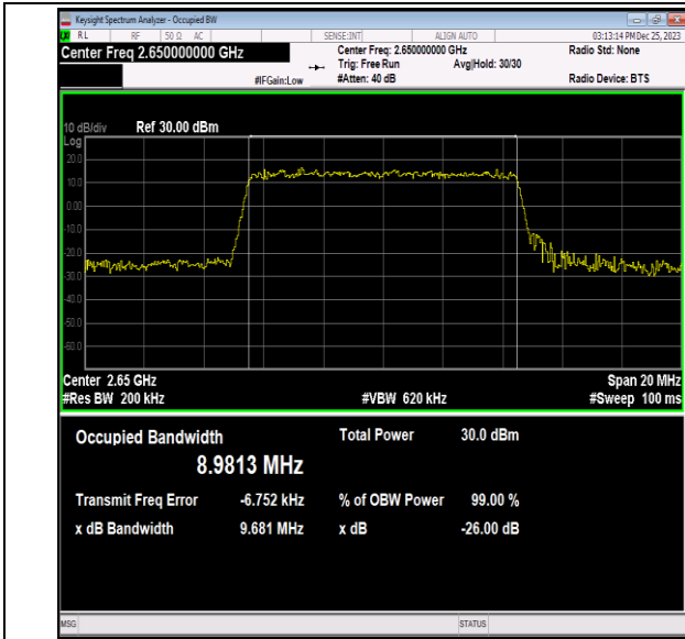
41(2535-2655)-10MHz-16QAM-41190-50RB#0-PASS
