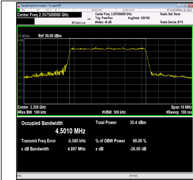
40(2350-2360)-5MHz-QPSK-39225-25RB#0-PASS
