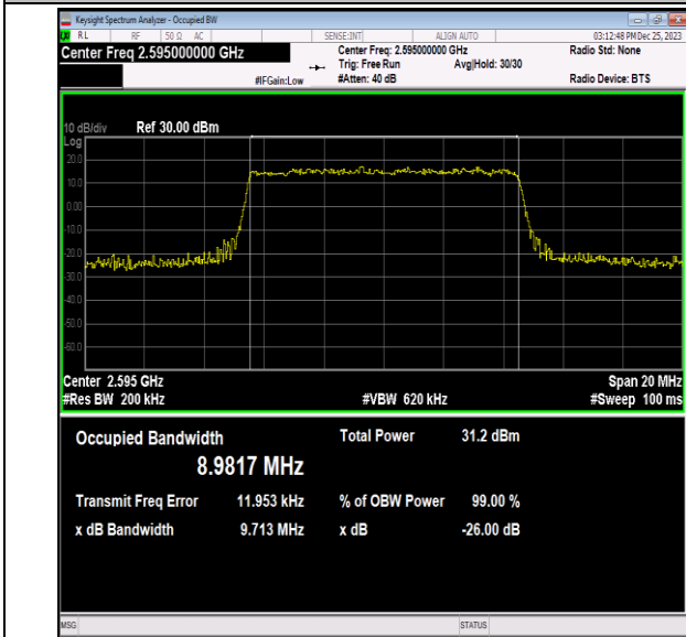
41(2535-2655)-10MHz-64QAM-40640-50RB#0-PASS
