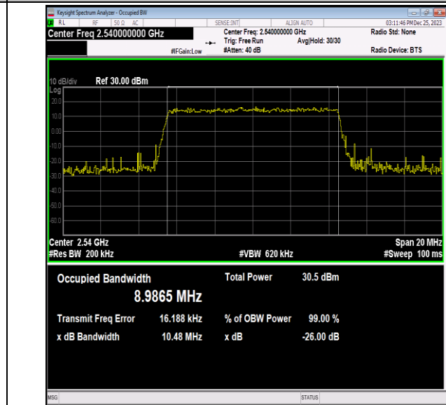
41(2535-2655)-10MHz-QPSK-40090-50RB#0-PASS
