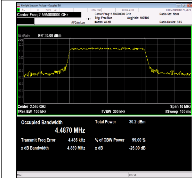
41(2535-2655)-5MHz-16QAM-40640-25RB#0-PASS
