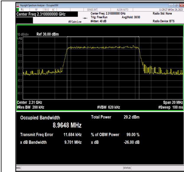
40(2305-2315)-10MHz-16QAM-38750-50RB#0-PASS
