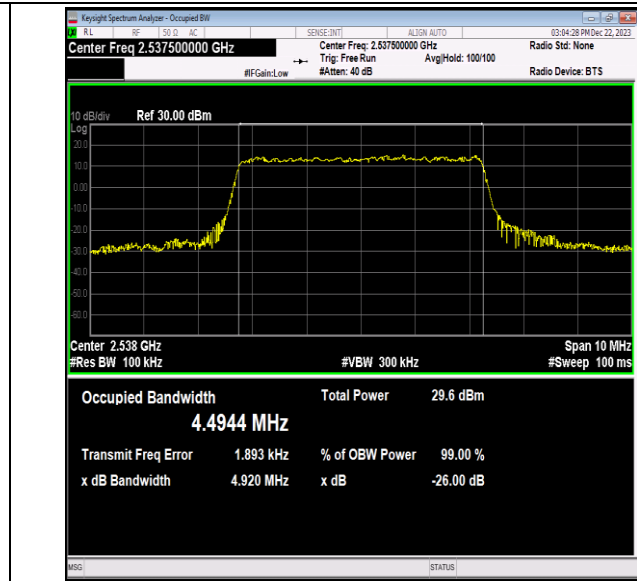
41(2535-2655)-5MHz-16QAM-40065-25RB#0-PASS
