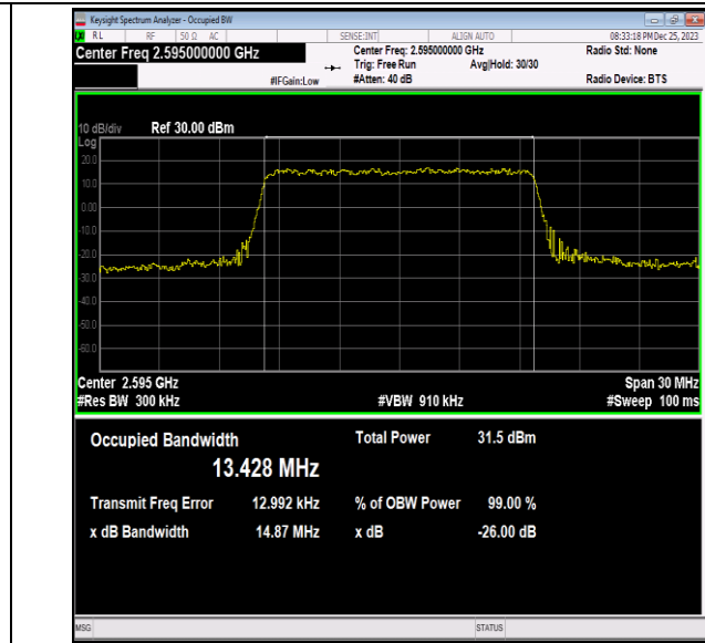
41(2535-2655)-15MHz-QPSK-40640-75RB#0-PASS
