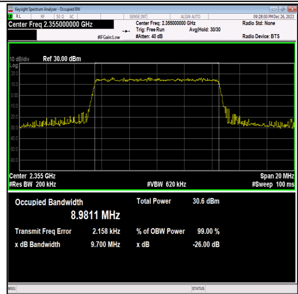
40(2350-2360)-10MHz-QPSK-39200-50RB#0-PASS
