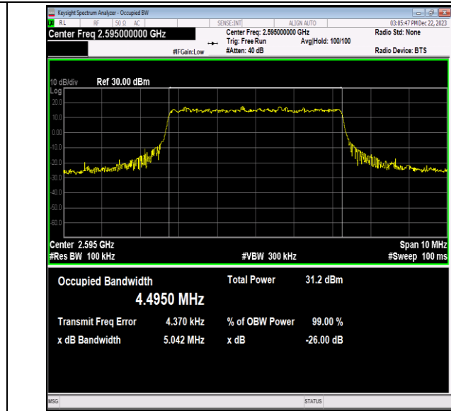
41(2535-2655)-5MHz-64QAM-40640-25RB#0-PASS
