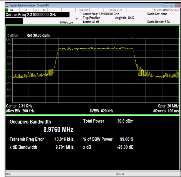
40(2305-2315)-10MHz-QPSK-38750-50RB#0-PASS
