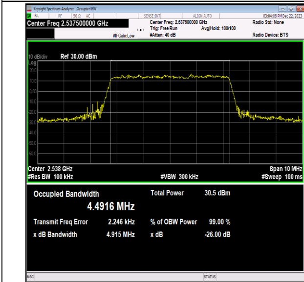
41(2535-2655)-5MHz-QPSK-40065-25RB#0-PASS
