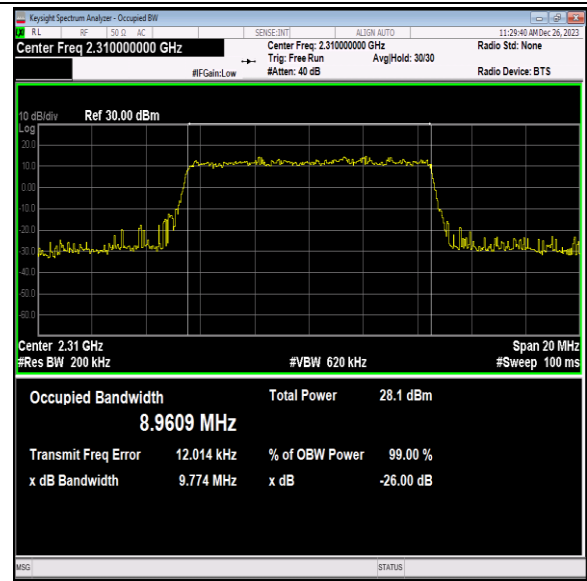
40(2305-2315)-10MHz-64QAM-38750-50RB#0-PASS
