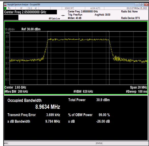
41(2535-2655)-10MHz-64QAM-41190-50RB#0-PASS
