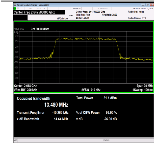
41(2535-2655)-15MHz-QPSK-41165-75RB#0-PASS
