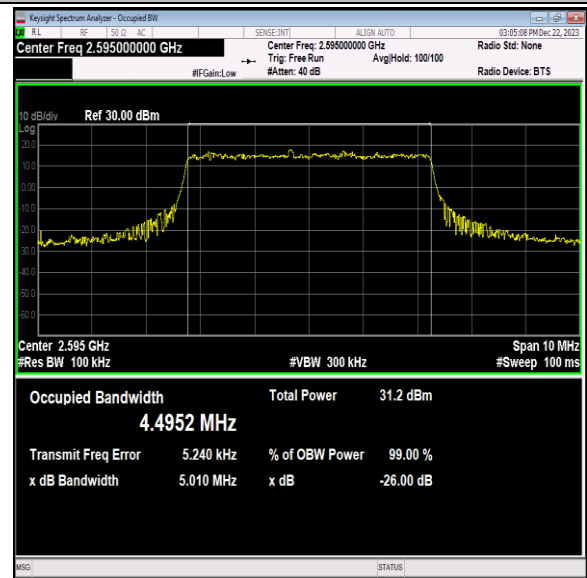
41(2535-2655)-5MHz-QPSK-40640-25RB#0-PASS
