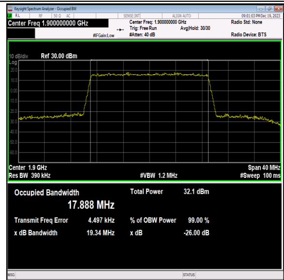
Band2-20MHz-QPSK-19100-100RB#0-PASS
