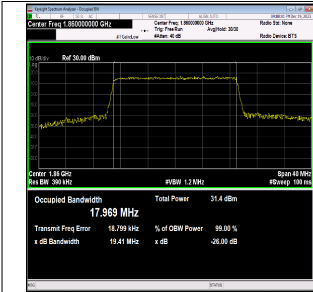
Band2-20MHz-16QAM-18700-100RB#0-PASS
