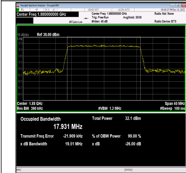
Band2-20MHz-QPSK-18900-100RB#0-PASS
