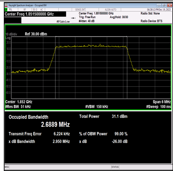
Band2-3MHz-QPSK-18615-15RB#0-PASS
