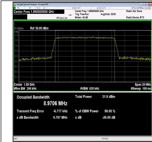
Band2-10MHz-QPSK-18900-50RB#0-PASS
