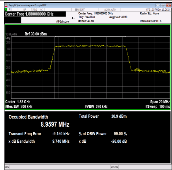
Band2-10MHz-16QAM-18900-50RB#0-PASS
