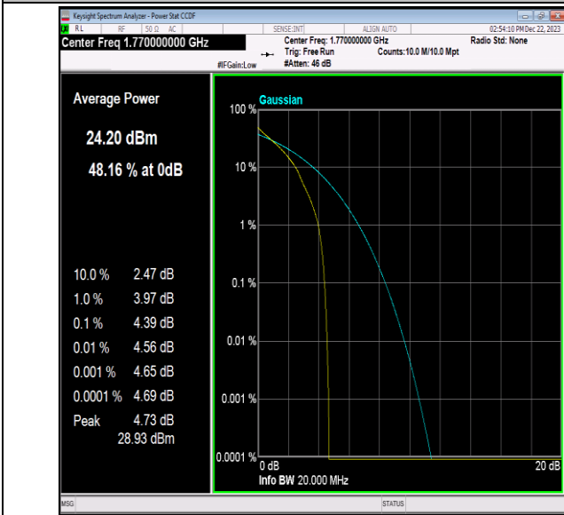
Band66-20MHz-QPSK-132572-1RB#0-PASS
