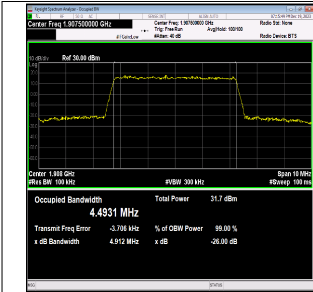
Band2-5MHz-QPSK-19075-25RB#0-PASS
