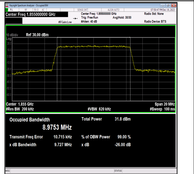
Band2-10MHz-QPSK-18650-50RB#0-PASS
