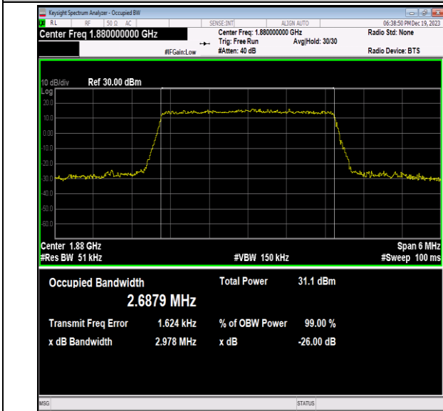
Band2-3MHz-QPSK-18900-15RB#0-PASS
