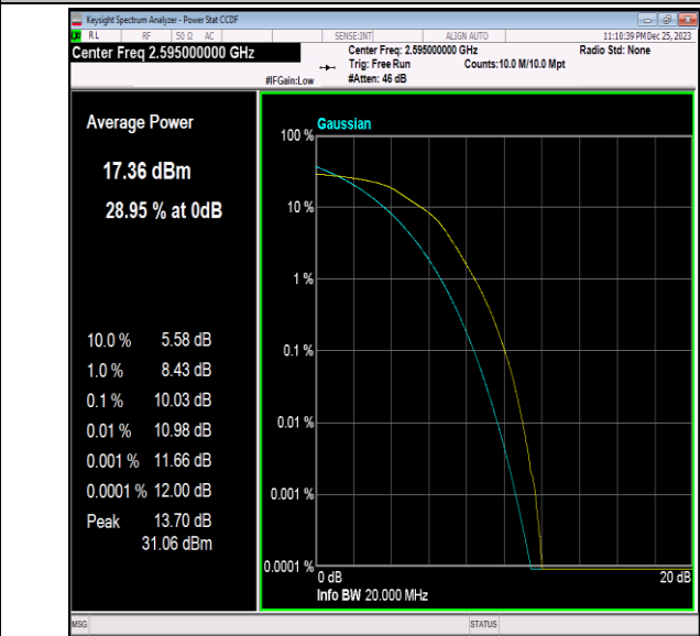
41(2535-2655)-20MHz-16QAM-40640-100RB#0-PASS
