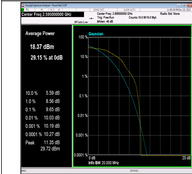
41(2535-2655)-20MHz-16QAM-40640-1RB#0-PASS
