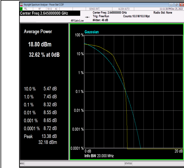
41(2535-2655)-20MHz-16QAM-41140-1RB#0-PASS
