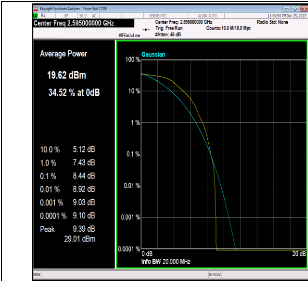
41(2535-2655)-20MHz-64QAM-40640-1RB#0-PASS
