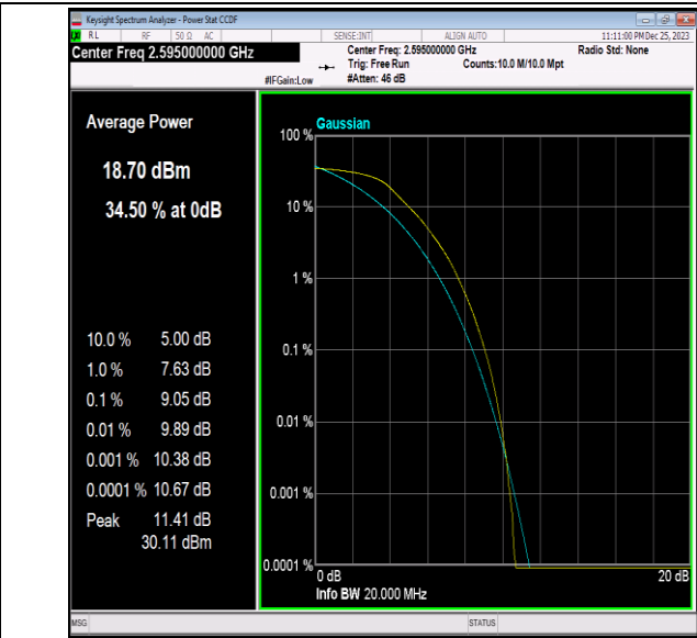
41(2535-2655)-20MHz-64QAM-40640-100RB#0-PASS
