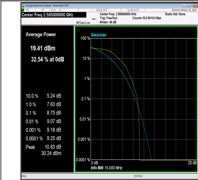
41(2535-2655)-15MHz-QPSK-40640-1RB#0-PASS
