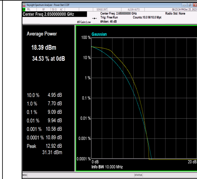
41(2535-2655)-10MHz-QPSK-41190-50RB#0-PASS
