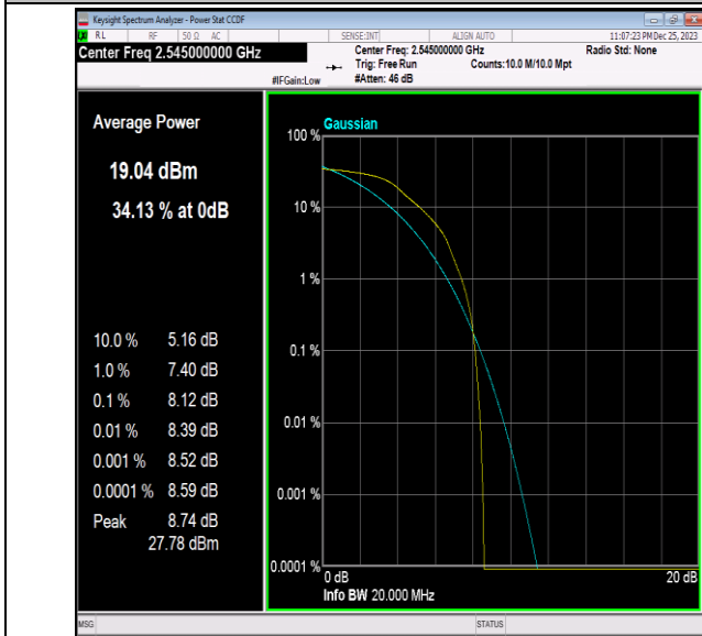
41(2535-2655)-20MHz-QPSK-40140-1RB#0-PASS
