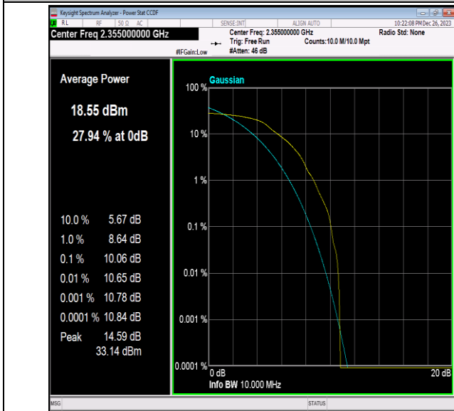
40(2350-2360)-10MHz-QPSK-39200-1RB#0-PASS
