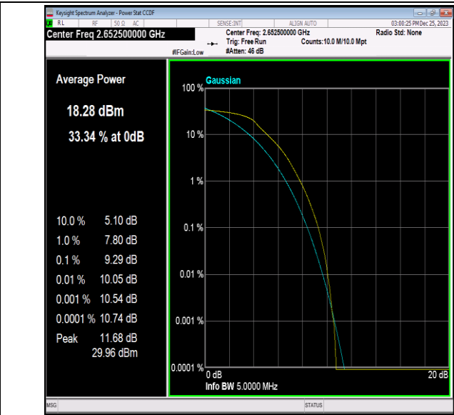
41(2535-2655)-5MHz-QPSK-41215-25RB#0-PASS
