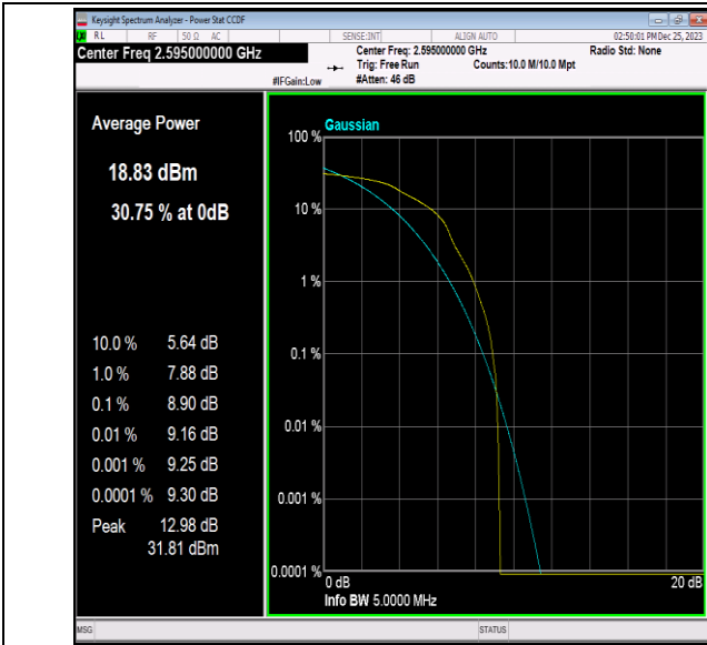
41(2535-2655)-5MHz-16QAM-40640-1RB#0-PASS
