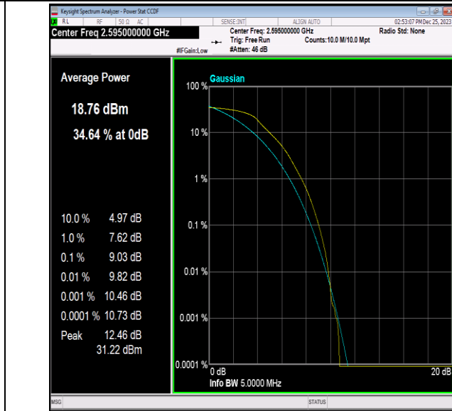
41(2535-2655)-5MHz-QPSK-40640-25RB#0-PASS
