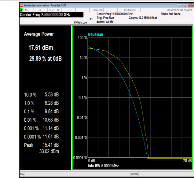
41(2535-2655)-5MHz-16QAM-40640-25RB#0-PASS
