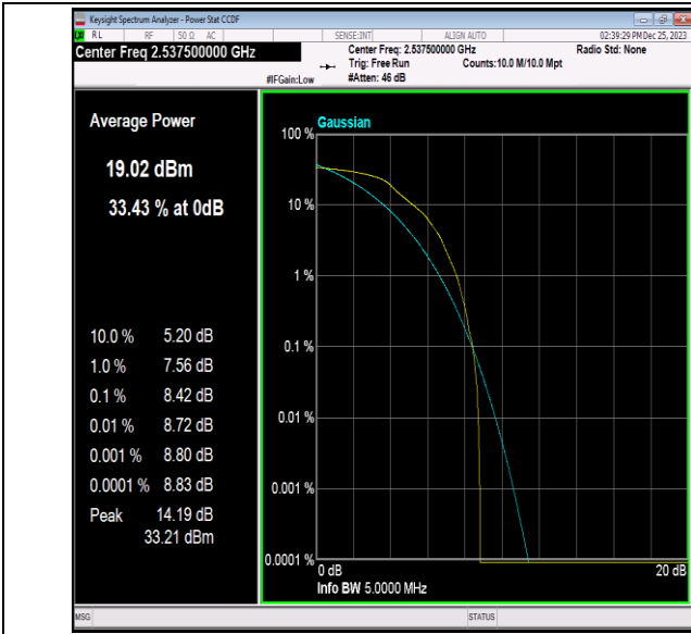
41(2535-2655)-5MHz-QPSK-40065-1RB#0-PASS
