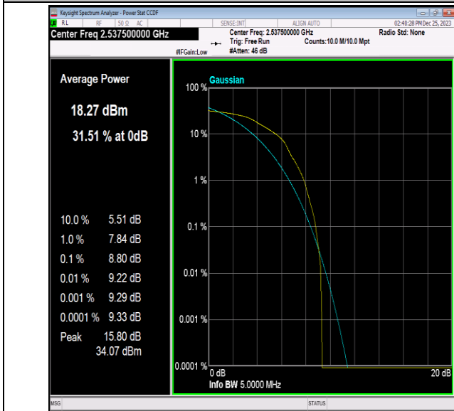
41(2535-2655)-5MHz-16QAM-40065-1RB#0-PASS
