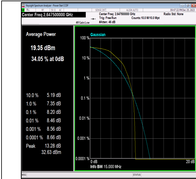
41(2535-2655)-15MHz-QPSK-41165-1RB#0-PASS
