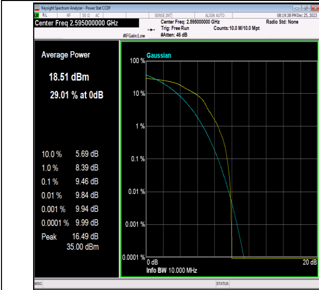
41(2535-2655)-10MHz-16QAM-40640-1RB#0-PASS
