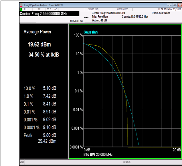
41(2535-2655)-20MHz-QPSK-40640-1RB#0-PASS
