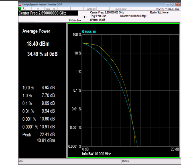
41(2535-2655)-10MHz-64QAM-41190-50RB#0-PASS
