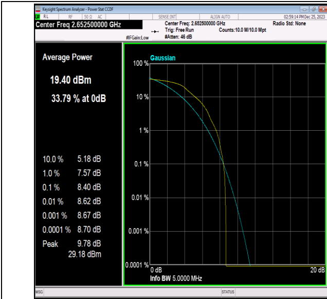
41(2535-2655)-5MHz-64QAM-41215-1RB#0-PASS
