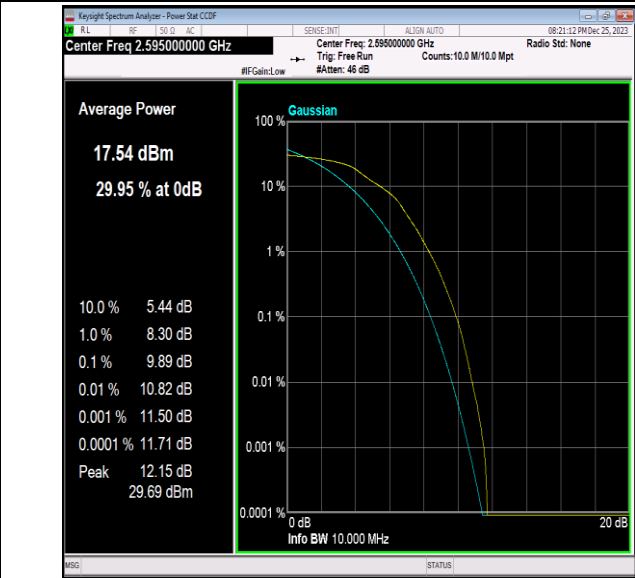
41(2535-2655)-10MHz-16QAM-40640-50RB#0-PASS
