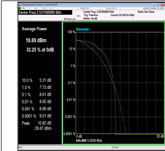
41(2535-2655)-5MHz-64QAM-40065-1RB#0-PASS
