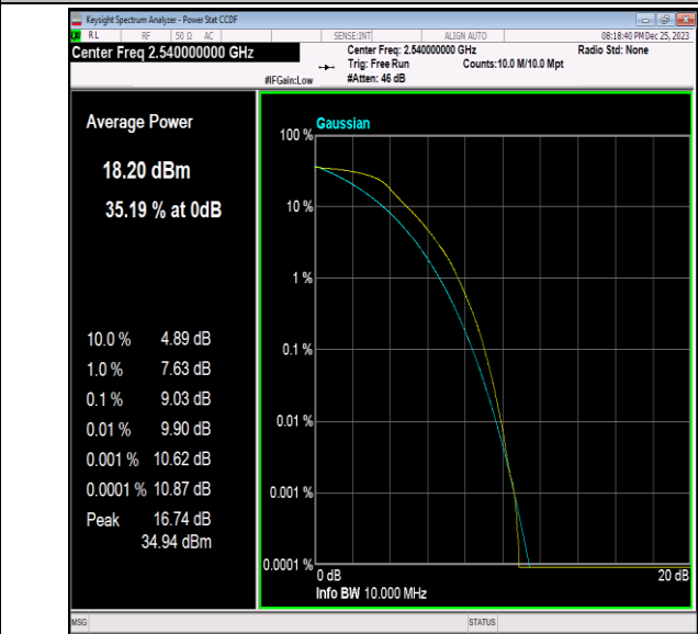
41(2535-2655)-10MHz-64QAM-40090-50RB#0-PASS
