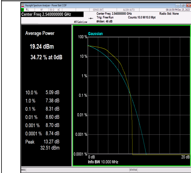
41(2535-2655)-10MHz-64QAM-40090-1RB#0-PASS
