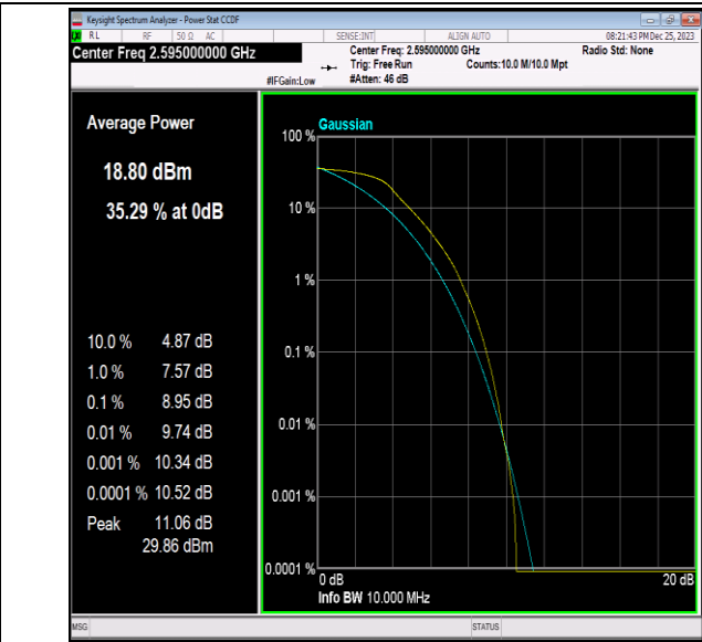
41(2535-2655)-10MHz-64QAM-40640-50RB#0-PASS
