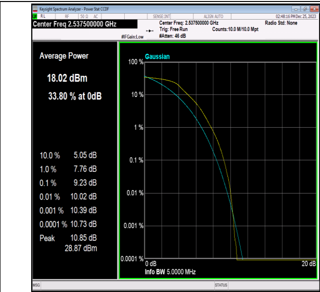
41(2535-2655)-5MHz-64QAM-40065-25RB#0-PASS
