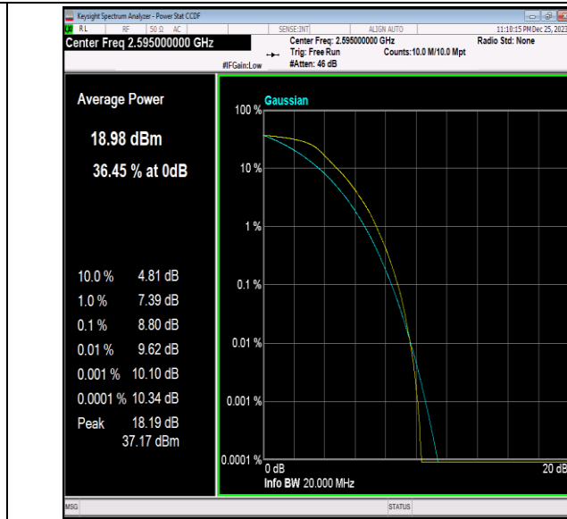
41(2535-2655)-20MHz-QPSK-40640-100RB#0-PASS
