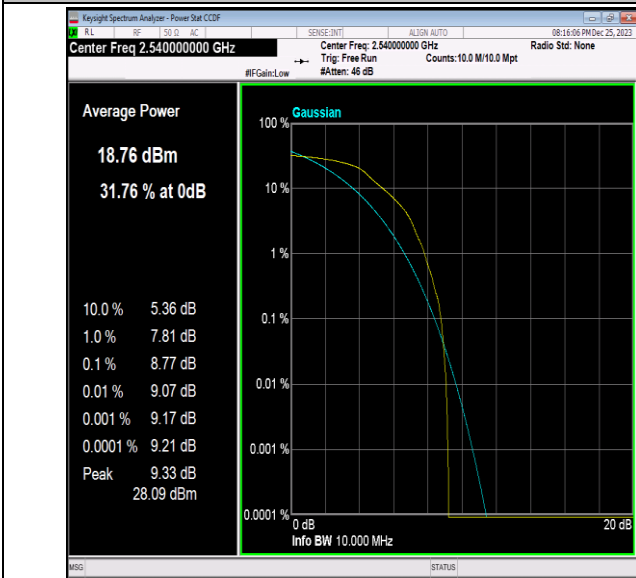
41(2535-2655)-10MHz-QPSK-40090-1RB#0-PASS
