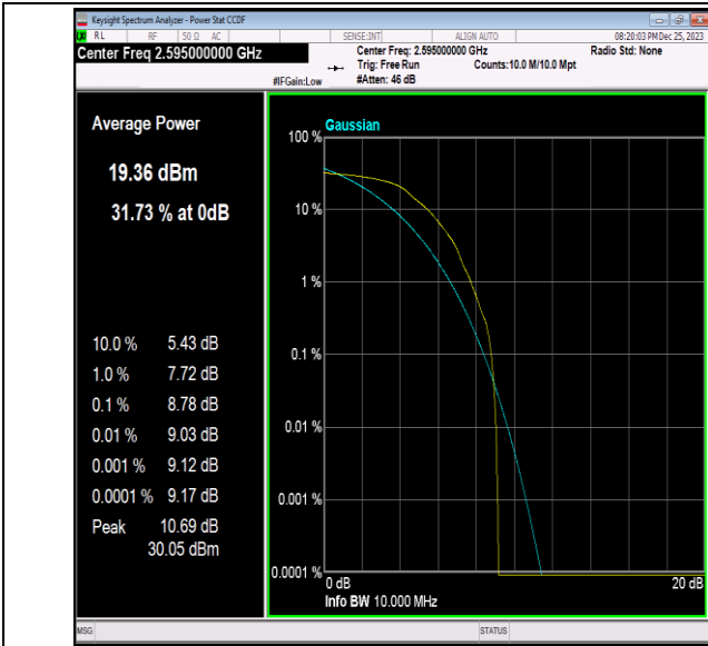
41(2535-2655)-10MHz-64QAM-40640-1RB#0-PASS
