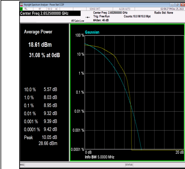
41(2535-2655)-5MHz-16QAM-41215-1RB#0-PASS
