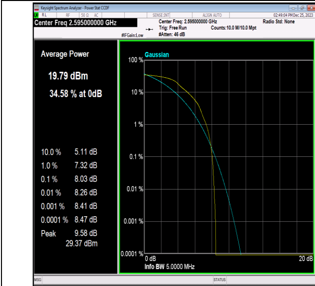
41(2535-2655)-5MHz-QPSK-40640-1RB#0-PASS
