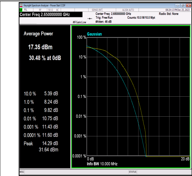
41(2535-2655)-10MHz-16QAM-41190-50RB#0-PASS
