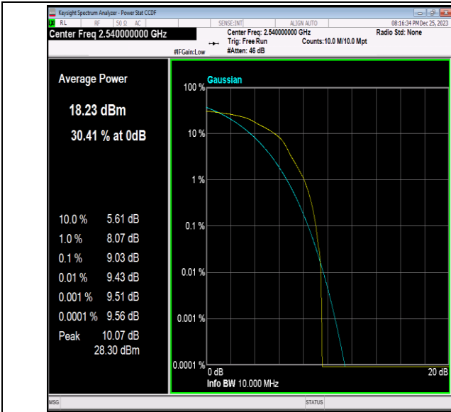
41(2535-2655)-10MHz-16QAM-40090-1RB#0-PASS
