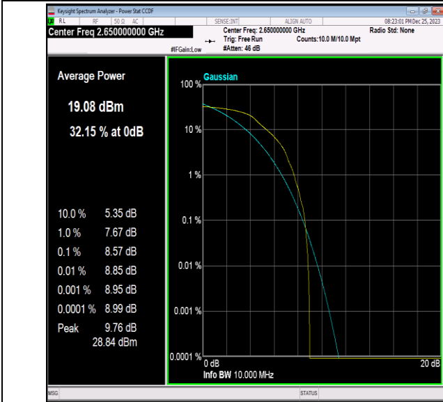
41(2535-2655)-10MHz-64QAM-41190-1RB#0-PASS
