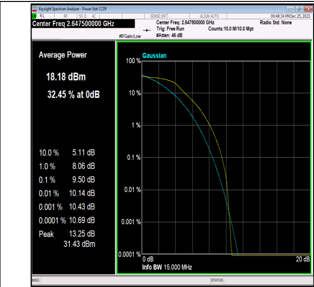
41(2535-2655)-15MHz-QPSK-41165-75RB#0-PASS
