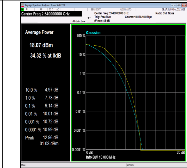
41(2535-2655)-10MHz-QPSK-40090-50RB#0-PASS
