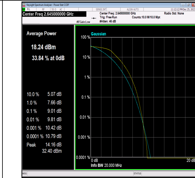
41(2535-2655)-20MHz-QPSK-41140-100RB#0-PASS
