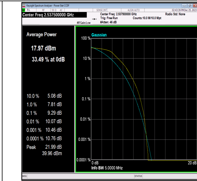
41(2535-2655)-5MHz-QPSK-40065-25RB#0-PASS
