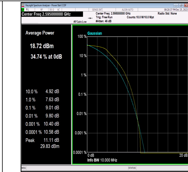
41(2535-2655)-10MHz-QPSK-40640-50RB#0-PASS
