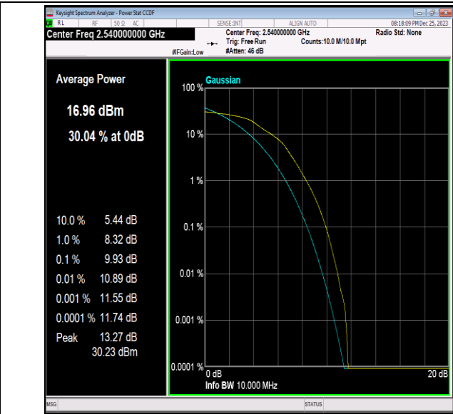
41(2535-2655)-10MHz-16QAM-40090-50RB#0-PASS
