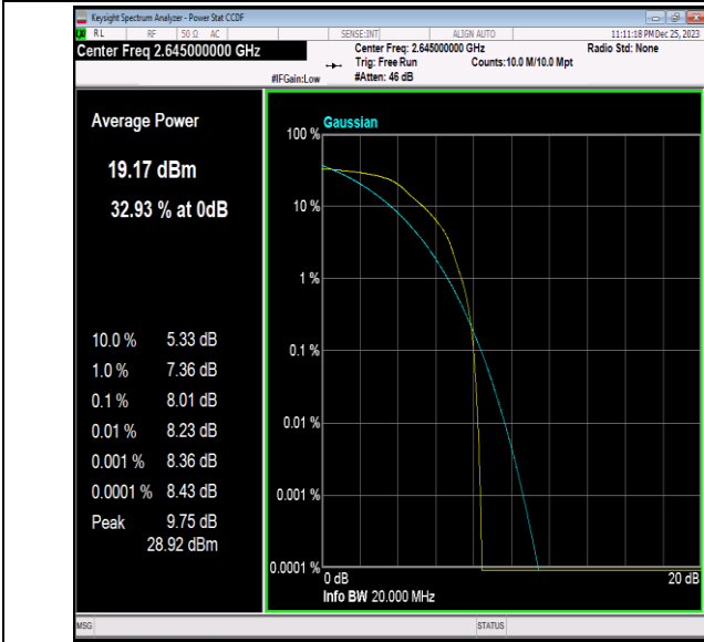
41(2535-2655)-20MHz-QPSK-41140-1RB#0-PASS
