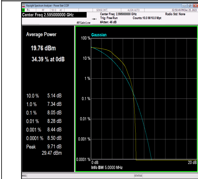
41(2535-2655)-5MHz-64QAM-40640-1RB#0-PASS
