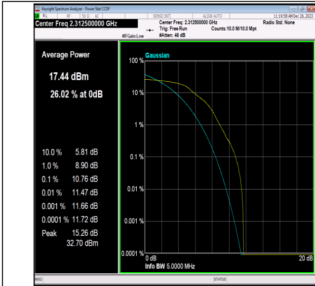
40(2305-2315)-5MHz-QPSK-38775-1RB#0-PASS
