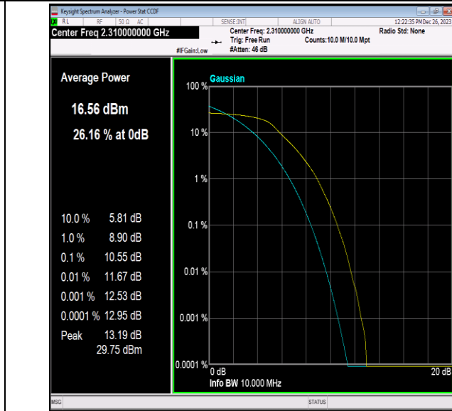
40(2305-2315)-10MHz-QPSK-38750-50RB#0-PASS
