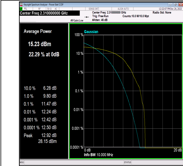
40(2305-2315)-10MHz-64QAM-38750-1RB#0-PASS
