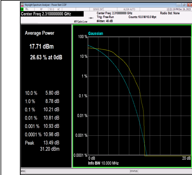
40(2305-2315)-10MHz-QPSK-38750-1RB#0-PASS
