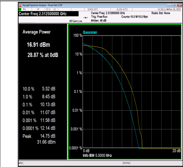
40(2305-2315)-5MHz-QPSK-38775-25RB#0-PASS
