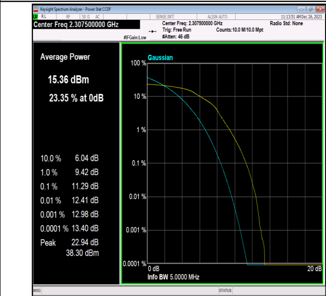
40(2305-2315)-5MHz-16QAM-38725-25RB#0-PASS
