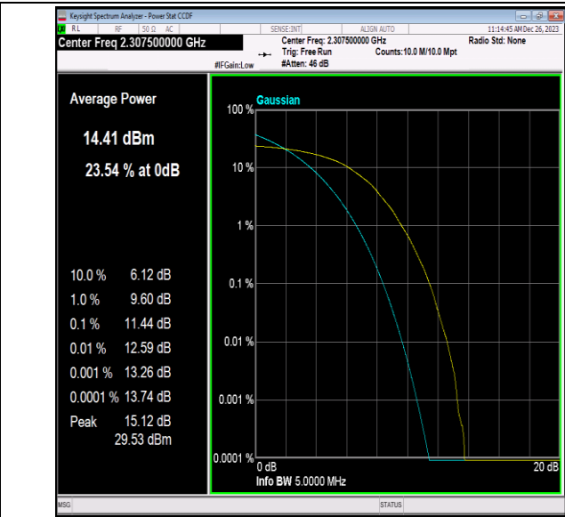
40(2305-2315)-5MHz-64QAM-38725-25RB#0-PASS
