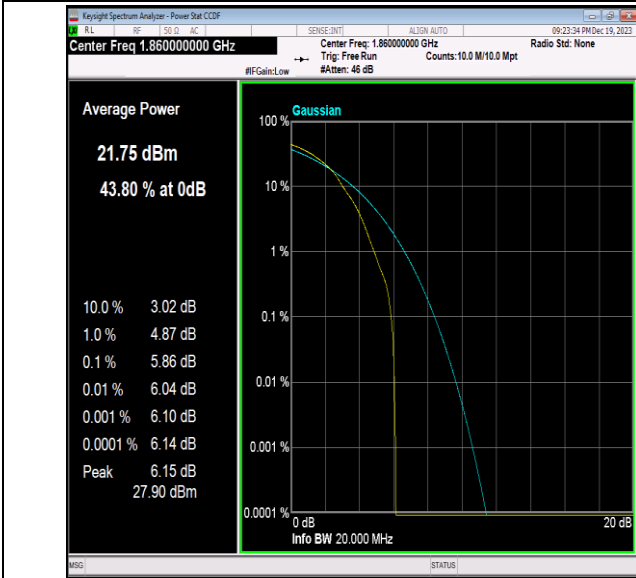
Band2-20MHz-64QAM-18700-1RB#0-PASS
