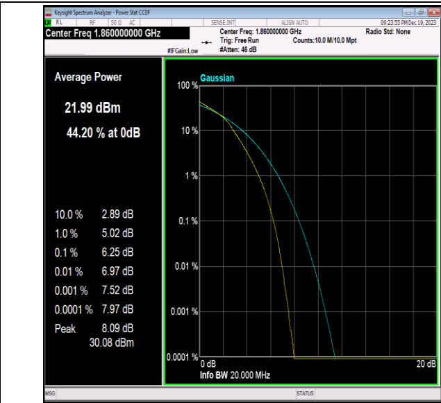
Band2-20MHz-16QAM-18700-100RB#0-PASS
