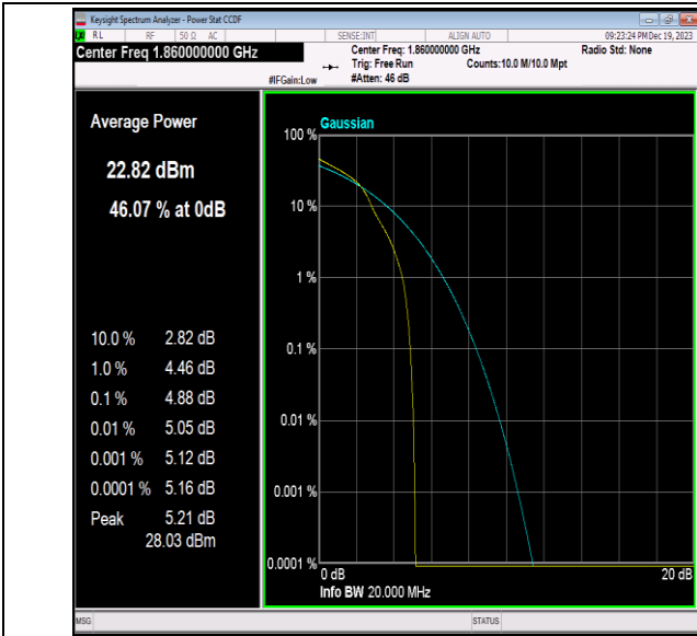
Band2-20MHz-16QAM-18700-1RB#0-PASS
