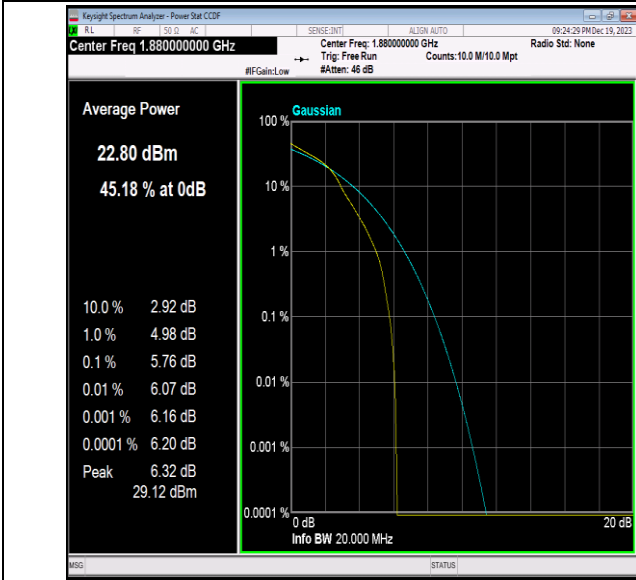
Band2-20MHz-16QAM-18900-1RB#0-PASS
