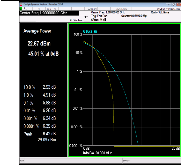
Band2-20MHz-16QAM-19100-1RB#0-PASS
