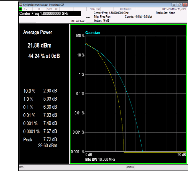
Band2-10MHz-16QAM-18900-50RB#0-PASS
