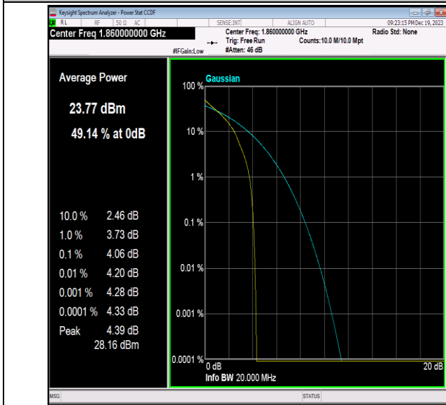
Band2-20MHz-QPSK-18700-1RB#0-PASS
