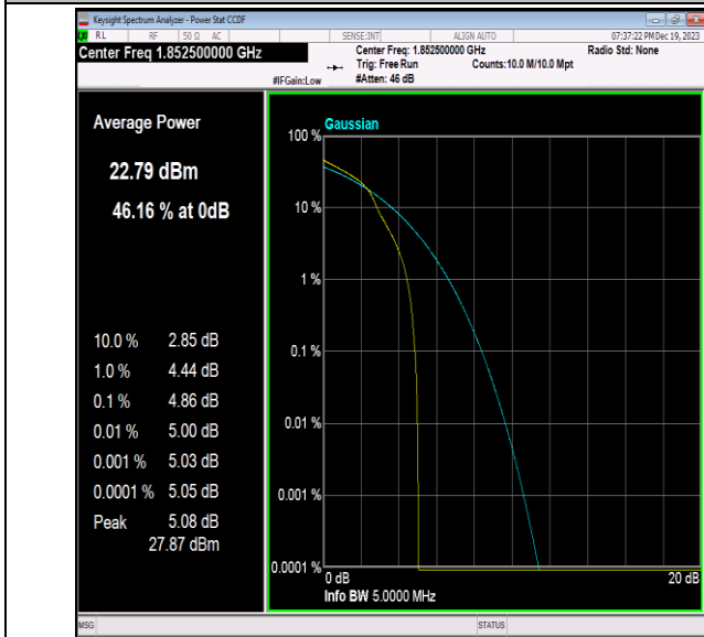
Band2-5MHz-16QAM-18625-1RB#0-PASS
