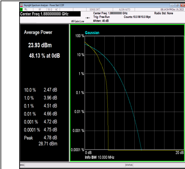
Band2-10MHz-QPSK-18900-1RB#0-PASS
