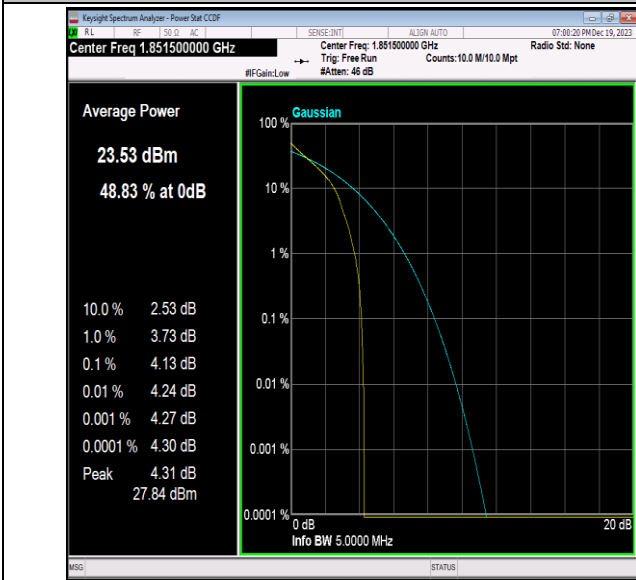
Band2-3MHz-QPSK-18615-1RB#0-PASS
