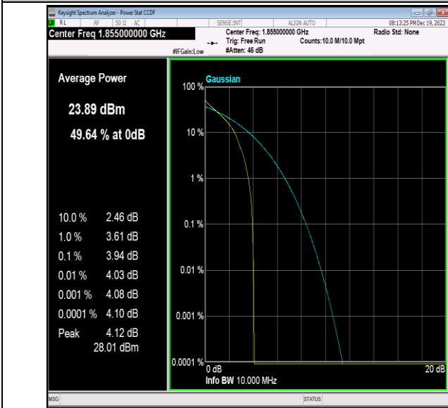
Band2-10MHz-QPSK-18650-1RB#0-PASS
