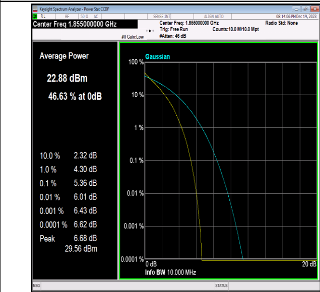
Band2-10MHz-QPSK-18650-50RB#0-PASS
