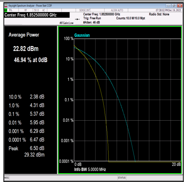
Band2-5MHz-QPSK-18625-25RB#0-PASS
