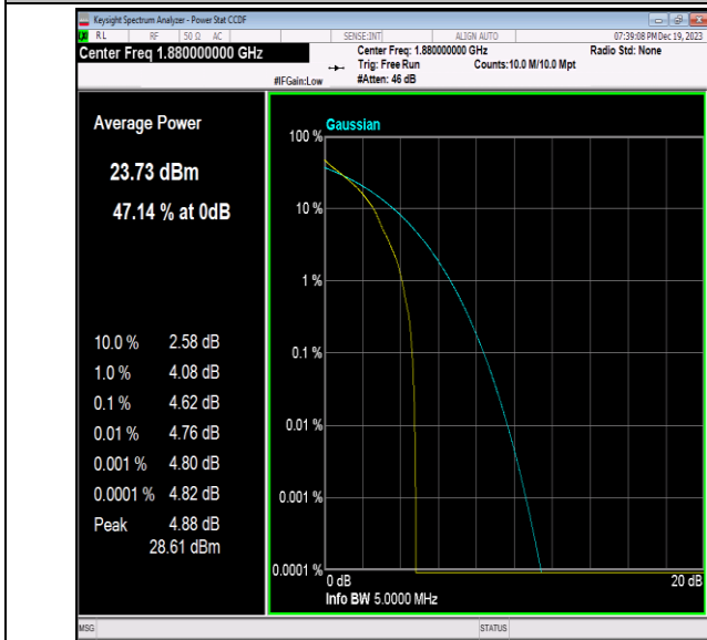
Band2-5MHz-QPSK-18900-1RB#0-PASS
