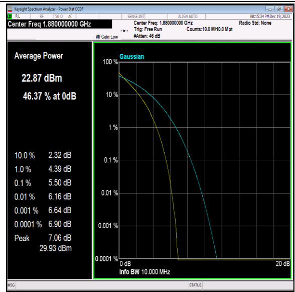
Band2-10MHz-QPSK-18900-50RB#0-PASS
