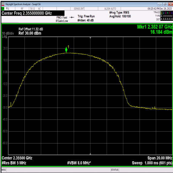
40(2350-2360)-10MHz-QPSK-39200-25RB#0-PASS
