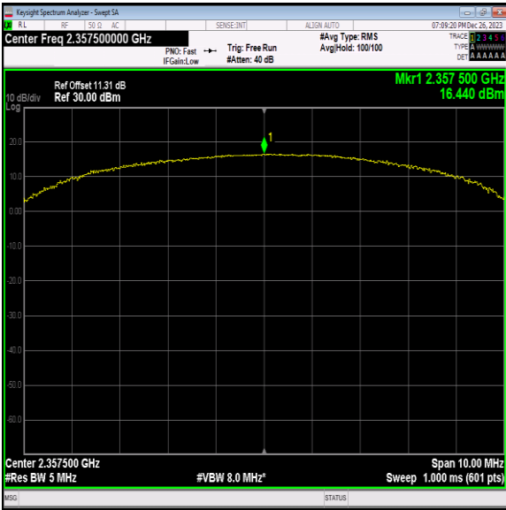
40(2350-2360)-5MHz-QPSK-39225-25RB#0-PASS
