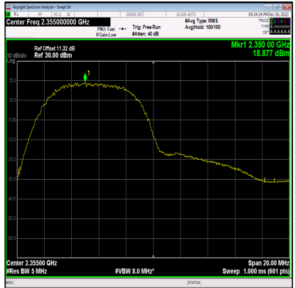
40(2350-2360)-10MHz-QPSK-39200-1RB#0-PASS
