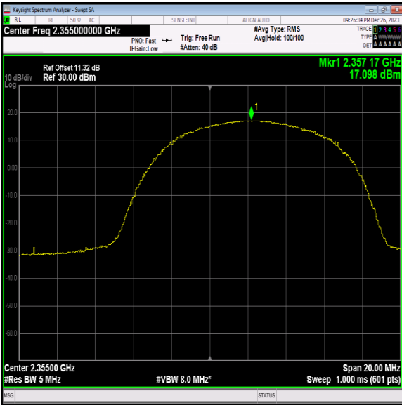
40(2350-2360)-10MHz-QPSK-39200-25RB#25-PASS
