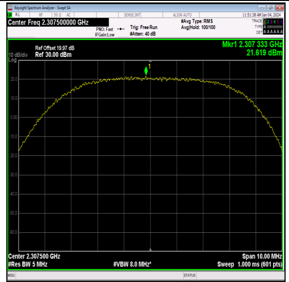
40(2305-2315)-5MHz-QPSK-38725-1RB#12-PASS
