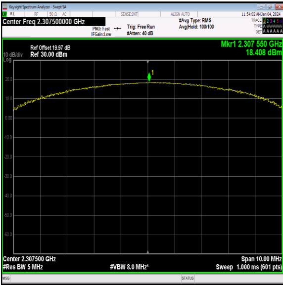
40(2305-2315)-5MHz-64QAM-38725-25RB#0-PASS
