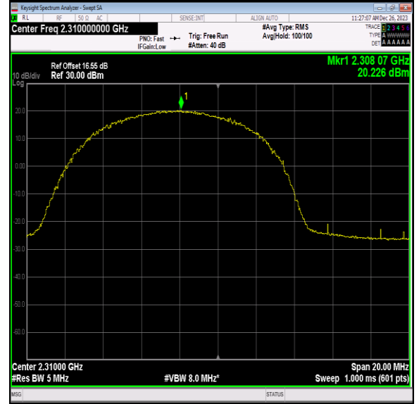
40(2305-2315)-10MHz-16QAM-38750-25RB#0-PASS
