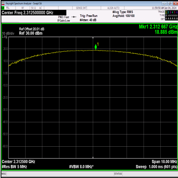
40(2305-2315)-5MHz-QPSK-38775-25RB#0-PASS
