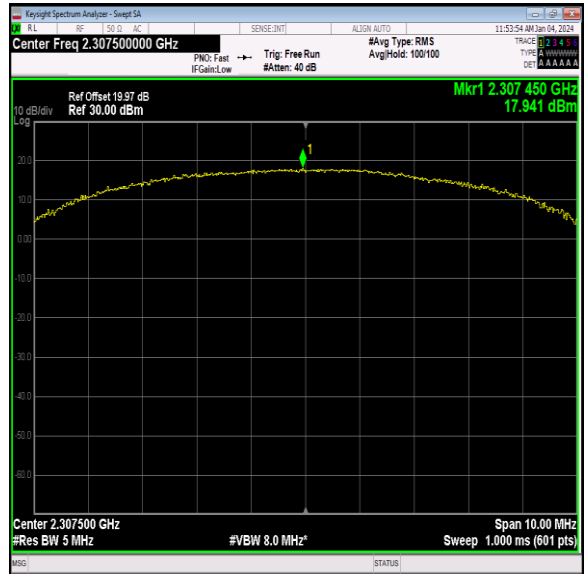
40(2305-2315)-5MHz-16QAM-38725-25RB#0-PASS
