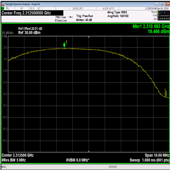
40(2305-2315)-5MHz-QPSK-38775-12RB#6-PASS
