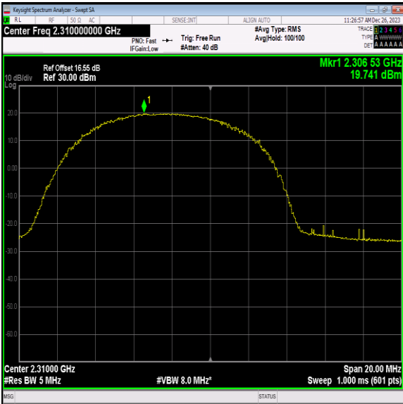
40(2305-2315)-10MHz-QPSK-38750-25RB#0-PASS
