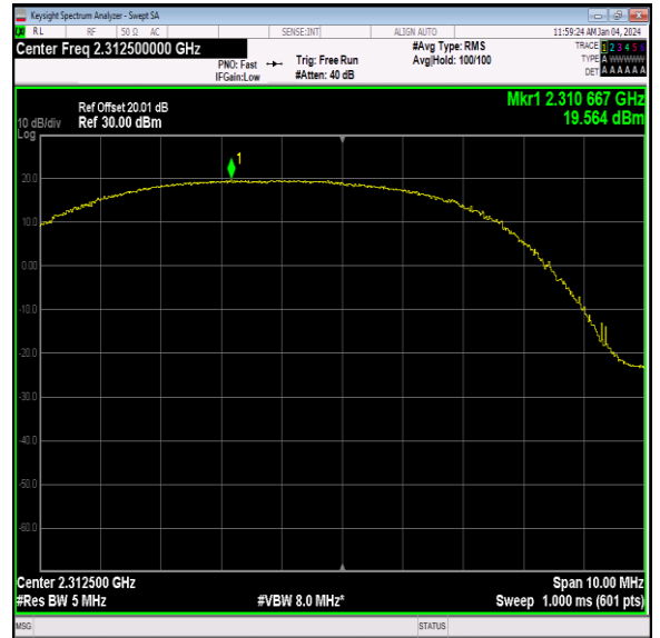
40(2305-2315)-5MHz-QPSK-38775-12RB#11-PASS
