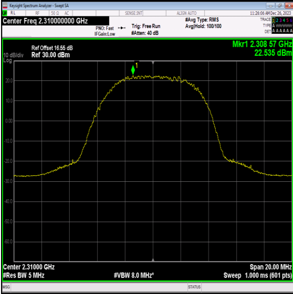
40(2305-2315)-10MHz-QPSK-38750-1RB#24-PASS
