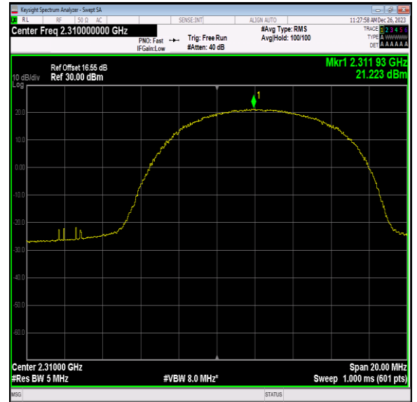
40(2305-2315)-10MHz-16QAM-38750-25RB#25-PASS
