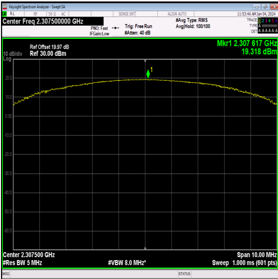
40(2305-2315)-5MHz-QPSK-38725-25RB#0-PASS
