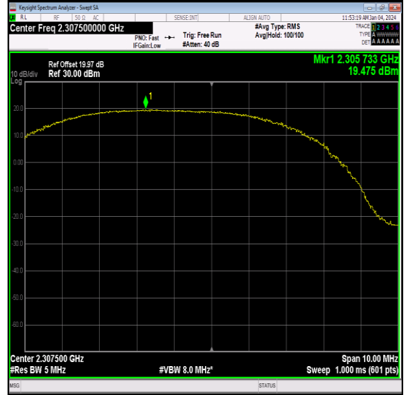
40(2305-2315)-5MHz-QPSK-38725-12RB#11-PASS
