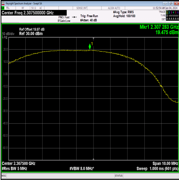
40(2305-2315)-5MHz-QPSK-38725-12RB#6-PASS
