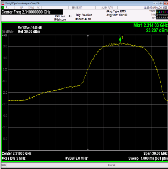
40(2305-2315)-10MHz-16QAM-38750-1RB#49-PASS
