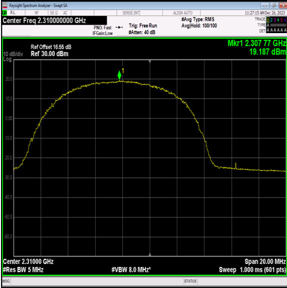
40(2305-2315)-10MHz-64QAM-38750-25RB#0-PASS
