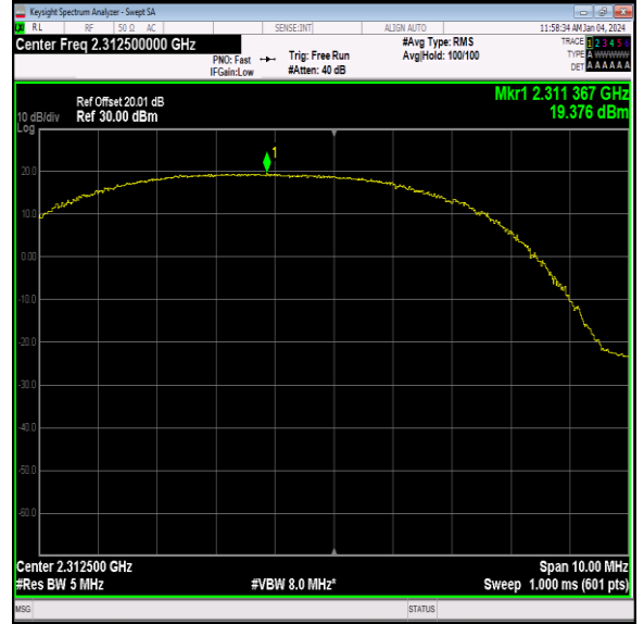
40(2305-2315)-5MHz-QPSK-38775-12RB#0-PASS
