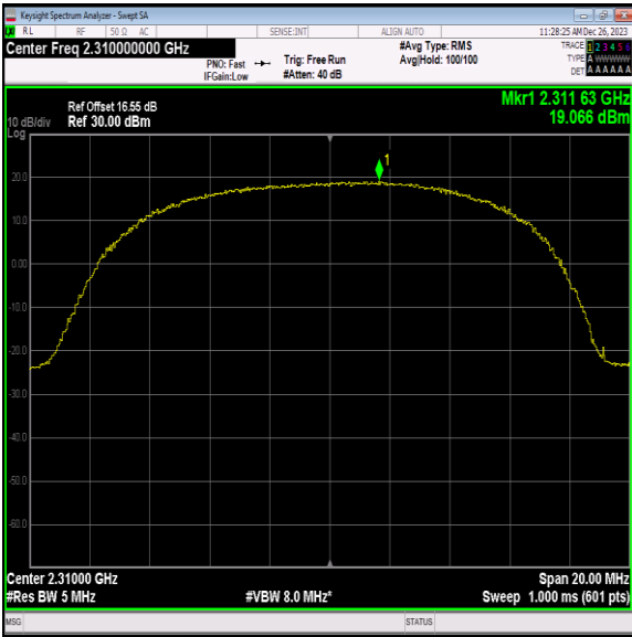
40(2305-2315)-10MHz-16QAM-38750-50RB#0-PASS
