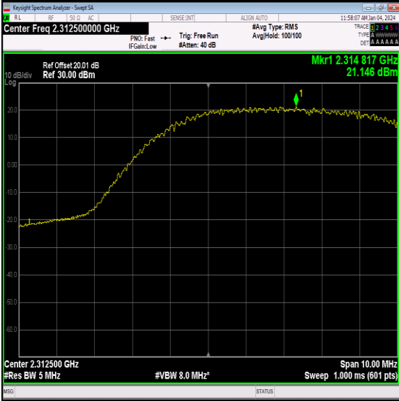
40(2305-2315)-5MHz-QPSK-38775-1RB#24-PASS
