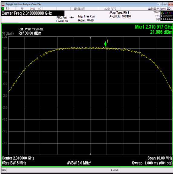
40(2305-2315)-5MHz-QPSK-38750-1RB#12-PASS
