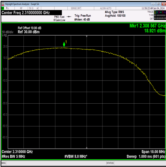
40(2305-2315)-5MHz-QPSK-38750-12RB#11-PASS
