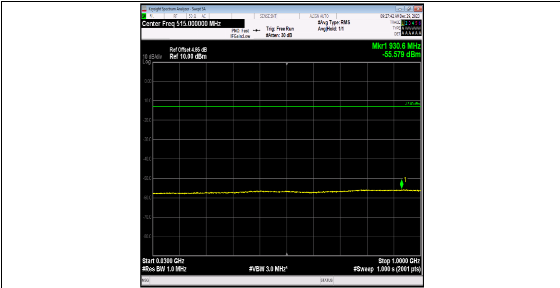
Band4-1513-5-30~1000MHz-PASS
