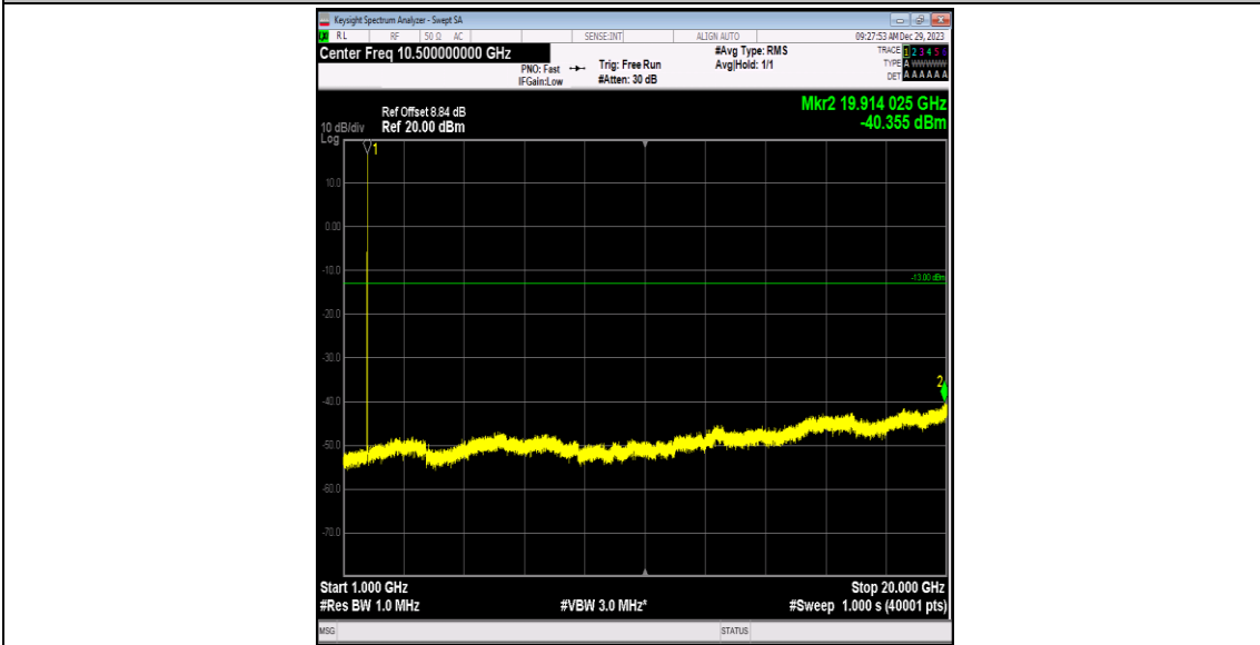
Band4-1513-5-1000~20000MHz-PASS
