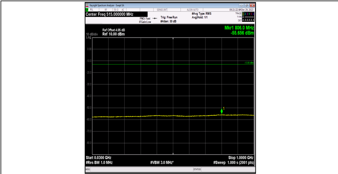
Band4-1513-3-30~1000MHz-PASS
