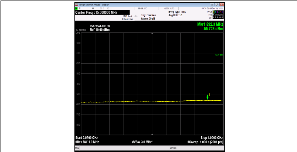
Band4-1413-3-30~1000MHz-PASS
