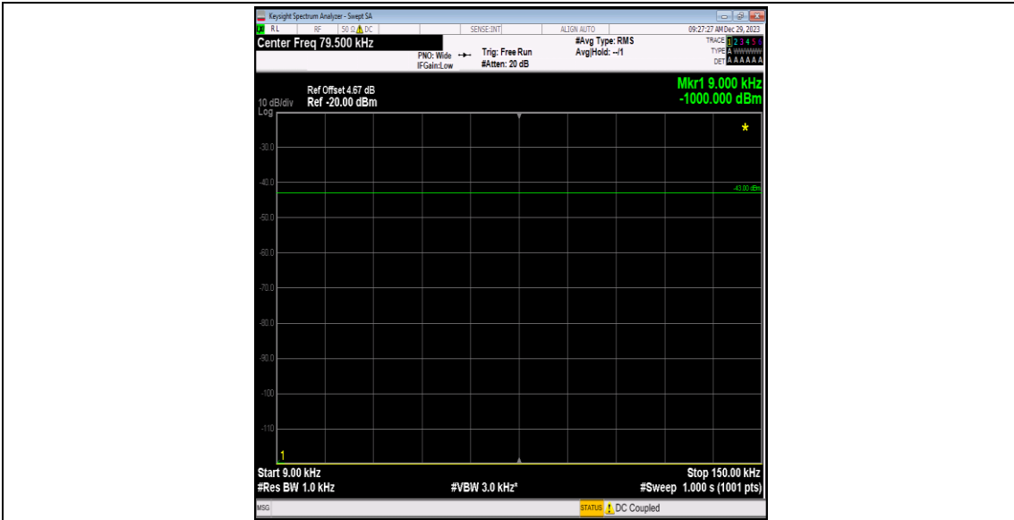
Band4-1513-5-0.009~0.15MHz-PASS
