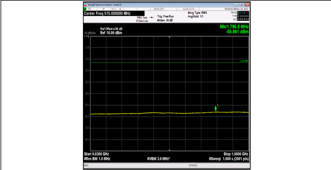
Band4-1312-5-30~1000MHz-PASS
