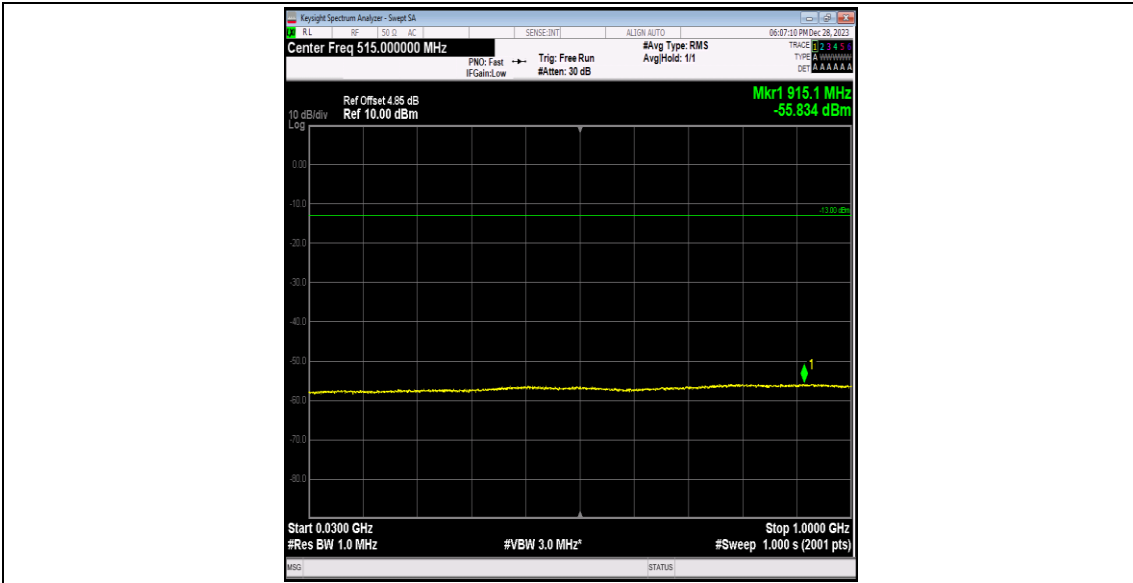
Band2-9538-5-30~1000MHz-PASS
