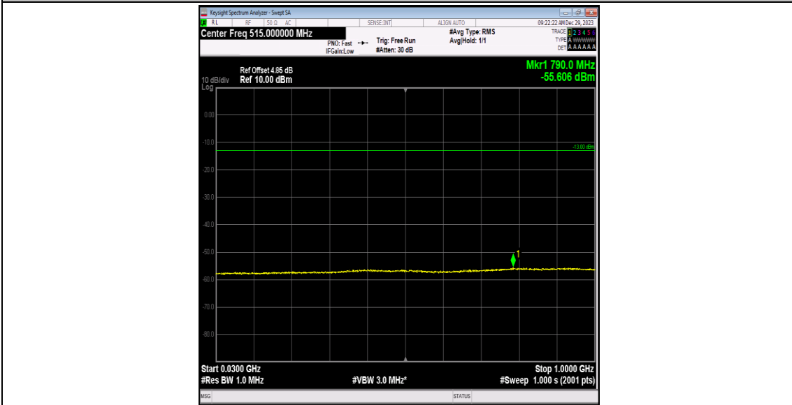
Band4-1312-4-30~1000MHz-PASS
