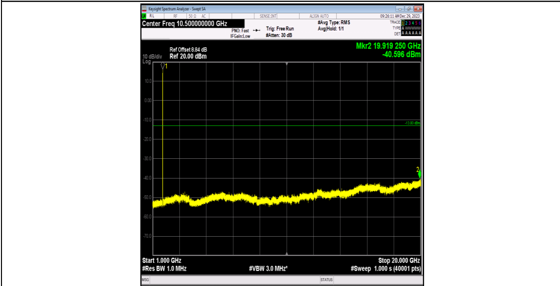
Band4-1312-5-1000~20000MHz-PASS
