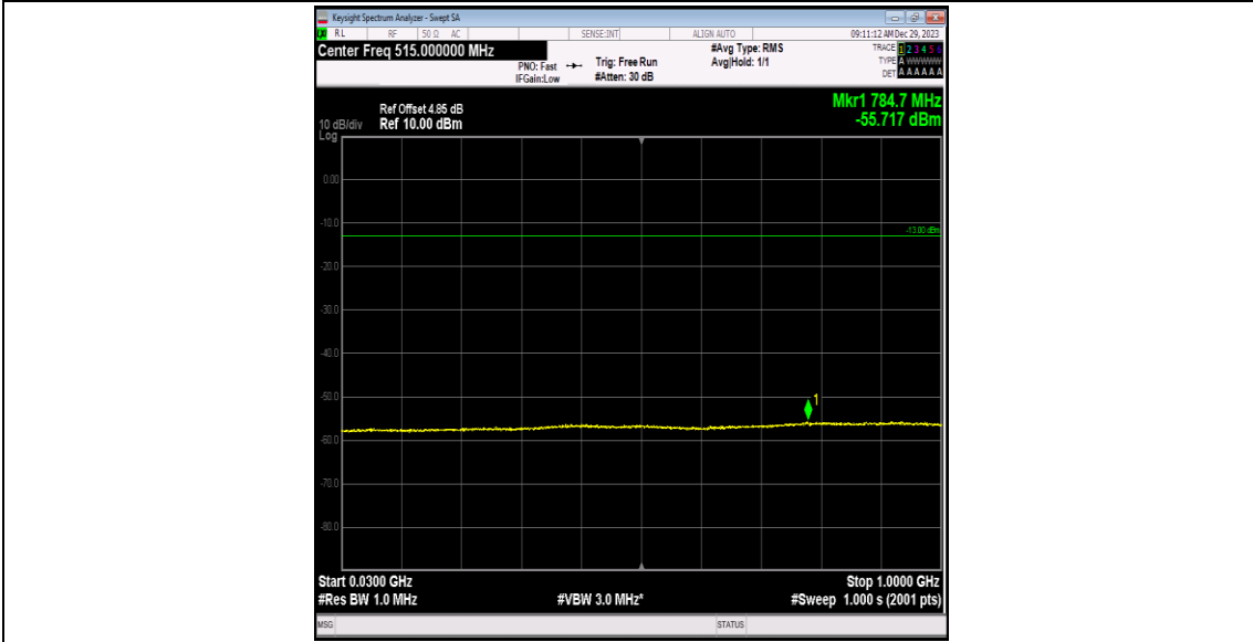
Band4-1312-1-30~1000MHz-PASS
