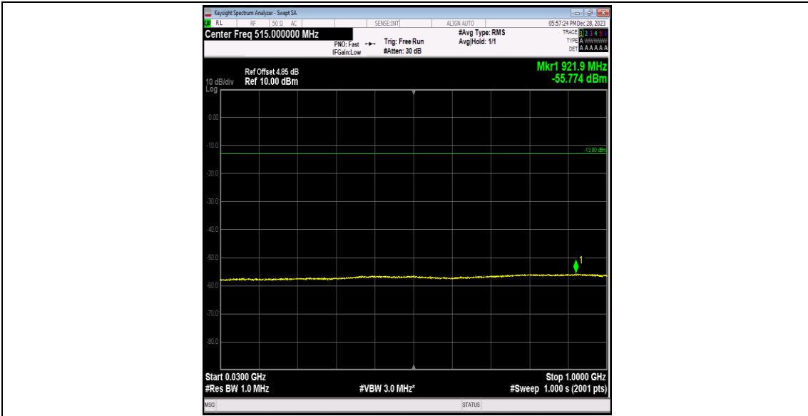
Band2-9538-2-30~1000MHz-PASS
