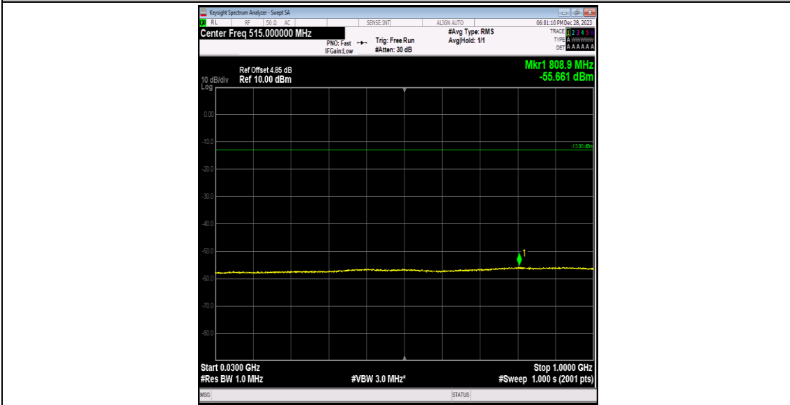
Band2-9538-3-30~1000MHz-PASS
