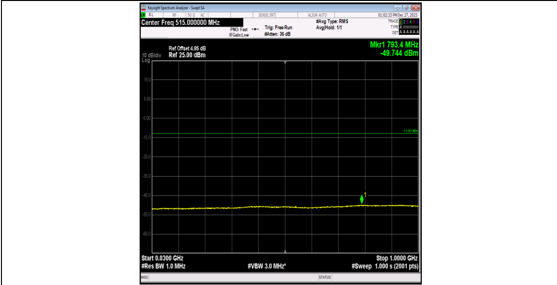
Band4-1312-3-30~1000MHz-PASS
