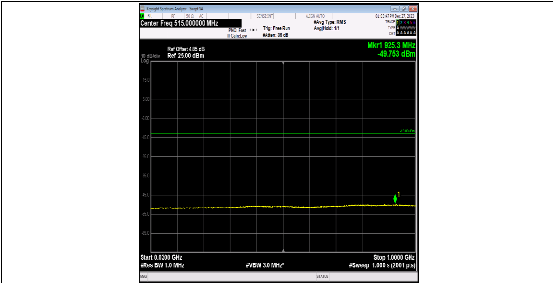
Band4-1513-3-30~1000MHz-PASS
