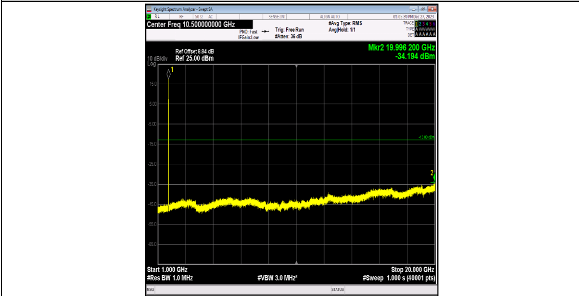
Band4-1413-4-1000~20000MHz-PASS
