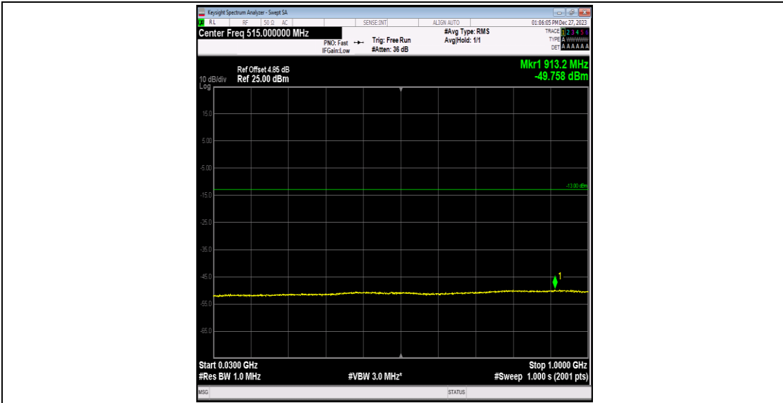
Band4-1513-4-30~1000MHz-PASS
