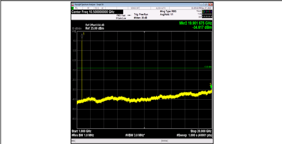
Band4-1312-4-1000~20000MHz-PASS
