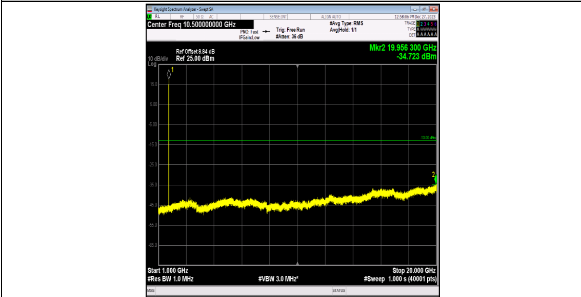
Band4-1312-1-1000~20000MHz-PASS
