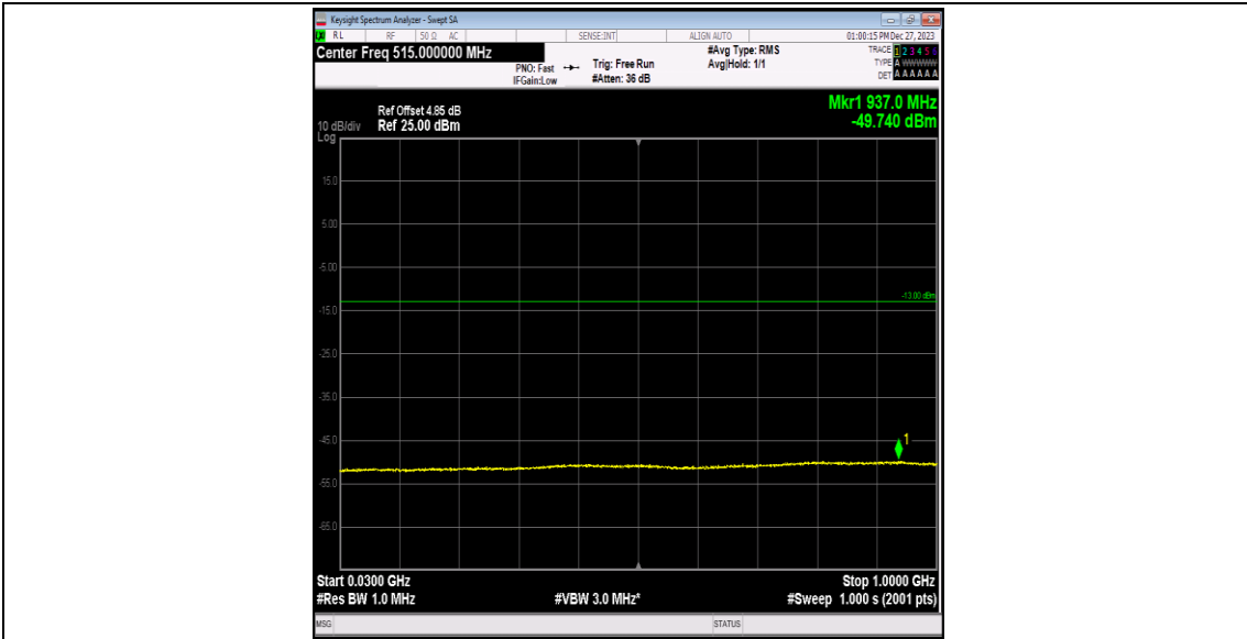
Band4-1312-2-30~1000MHz-PASS
