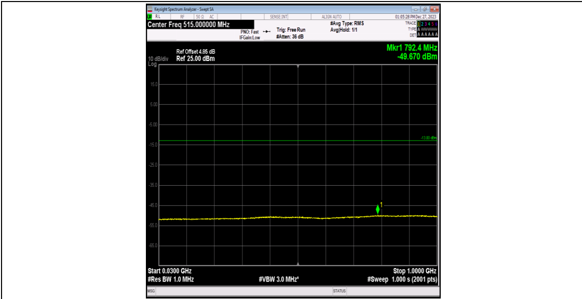
Band4-1413-4-30~1000MHz-PASS
