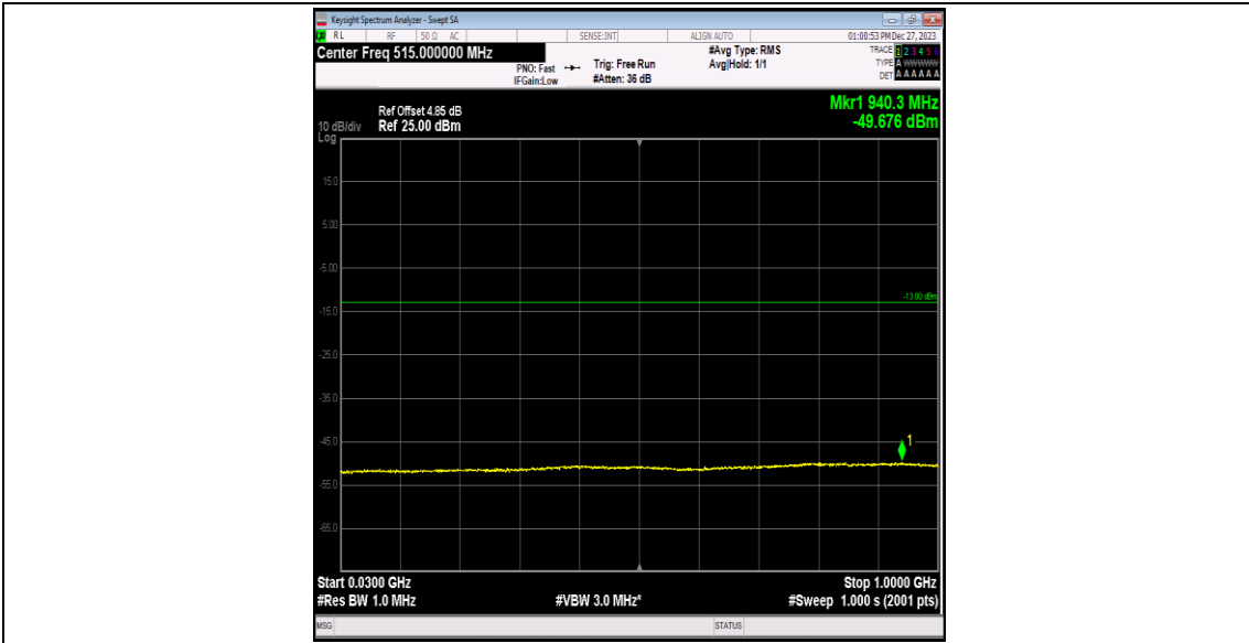
Band4-1413-2-30~1000MHz-PASS
