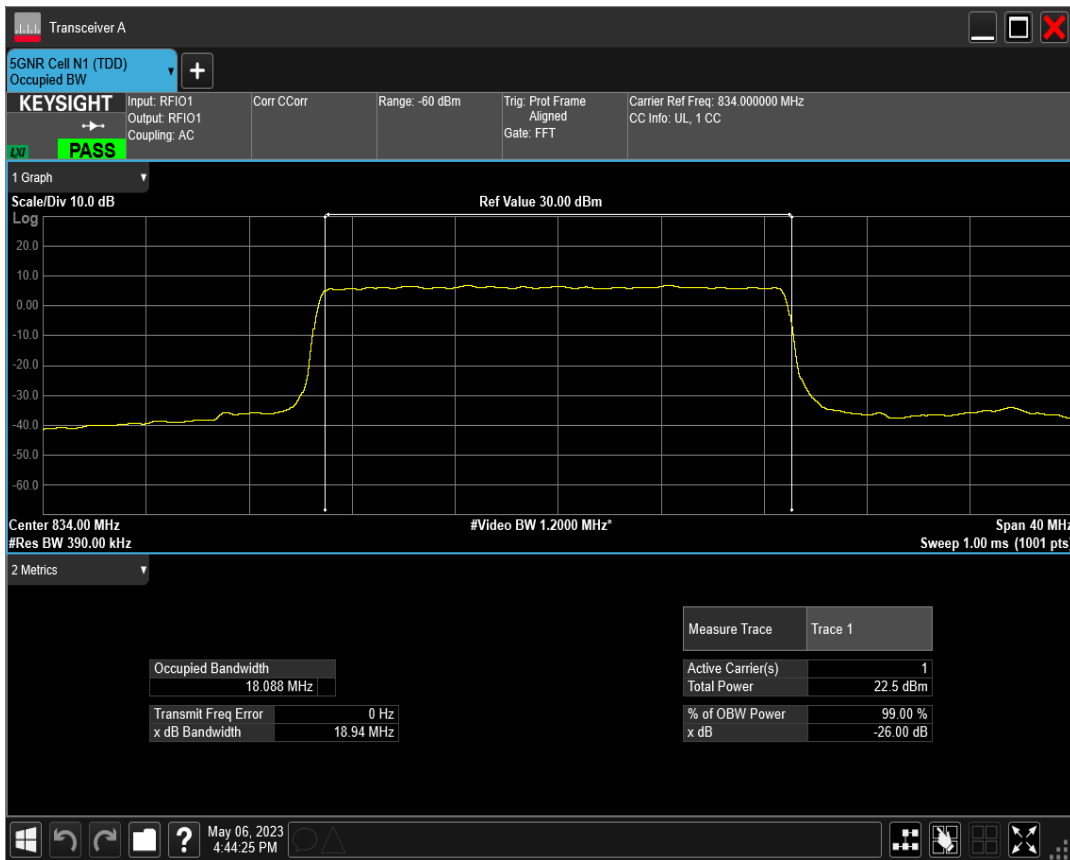
n5 SCS=30kHz DFT_QPSK BW=20MHz Channel=166800 RB=50@0
