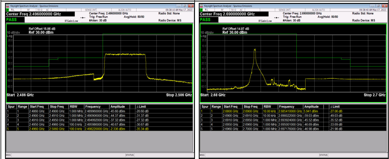
Band41-5MHz-64QAM-41565-1RB#24
