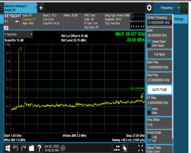
Band41-5MHz-16QAM-40640-1RB#0-Range2:1000~27000MHz
