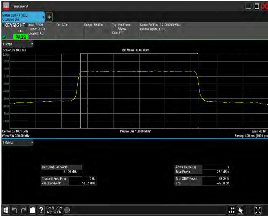
n78(3700-3800) SCS=30kHz DFT_QAM256 BW=20MHz Channel=647334 RB=50@0
