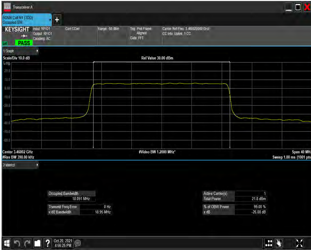
n77(3450-3550) SCS=30kHz CP_QPSK BW=20MHz Channel=630668 RB=51 @0
