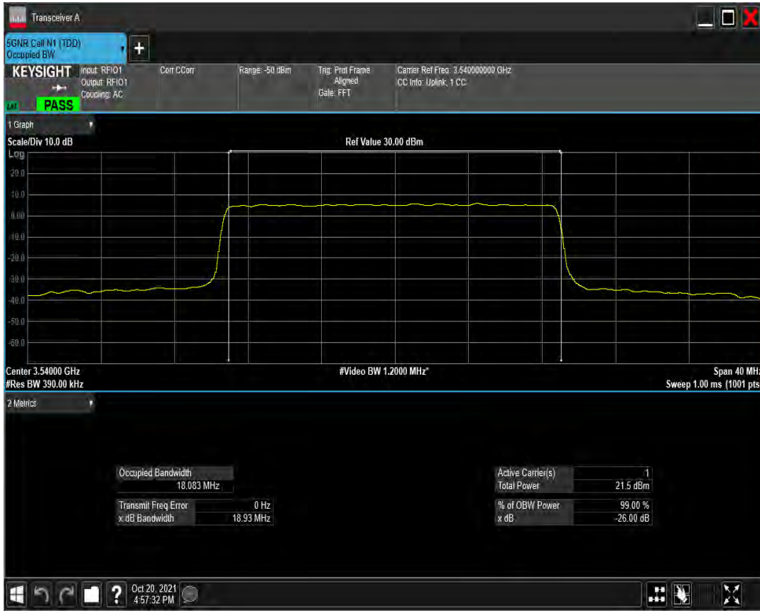
n77(3450-3550) SCS=30kHz CP_QPSK BW=20MHz Channel=636000 RB=51 @0
