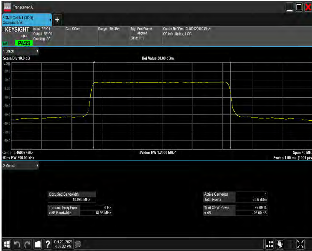
n77(3450-3550) SCS=30kHz DFT_QAM256 BW=20MHz Channel=630668 RB=50@0
