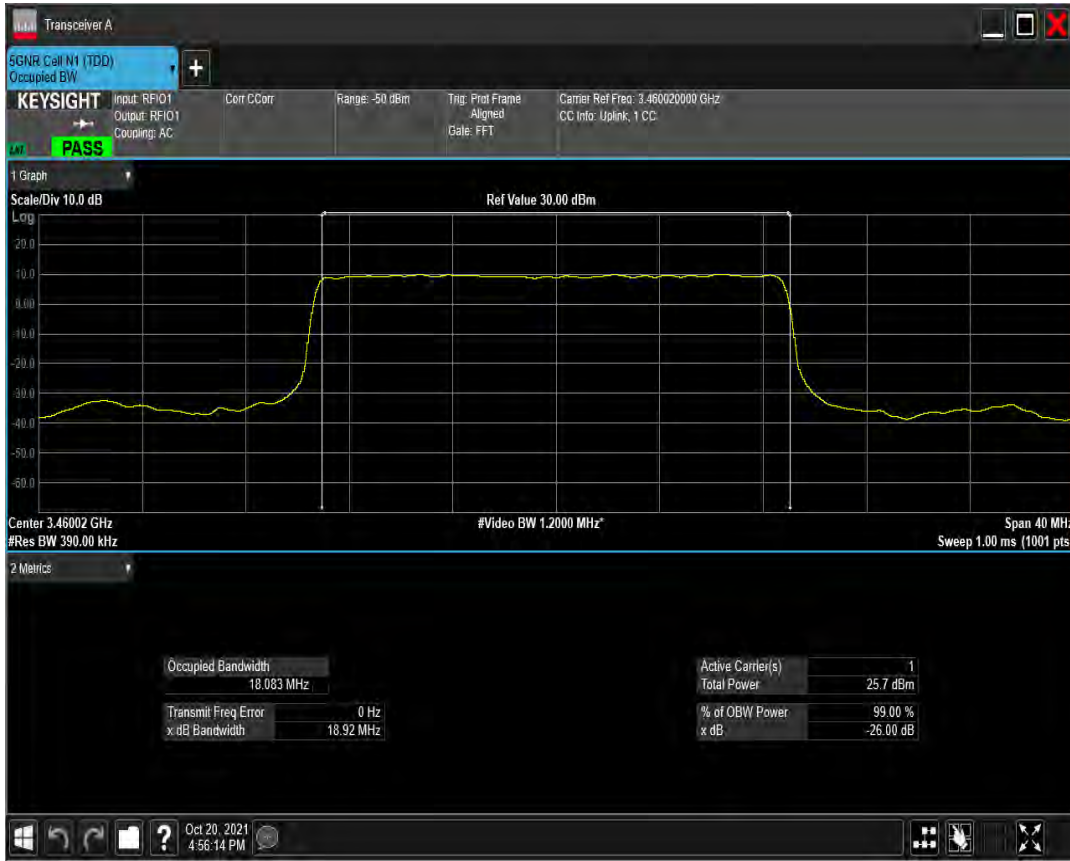
n77(3450-3550) SCS=30kHz DFT_QPSK BW=20MHz Channel=630668 RB=50@0
