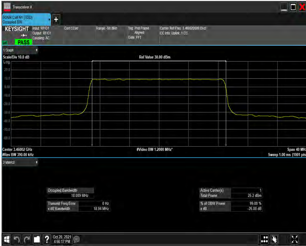
n77(3450-3550) SCS=30kHz DFT_QAM16 BW=20MHz Channel=630668 RB=50@0
