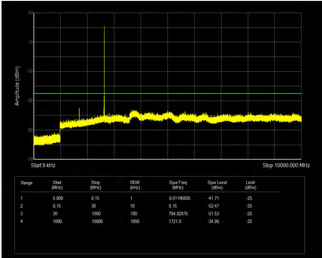
n41(2535-2655) SCS=30kHz DFT_QPSK BW=50MHz Channel=512004 RB=128@0
