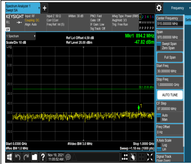
Band7-5MHz-QPSK-21425-1RB#0-Range1:30~10 00MHz
