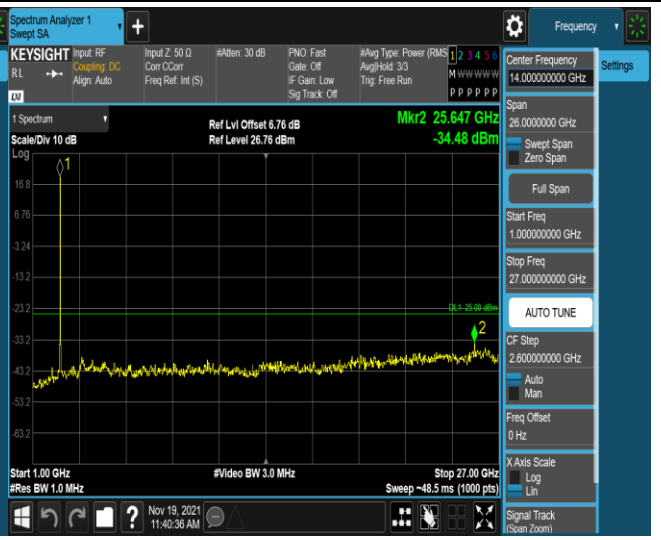
Band7-20MHz-QPSK-21100-1RB#0-Range2:1000~27000MHz
