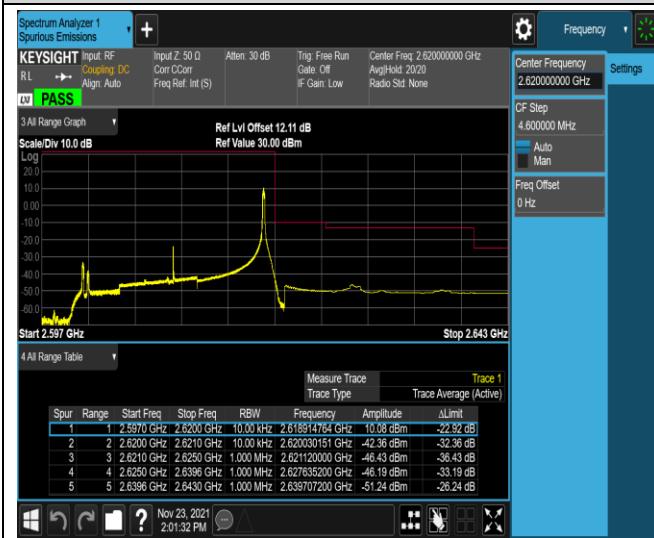
Band38-20MHz-QPSK-38150-1RB#99
