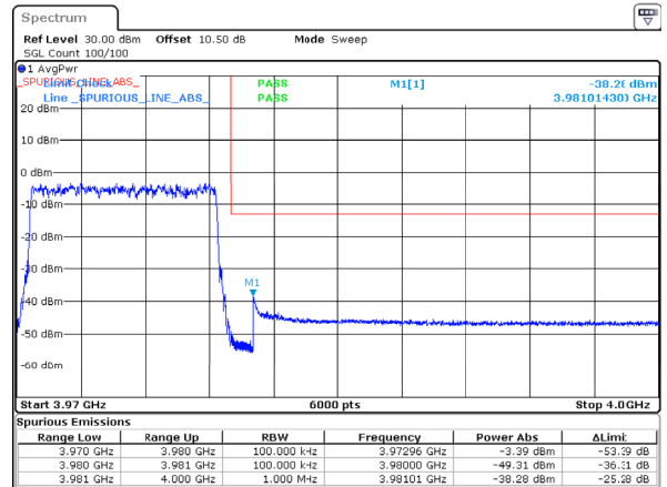
n77_3_10MHz_30kHz_3975MHz_DFT-s-OFDM QPSK_RB24@0 -38.284MHz
