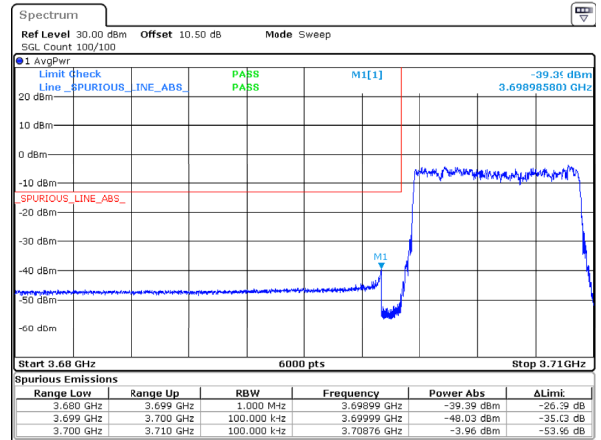
n77_3_10MHz_30kHz_3705MHz_DFT-s-OFDM QPSK_RB24@0 -39.389MHz
