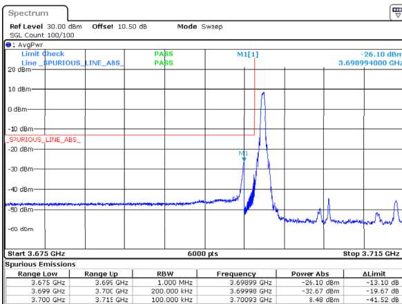
n77_3_15MHz_30kHz_3707.5MHz_DFT-s-OFDM QPSK_RB1@0 -26.101MHz
