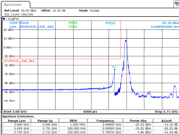
n77_3_10MHz_30kHz_3705MHz_DFT-s-OFDM QPSK_RB1@0 -26.101MHz
