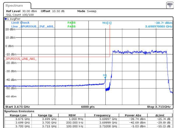
n77_3_15MHz_30kHz_3707.5MHz_DFT-s-OFDM QPSK_RB36@0 -38.736MHz
