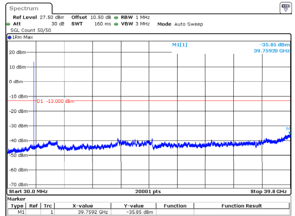
n77_3_20MHz_30kHz_3710MHz_DFT-s-OFDM QPSK_RB1@0 -35.85dBm
