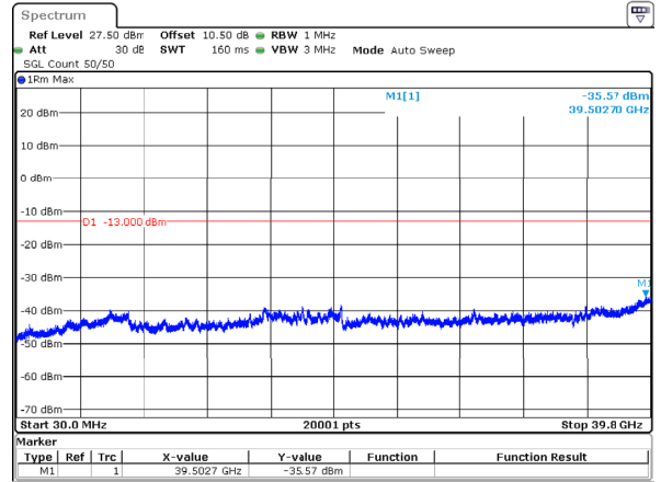
n77_3_15MHz_30kHz_3707.5MHz_DFT-s-OFDM QPSK_RB1@37 -35.57dBm
