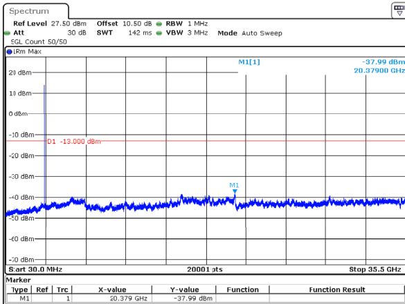
n77_1_80MHz_30kHz_3490MHz_DFT-s-OFDM QPSK_RB1@0 -37.99dBm
