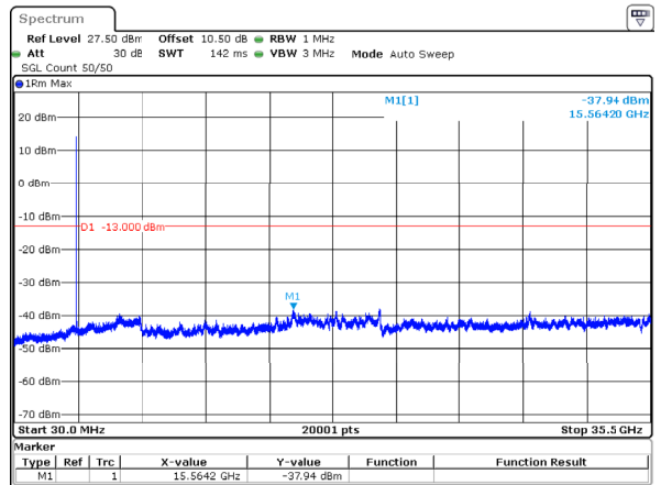
n77_1_30MHz_30kHz_3465MHz_DFT-s-OFDM QPSK_RB1@0 -37.94dBm
