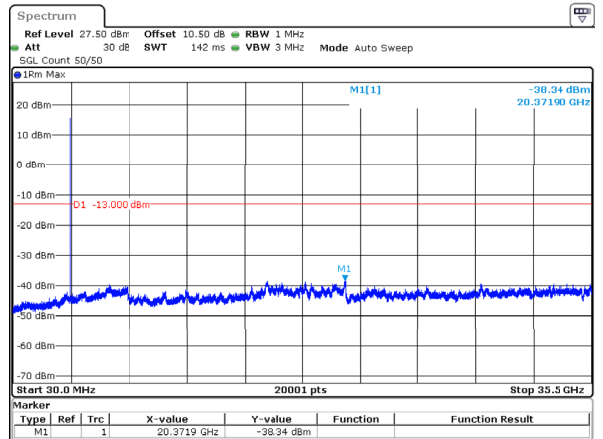
n77_1_10MHz_30kHz_3500MHz_DFT-s-OFDM QPSK_RB1@0 -38.34dBm
