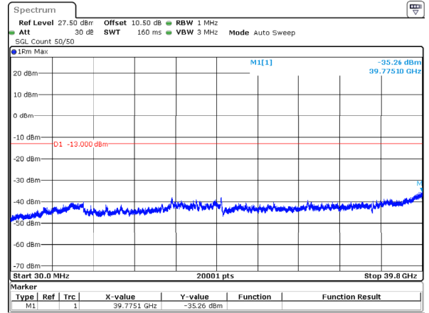
n77_3_15MHz_30kHz_3972.5MHz_DFT-s-OFDM QPSK_RB1@37 -35.26dBm
