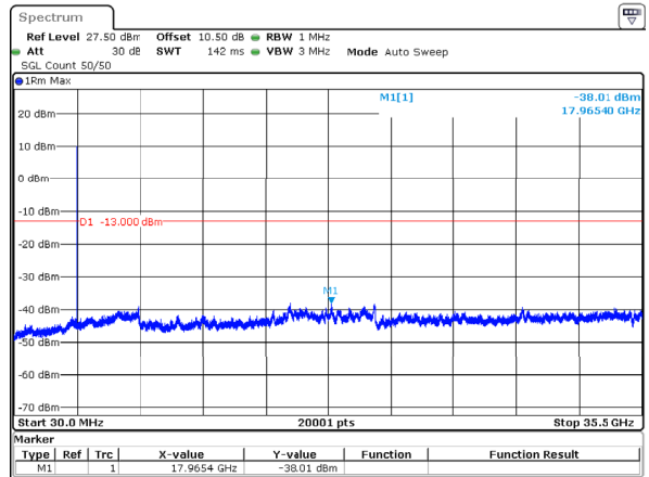
n77_1_80MHz_30kHz_3490MHz_DFT-s-OFDM QPSK_RB1@216 -38.01dBm
