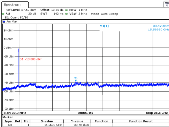
n77_1_100MHz_30kHz_3500MHz_DFT-s-OFDM QPSK_RB270@0 -38.42dBm
