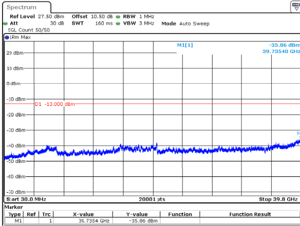
n77_3_15MHz_30kHz_3707.5MHz_DFT-s-OFDM QPSK_RB1@0 -35.86dBm
