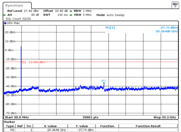
n77_1_30MHz_30kHz_3465MHz_DFT-s-OFDM QPSK_RB75@0 -37.74dBm
