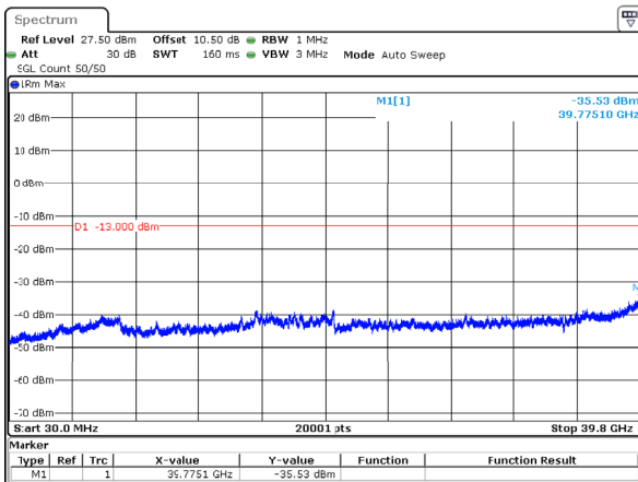
n77_3_20MHz_30kHz_3710MHz_DFT-s-OFDM QPSK_RB1@50 -35.53dBm
