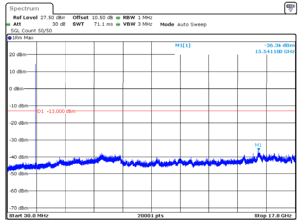
n66_40MHz_15kHz_1760MHz_DFT-s-OFDM QPSK_RB1@0 -36.36dBm
