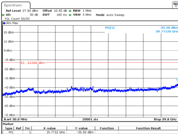
n77_3_10MHz_30kHz_3705MHz_DFT-s-OFDM QPSK_RB1@23 -35.50dBm
