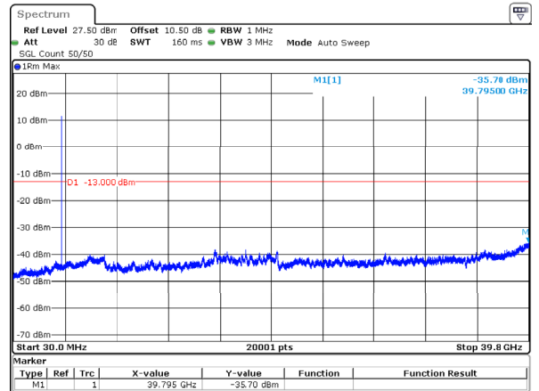
n77_3_10MHz_30kHz_3705MHz_DFT-s-OFDM QPSK_RB1@0 -35.70dBm
