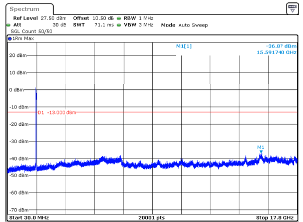
n66_40MHz_15kHz_1760MHz_DFT-s-OFDM QPSK_RB216@0 -36.87dBm
