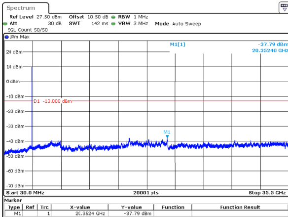
n77_1_10MHz_30kHz_3455MHz_DFT-s-OFDM QPSK_RB24@0 -37.79dBm
