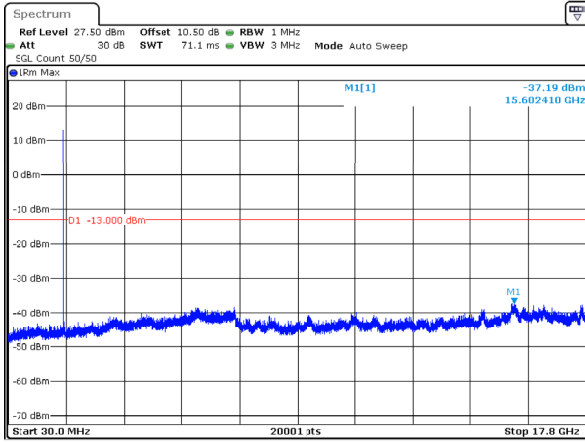
n66_40MHz_15kHz_1745MHz_DFT-s-OFDM QPSK_RB1@0 -37.19dBm
