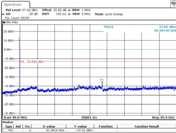
n77_1_10MHz_30kHz_3455MHz_DFT-s-OFDM QPSK_RB1@0 -37.01dBm
