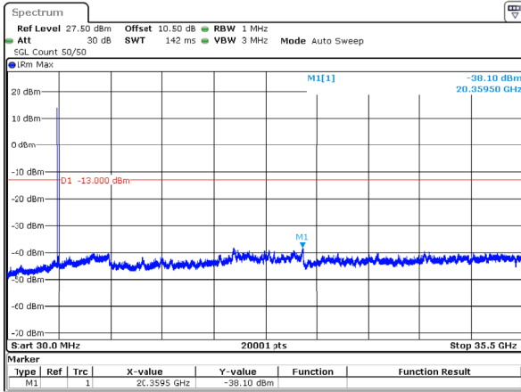
n77_1_100MHz_30kHz_3500MHz_DFT-s-OFDM QPSK_RB1@0 -38.10dBm
