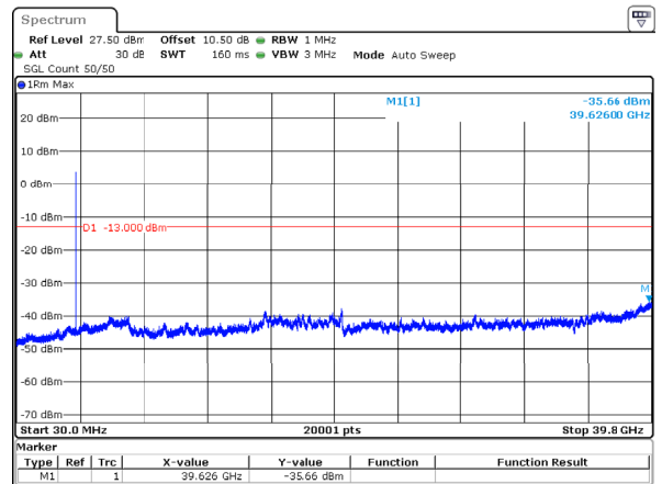
n77_3_20MHz_30kHz_3710MHz_DFT-s-OFDM QPSK_RB50@0 -35.66dBm
