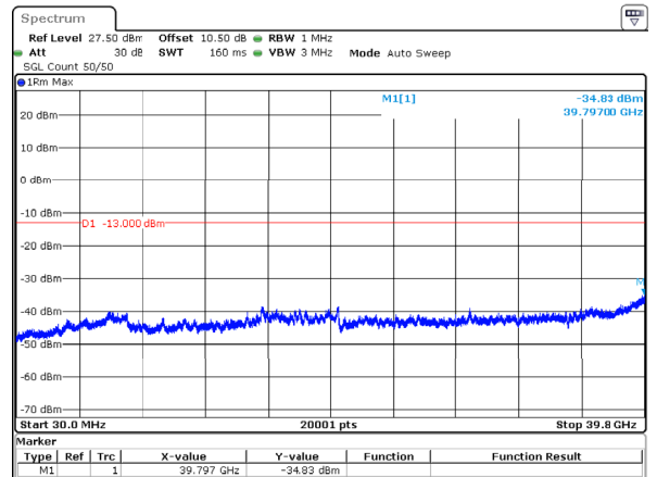
n77_3_10MHz_30kHz_3705MHz_DFT-s-OFDM QPSK_RB24@0 -34.83dBm
