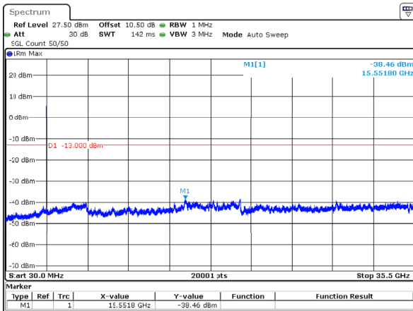
n77_1_20MHz_30kHz_3540MHz_DFT-s-OFDM QPSK_RB50@0 -38.46dBm
