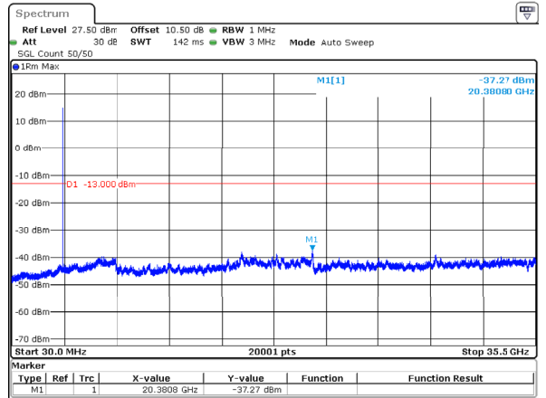
n77_1_10MHz_30kHz_3455MHz_DFT-s-OFDM QPSK_RB1@23 -37.27dBm
