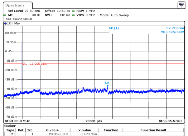
n77_1_10MHz_30kHz_3500MHz_DFT-s-OFDM QPSK_RB24@0 -37.73dBm
