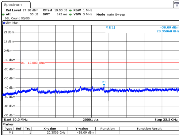
n77_1_10MHz_30kHz_3545MHz_DFT-s-OFDM QPSK_RB24@0 -38.09dBm
