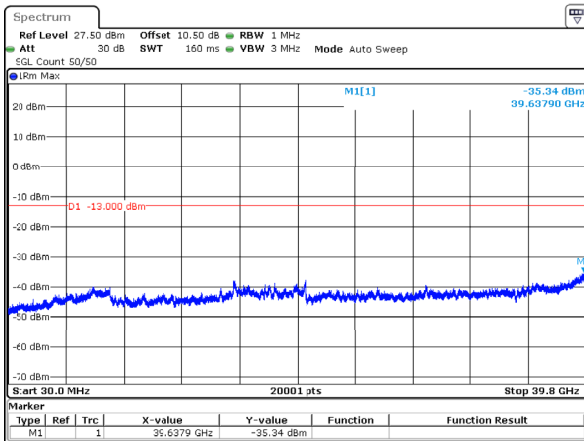
n77_3_15MHz_30kHz_3707.5MHz_DFT-s-OFDM QPSK_RB36@0 -35.34dBm
