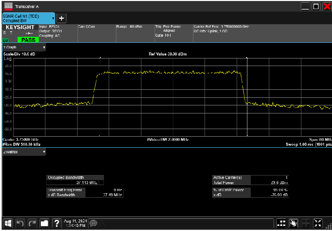
n78_3_40MHz_30kHz_3750MHz_CP-OFDM QPSK_RB106@0 37.780MHz
