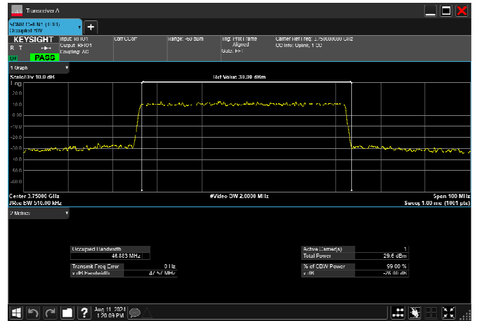
n78_3_50MHz_30kHz_3750MHz_CP-OFDM QPSK_RB133@0 47.407MHz
