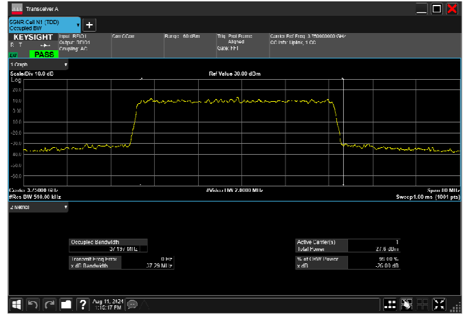
n78_3_40MHz_30kHz_3750MHz_CP-OFDM 16 QAM_RB106@0 37.778MHz
