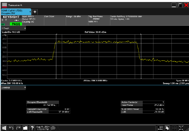
n78_3_40MHz_30kHz_3750MHz_DFT-s-OFDM QPSK_RB100@0 37.452MHz
