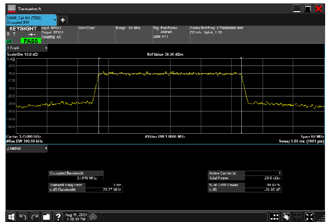
n78_3_30MHz_30kHz_3750MHz_CP-OFDM QPSK_RB78@0 27.848MHz
