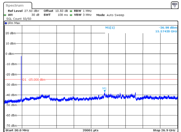
n41_30MHz_30kHz_2592.99MHz_DFT-s-OFDM QPSK_RB75@0 -36.98dBm
