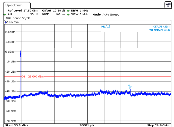
n41_100MHz_30kHz_2592.99MHz_DFT-s-OFDM QPSK_RB270@0 -37.58dBm
