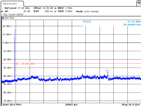
n41_40MHz_30kHz_2516.01MHz_DFT-s-OFDM QPSK_RB1@0 -37.12dBm
