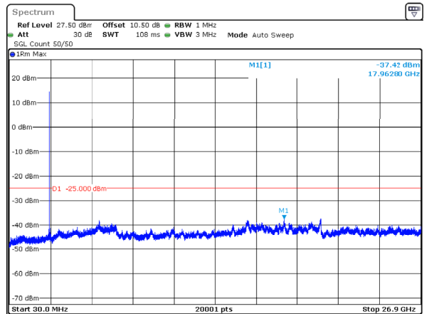
n41_90MHz_30kHz_2644.98MHz_DFT-s-OFDM QPSK_RB1@0 -37.42dBm
