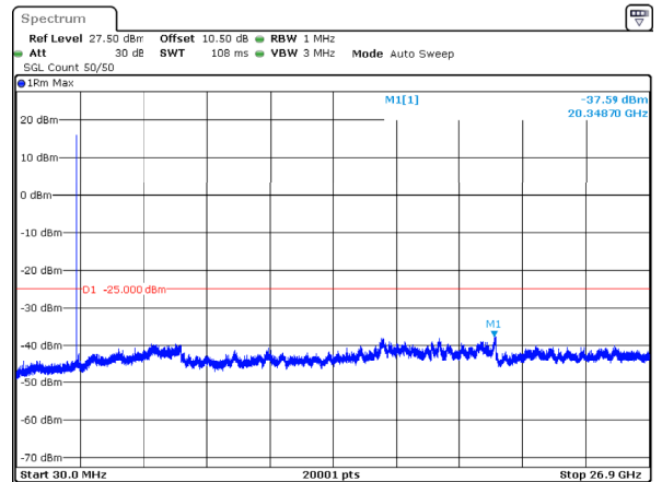
n41_100MHz_30kHz_2592.99MHz_DFT-s-OFDM QPSK_RB1@0 -37.59dBm
