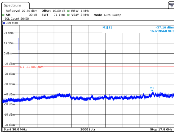
n66_15MHz_15kHz_1717.5MHz_DFT-s-OFDM QPSK_RB1@78 -37.16dBm
