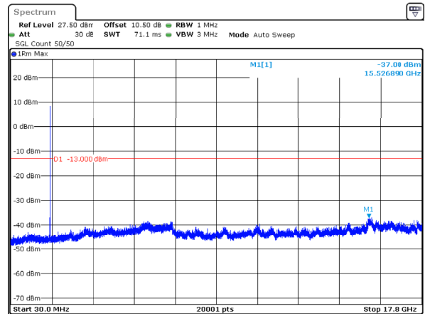
n66_5MHz_15kHz_1712.5MHz_DFT-s-OFDM QPSK_RB25@0 -37dBm
