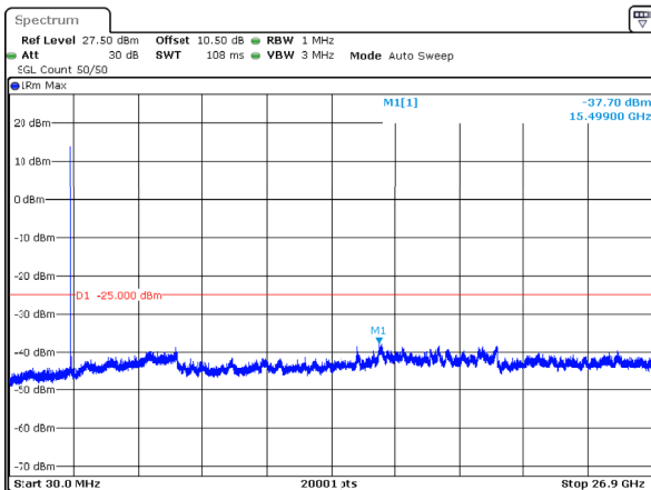
n41_50MHz_30kHz_2592.99MHz_DFT-s-OFDM QPSK_RB1@0 -37.70dBm
