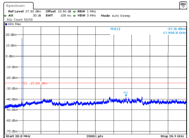
n41_60MHz_30kHz_2526MHz_DFT-s-OFDM QPSK_RB1@161 -37.21dBm
