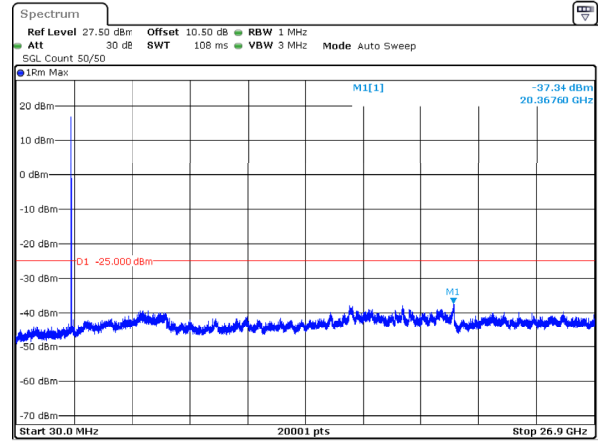
n41_60MHz_30kHz_2592.99MHz_DFT-s-OFDM QPSK_RB1@0 -37.34dBm
