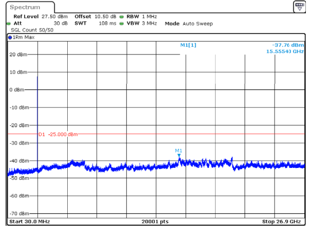
n41_30MHz_30kHz_2674.98MHz_DFT-s-OFDM QPSK_RB1@77 -37.76dBm
