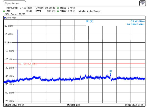
n41_50MHz_30kHz_2664.99MHz_DFT-s-OFDM QPSK_RB1@0 -37.42dBm
