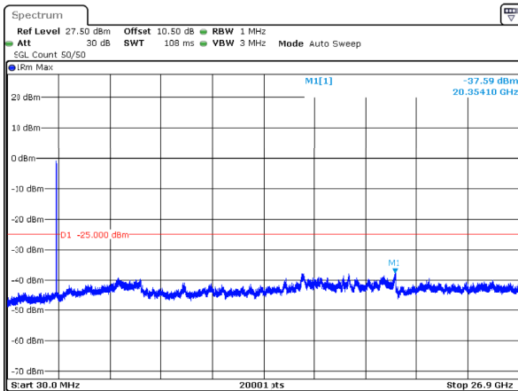
n41_20MHz_30kHz_2592.99MHz_DFT-s-OFDM QPSK_RB50@0 -37.59dBm
