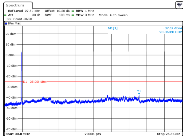
n41_60MHz_30kHz_2526MHz_DFT-s-OFDM QPSK_RB162@0 -37.17dBm
