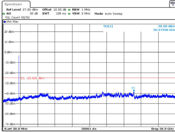
n41_15MHz_30kHz_2503.5MHz_DFT-s-OFDM QPSK_RB1@0 -38dBm
