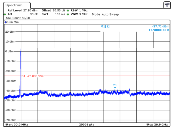
n41_80MHz_30kHz_2592.99MHz_DFT-s-OFDM QPSK_RB216@0 -37.72dBm
