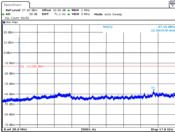
n66_10MHz_15kHz_1715MHz_DFT-s-OFDM QPSK_RB1@0 -37.16dBm
