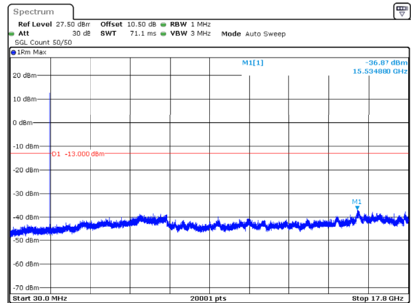
n66_15MHz_15kHz_1772.5MHz_DFT-s-OFDM QPSK_RB1@0 -36.87dBm
