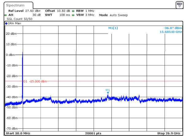
n41_60MHz_30kHz_2659.98MHz_DFT-s-OFDM QPSK_RB162@0 -36.87dBm
