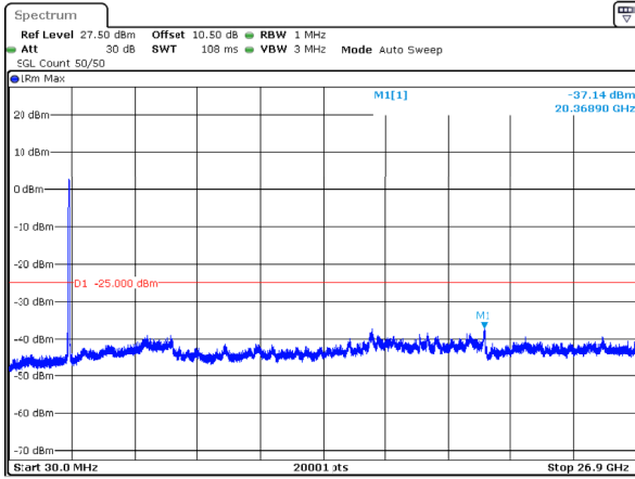
n41_60MHz_30kHz_2592.99MHz_DFT-s-OFDM QPSK_RB162@0 -37.14dBm
