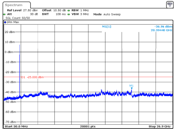
n41_20MHz_30kHz_2506.02MHz_DFT-s-OFDM QPSK_RB1@0 -36.96dBm
