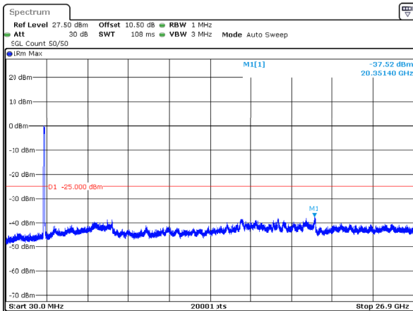
n41_100MHz_30kHz_2546.01MHz_DFT-s-OFDM QPSK_RB270@0 -37.52dBm
