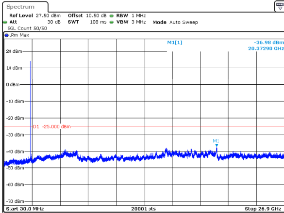
n41_90MHz_30kHz_2592.99MHz_DFT-s-OFDM QPSK_RB1@0 -36.98dBm
