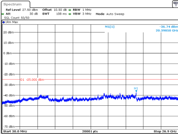
n41_30MHz_30kHz_2674.98MHz_DFT-s-OFDM QPSK_RB1@0 -36.74dBm
