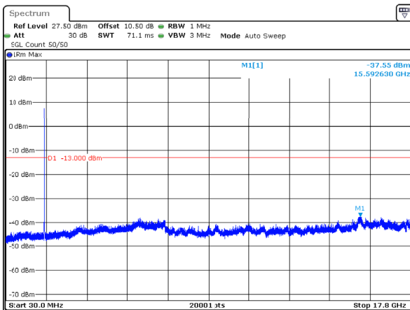
n66_10MHz_15kHz_1715MHz_DFT-s-OFDM QPSK_RB50@0 -37.55dBm
