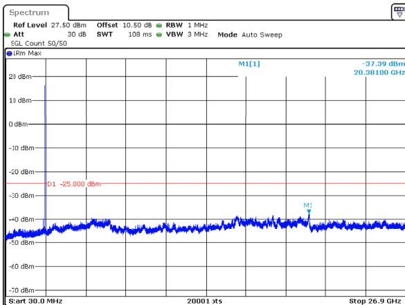
n41_100MHz_30kHz_2592.99MHz_DFT-s-OFDM QPSK_RB1@272 -37.39dBm
