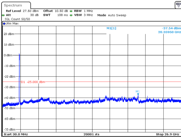
n41_80MHz_30kHz_2536.02MHz_DFT-s-OFDM QPSK_RB216@0 -37.54dBm
