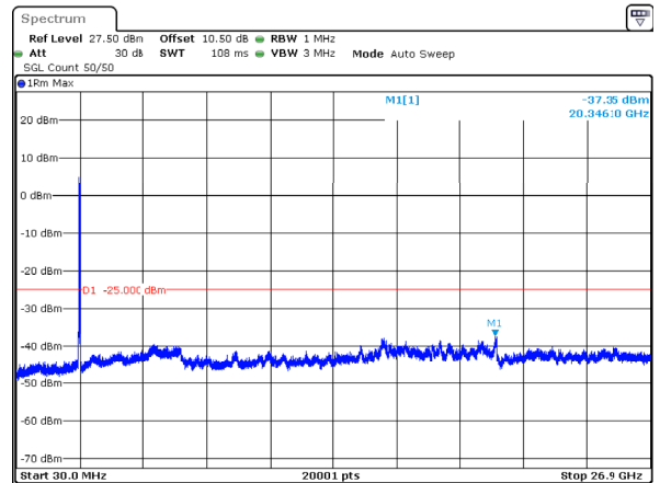
n41_40MHz_30kHz_2670MHz_DFT-s-OFDM QPSK_RB100@0 -37.35dBm
