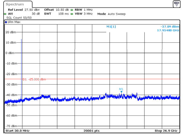
n41_80MHz_30kHz_2536.02MHz_DFT-s-OFDM QPSK_RB1@216 -37.89dBm
