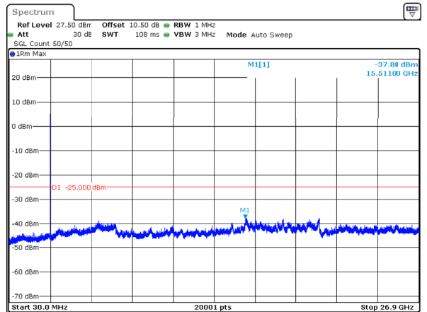
n41_20MHz_30kHz_2679.99MHz_DFT-s-OFDM QPSK_RB1@0 -37.80dBm
