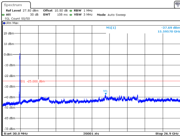
n41_100MHz_30kHz_2640MHz_DFT-s-OFDM QPSK_RB270@0 -37.69dBm
