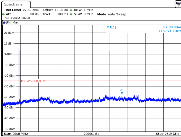
n41_80MHz_30kHz_2536.02MHz_DFT-s-OFDM QPSK_RB1@0 -37.30dBm
