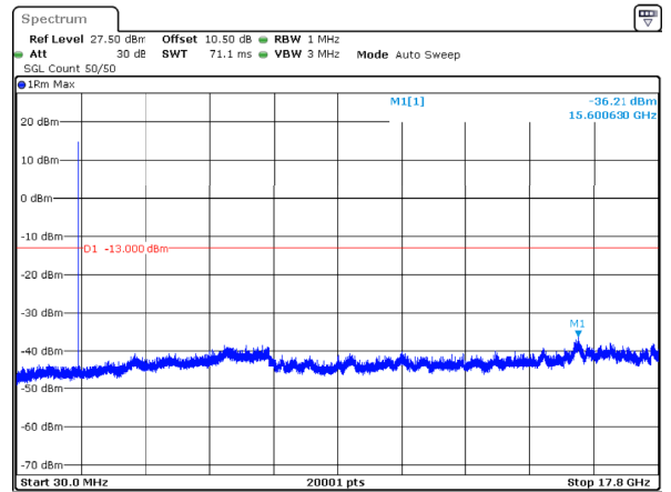
n66_15MHz_15kHz_1717.5MHz_DFT-s-OFDM QPSK_RB1@0 -36.21dBm
