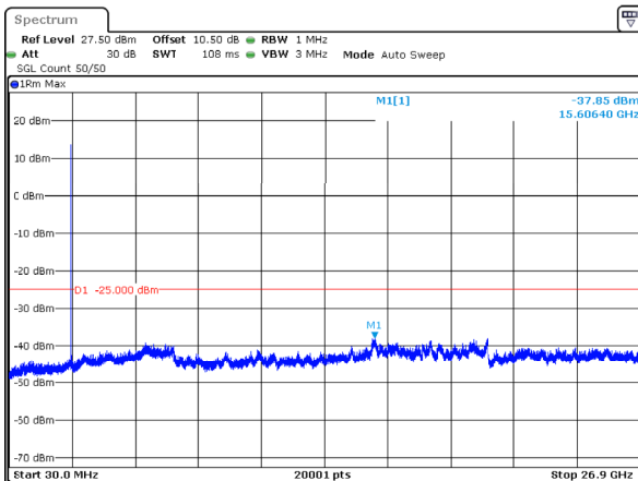
n41_40MHz_30kHz_2670MHz_DFT-s-OFDM QPSK_RB1@0 -37.85dBm
