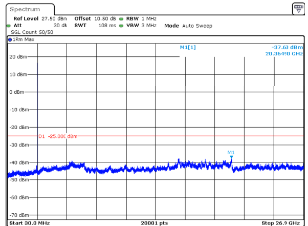
n41_40MHz_30kHz_2670MHz_DFT-s-OFDM QPSK_RB1@105 -37.60dBm
