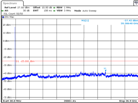
n41_100MHz_30kHz_2640MHz_DFT-s-OFDM QPSK_RB1@0 -37.42dBm
