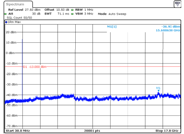
n66_20MHz_15kHz_1770MHz_DFT-s-OFDM QPSK_RB1@0 -36.93dBm
