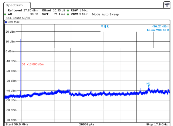
n66_25MHz_15kHz_1722.5MHz_DFT-s-OFDM QPSK_RB1@132 -36.27dBm
