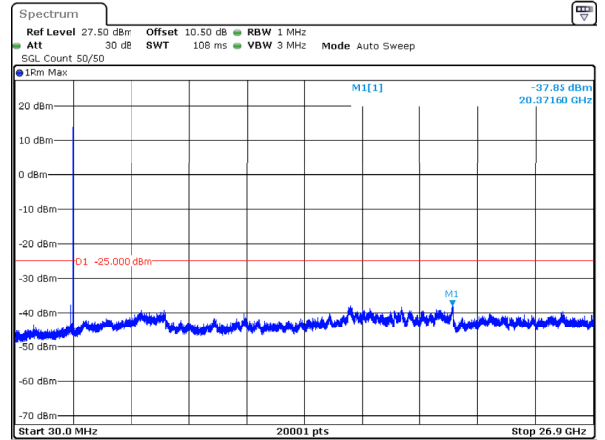
n41_100MHz_30kHz_2640MHz_DFT-s-OFDM QPSK_RB1@272 -37.85dBm
