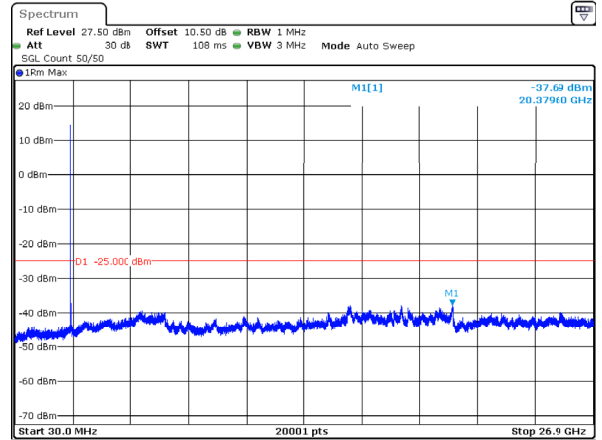
n41_40MHz_30kHz_2592.99MHz_DFT-s-OFDM QPSK_RB1@0 -37.69dBm
