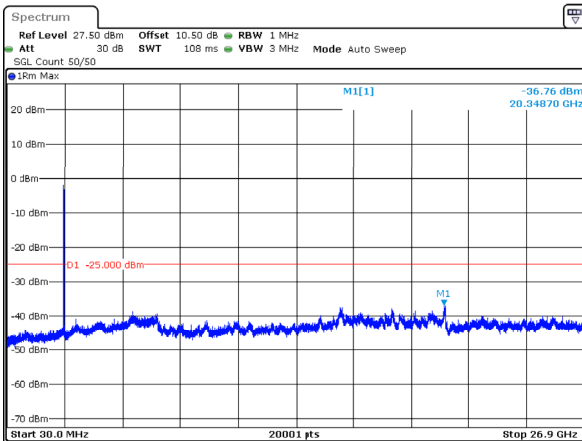
n41_30MHz_30kHz_2674.98MHz_DFT-s-OFDM QPSK_RB75@0 -36.76dBm
