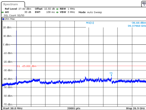
n41_50MHz_30kHz_2664.99MHz_DFT-s-OFDM QPSK_RB1@132 -36.66dBm
