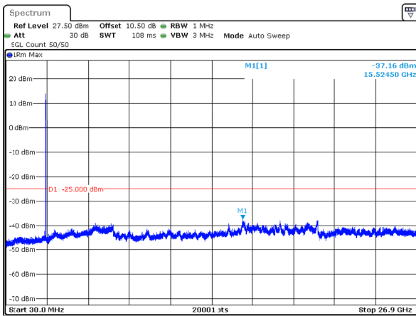
n41_80MHz_30kHz_2592.99MHz_DFT-s-OFDM QPSK_RB1@216 -37.16dBm
