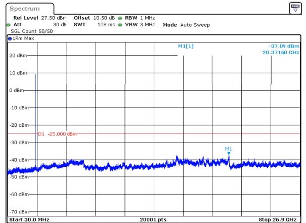
n41_30MHz_30kHz_2592.99MHz_DFT-s-OFDM QPSK_RB1@0 -37.09dBm
