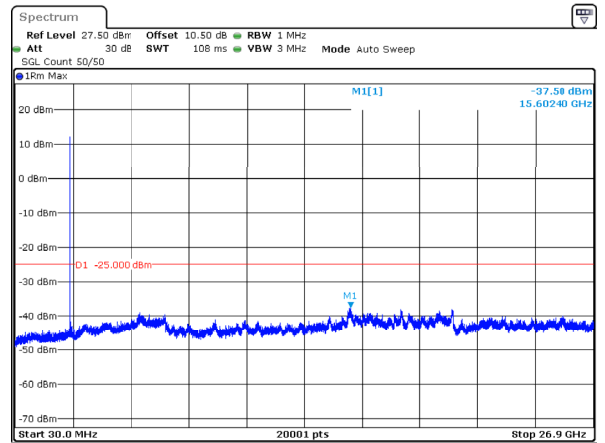
n41_80MHz_30kHz_2592.99MHz_DFT-s-OFDM QPSK_RB1@0 -37.50dBm
