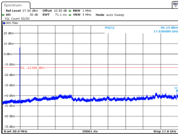
n66_10MHz_15kHz_1775MHz_DFT-s-OFDM QPSK_RB50@0 -36.13dBm
