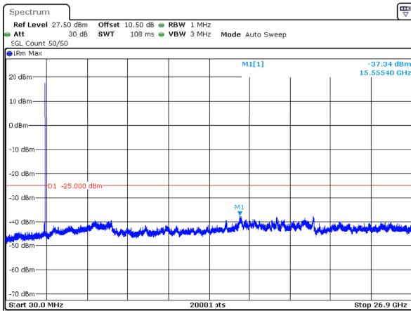
n41_60MHz_30kHz_2592.99MHz_DFT-s-OFDM QPSK_RB1@161 -37.34dBm
