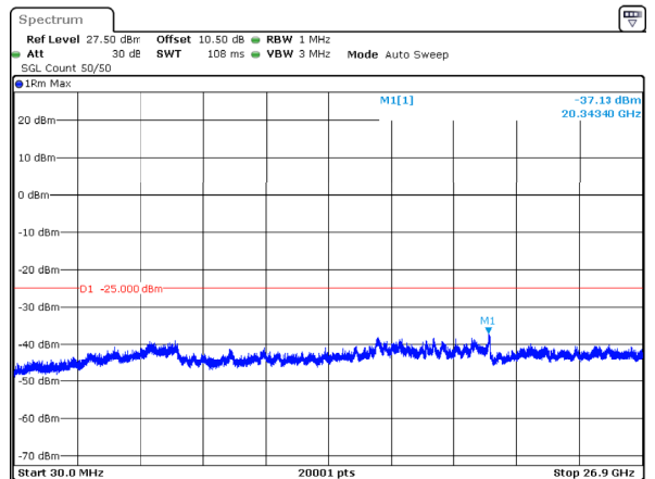
n41_20MHz_30kHz_2679.99MHz_DFT-s-OFDM QPSK_RB50@0 -37.13dBm
