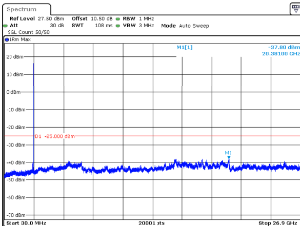
n41_90MHz_30kHz_2644.98MHz_DFT-s-OFDM QPSK_RB1@244 -37.80dBm
