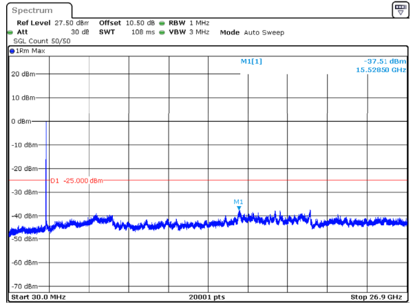
n41_20MHz_30kHz_2506.02MHz_DFT-s-OFDM QPSK_RB50@0 -37.51dBm
