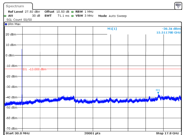
n66_10MHz_15kHz_1745MHz_DFT-s-OFDM QPSK_RB50@0 -36.56dBm
