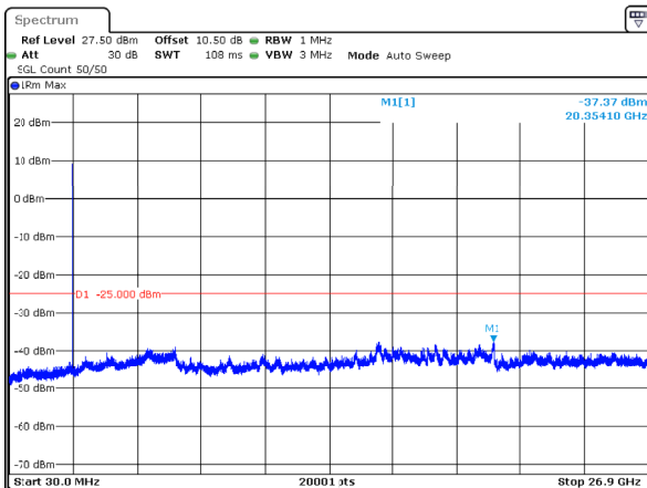
n41_20MHz_30kHz_2679.99MHz_DFT-s-OFDM QPSK_RB1@50 -37.37dBm
