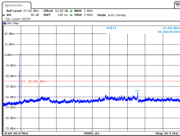
n41_15MHz_30kHz_2503.5MHz_DFT-s-OFDM QPSK_RB36@0 -37.60dBm
