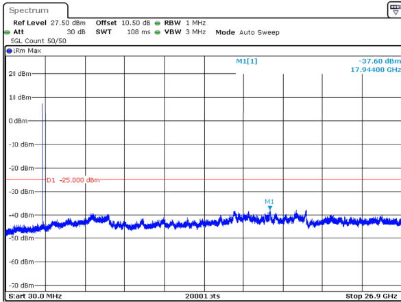
n41_20MHz_30kHz_2506.02MHz_DFT-s-OFDM QPSK_RB1@50 -37.60dBm
