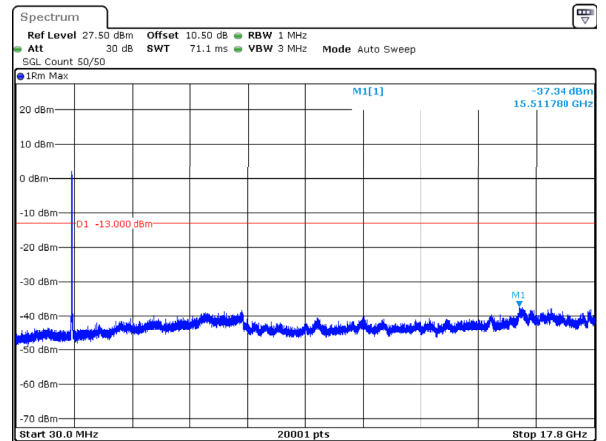
n66_25MHz_15kHz_1722.5MHz_DFT-s-OFDM QPSK_RB128@0 -37.34dBm
