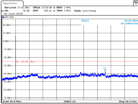
n41_15MHz_30kHz_2682.48MHz_DFT-s-OFDM QPSK_RB1@0 -36.66dBm
