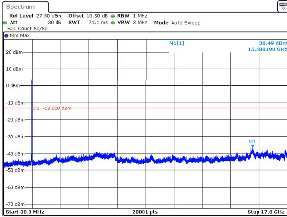
n66_20MHz_15kHz_1770MHz_DFT-s-OFDM QPSK_RB100@0 -36.49dBm
