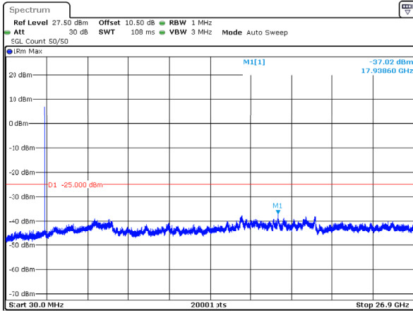
n41_20MHz_30kHz_2592.99MHz_DFT-s-OFDM QPSK_RB1@0 -37.02dBm
