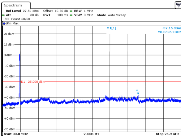
n41_90MHz_30kHz_2592.99MHz_DFT-s-OFDM QPSK_RB243@0 -37.15dBm
