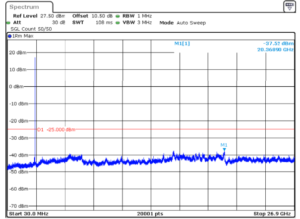
n41_100MHz_30kHz_2546.01MHz_DFT-s-OFDM QPSK_RB1@272 -37.52dBm
