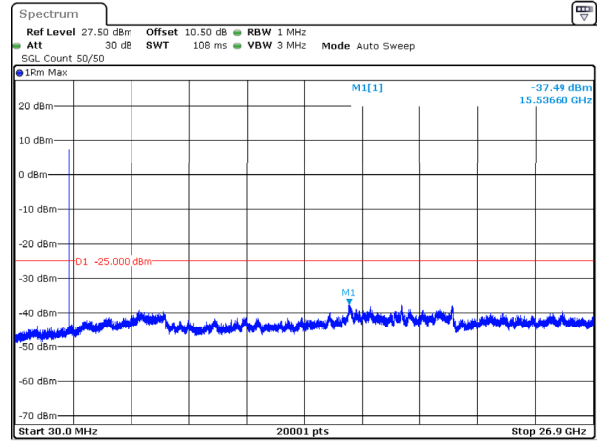
n41_30MHz_30kHz_2511MHz_DFT-s-OFDM QPSK_RB1@77 -37.49dBm
