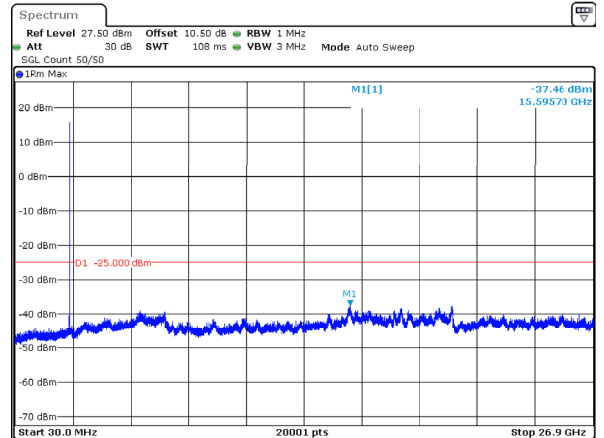
n41_40MHz_30kHz_2516.01MHz_DFT-s-OFDM QPSK_RB1@105 -37.46dBm
