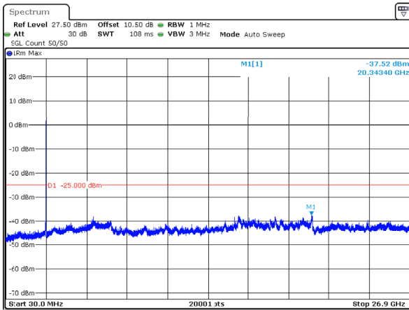
n41_15MHz_30kHz_2682.48MHz_DFT-s-OFDM QPSK_RB36@0 -37.52dBm
