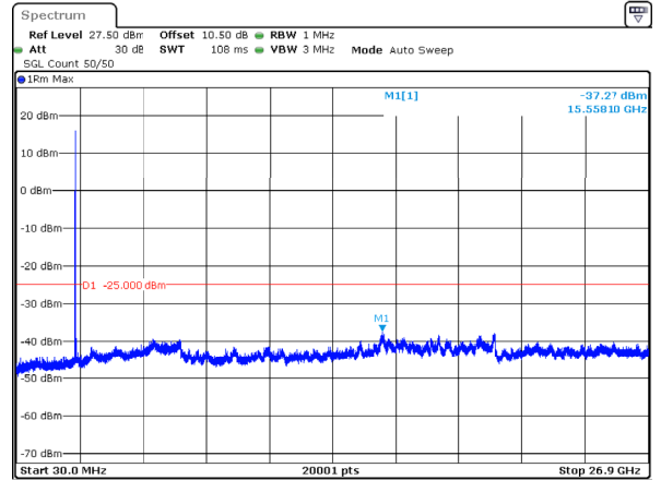
n41_50MHz_30kHz_2521.02MHz_DFT-s-OFDM QPSK_RB1@0 -37.27dBm
