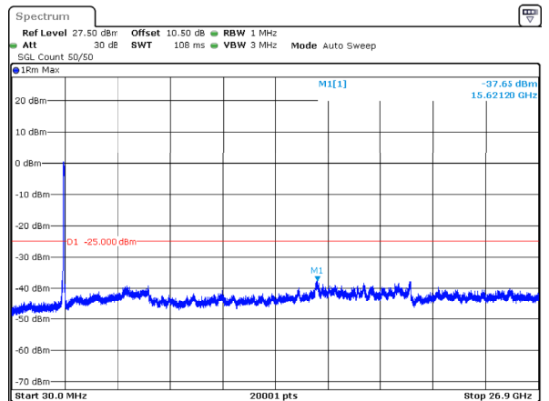
n41_90MHz_30kHz_2644.98MHz_DFT-s-OFDM QPSK_RB243@0 -37.65dBm
