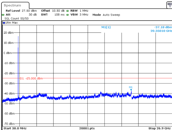
n41_60MHz_30kHz_2526MHz_DFT-s-OFDM QPSK_RB1@0 -37.18dBm
