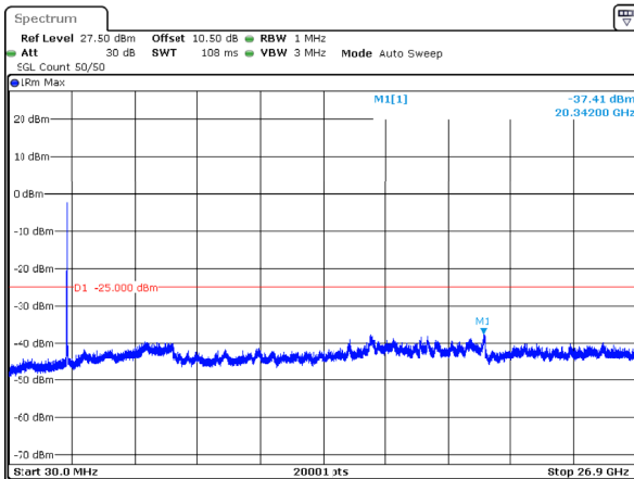
n41_30MHz_30kHz_2511MHz_DFT-s-OFDM QPSK_RB75@0 -37.41dBm
