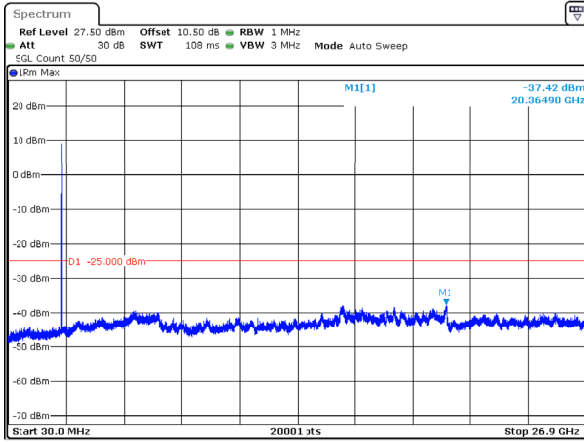
n41_30MHz_30kHz_2511MHz_DFT-s-OFDM QPSK_RB1@0 -37.42dBm
