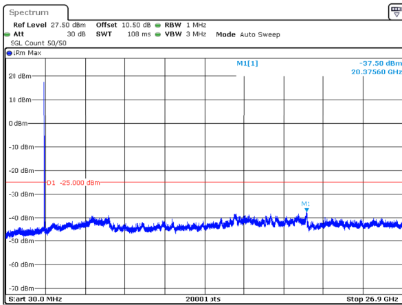
n41_60MHz_30kHz_2659.98MHz_DFT-s-OFDM QPSK_RB1@0 -37.50dBm
