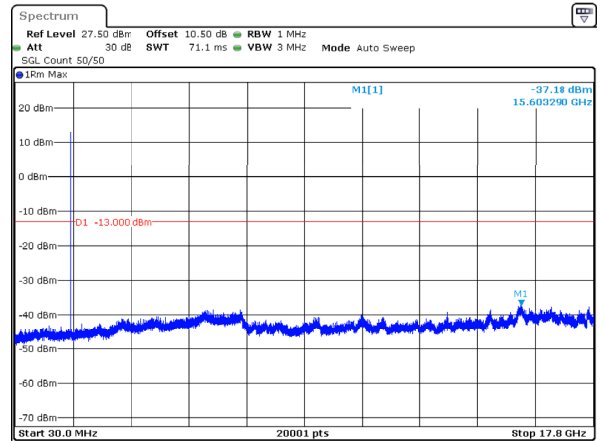
n66_5MHz_15kHz_1712.5MHz_DFT-s-OFDM QPSK_RB1@0 -37.18dBm
