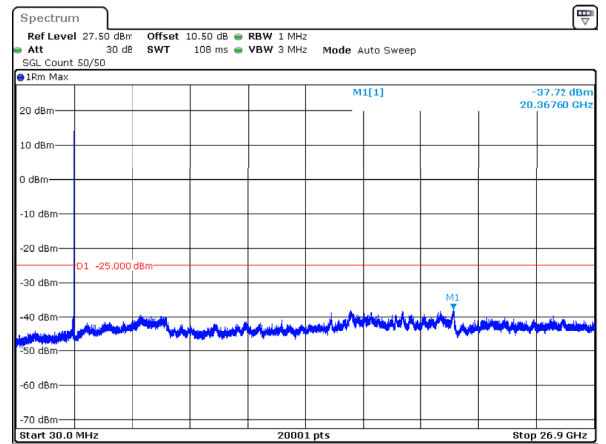
n41_60MHz_30kHz_2659.98MHz_DFT-s-OFDM QPSK_RB1@161 -37.72dBm
