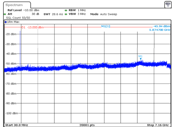
n12_15MHz_15kHz_707.5MHz_DFT-s-OFDM QPSK_RB1@0 -45.94dBm
