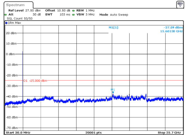
n7_5MHz_15kHz_2535MHz_DFT-s-OFDM QPSK_RB1@0 -37.09dBm
