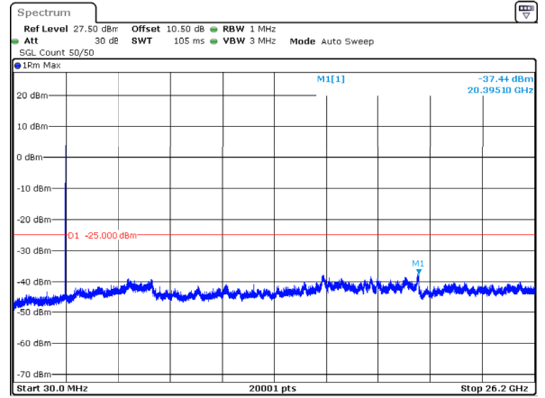
n38_10MHz_30kHz_2595MHz_DFT-s-OFDM QPSK_RB1@23 -37.44dBm
