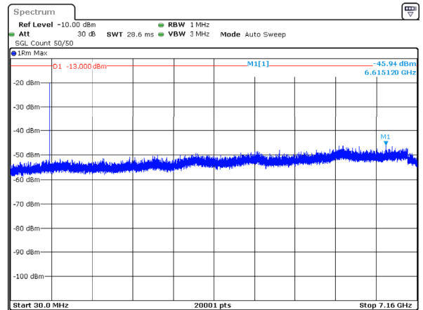
n12_5MHz_15kHz_707.5MHz_DFT-s-OFDM QPSK_RB25@0 -45.94dBm
