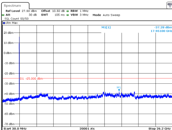
n38_5MHz_15kHz_2595MHz_DFT-s-OFDM QPSK_RB1@24 -37.28dBm
