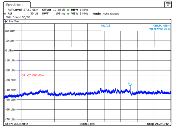
n41_10MHz_30kHz_2501.01MHz_DFT-s-OFDM QPSK_RB1@0 -36.91dBm
