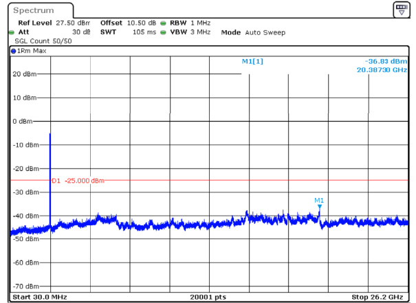
n38_30MHz_30kHz_2605MHz_DFT-s-OFDM QPSK_RB75@0 -36.83dBm
