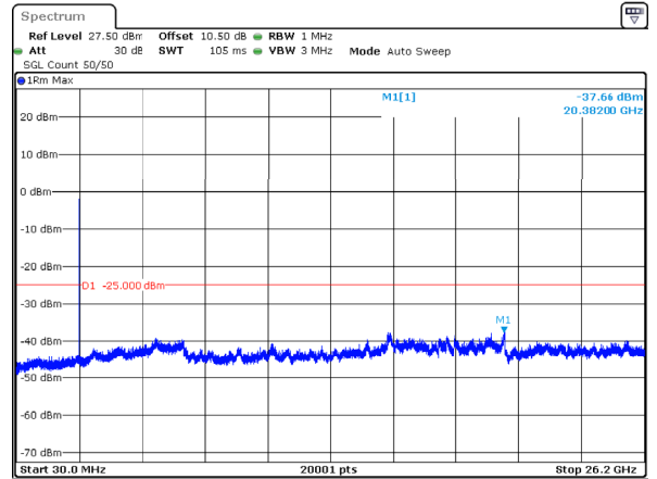
n38_10MHz_30kHz_2615MHz_DFT-s-OFDM QPSK_RB24@0 -37.66dBm
