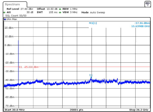
n38_30MHz_30kHz_2605MHz_DFT-s-OFDM QPSK_RB1@0 -37.95dBm
