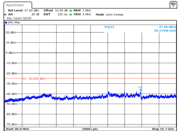
n7_5MHz_15kHz_2535MHz_DFT-s-OFDM QPSK_RB25@0 -37.06dBm
