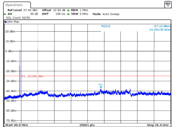
n41_10MHz_30kHz_2501.01MHz_DFT-s-OFDM QPSK_RB24@0 -37.15dBm
