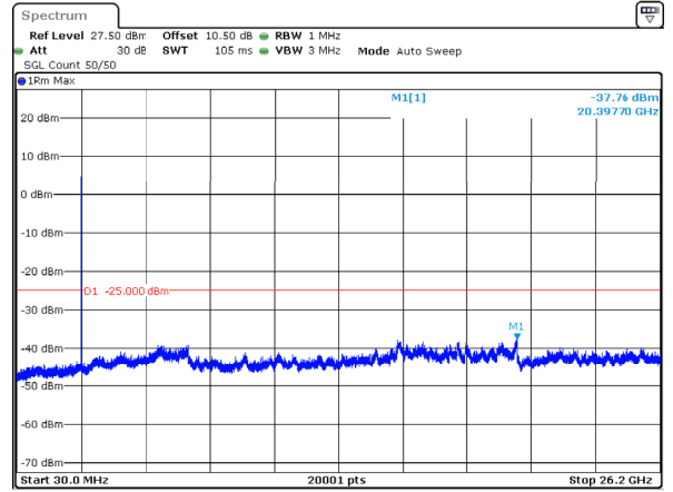
n38_30MHz_30kHz_2595MHz_DFT-s-OFDM QPSK_RB1@77 -37.76dBm
