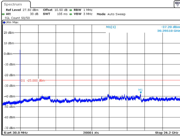
n38_10MHz_30kHz_2595MHz_DFT-s-OFDM QPSK_RB1@0 -37.20dBm
