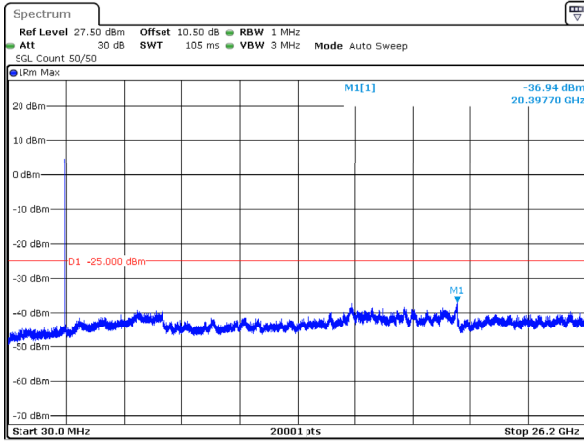
n38_30MHz_30kHz_2595MHz_DFT-s-OFDM QPSK_RB1@0 -36.94dBm
