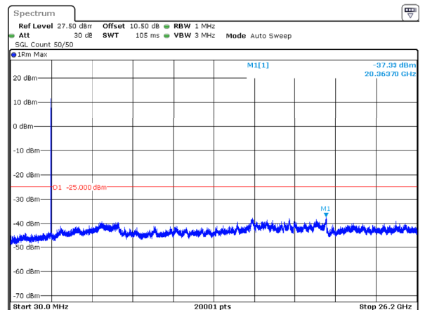
n38_5MHz_15kHz_2595MHz_DFT-s-OFDM QPSK_RB25@0 -37.33dBm
