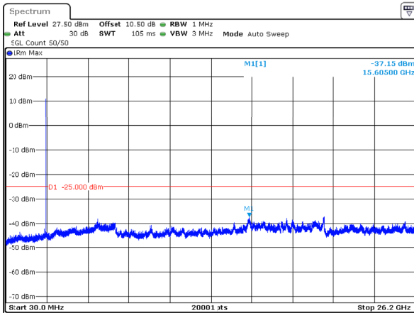
n38_5MHz_15kHz_2572.5MHz_DFT-s-OFDM QPSK_RB25@0 -37.15dBm
