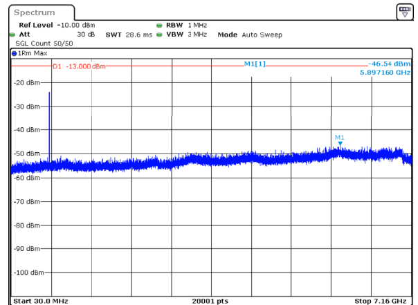
n12_10MHz_15kHz_704MHz_DFT-s-OFDM QPSK_RB50@0 -46.54dBm
