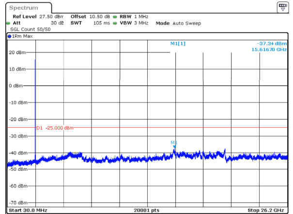
n38_5MHz_15kHz_2595MHz_DFT-s-OFDM QPSK_RB1@0 -37.34dBm
