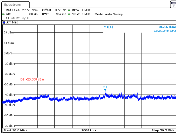
n38_10MHz_30kHz_2615MHz_DFT-s-OFDM QPSK_RB1@23 -36.16dBm
