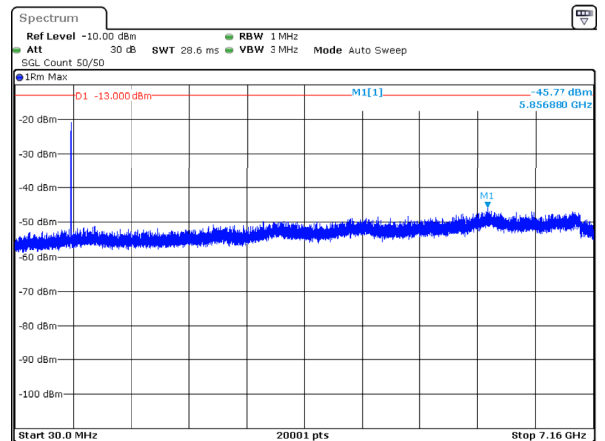
n12_10MHz_15kHz_711MHz_DFT-s-OFDM QPSK_RB50@0 -45.77dBm
