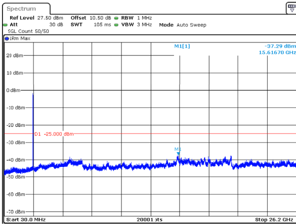
n38_10MHz_30kHz_2595MHz_DFT-s-OFDM QPSK_RB24@0 -37.29dBm
