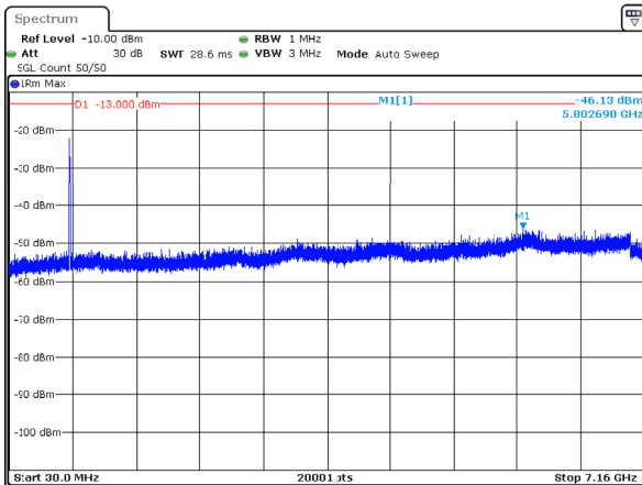
n12_10MHz_15kHz_707.5MHz_DFT-s-OFDM QPSK_RB50@0 -46.13dBm
