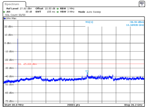
n38_10MHz_30kHz_2615MHz_DFT-s-OFDM QPSK_RB1@0 -36.94dBm
