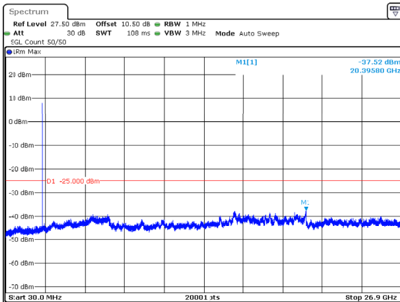
n41_10MHz_30kHz_2501.01MHz_DFT-s-OFDM QPSK_RB1@23 -37.52dBm
