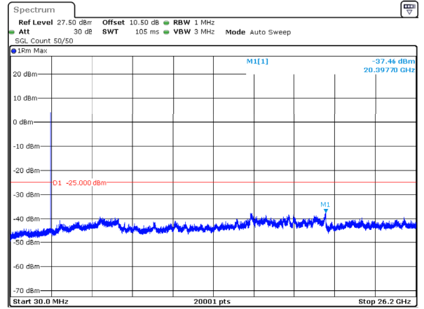
n38_40MHz_30kHz_2600MHz_DFT-s-OFDM QPSK_RB1@0 -37.46dBm
