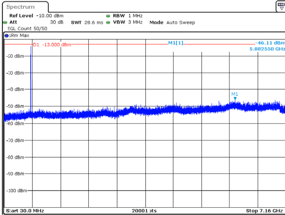
n12_10MHz_15kHz_707.5MHz_DFT-s-OFDM QPSK_RB1@0 -46.11dBm
