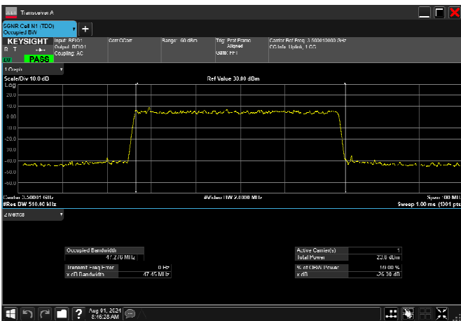
n78_1_50MHz_30kHz_3500MHz_DFT-s-OFDM QPSK_RB128@0 47.276MHz
