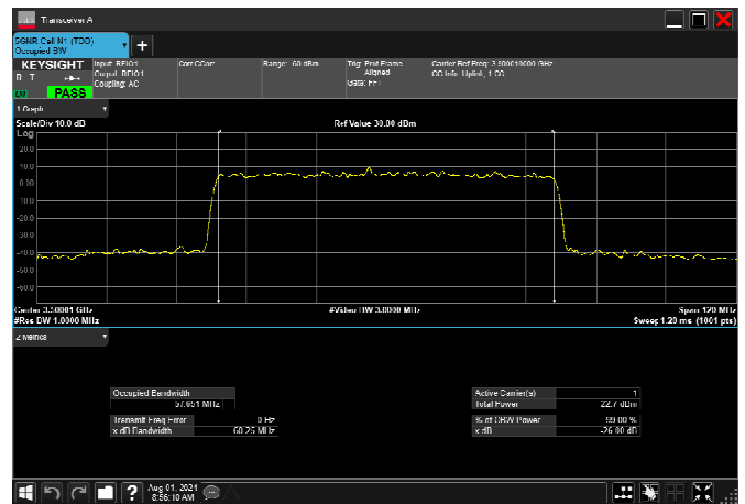
n78_1_60MHz_30kHz_3500MHz_CP-OFDM QPSK_RB162@0 57.651MHz
