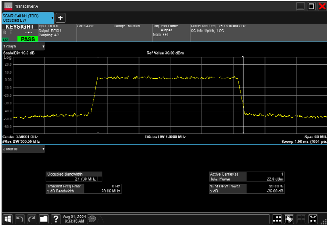
n78_1_30MHz_30kHz_3500MHz_CP-OFDM QPSK_RB78@0 27.859MHz
