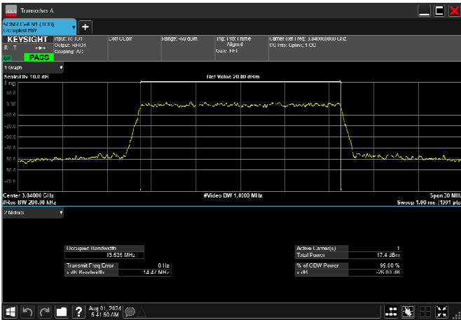
n77_3_20MHz_30kHz_3840MHz_DFT-s-OFDM QPSK_RB50@0 18.081MHz
