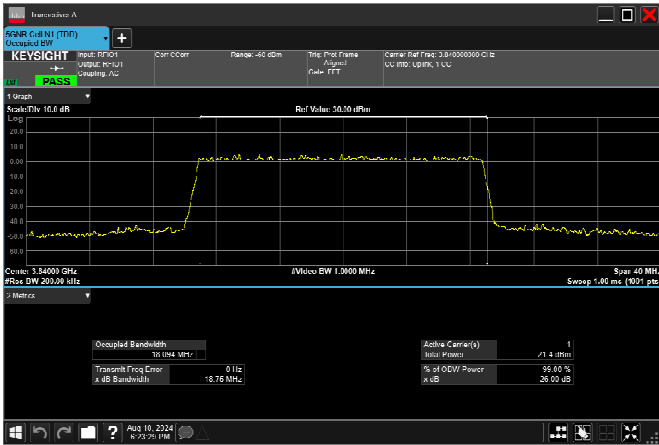
n77_3_20MHz_30kHz_3840MHz_CP-OFDM QPSK_RB51@0 18.181MHz
