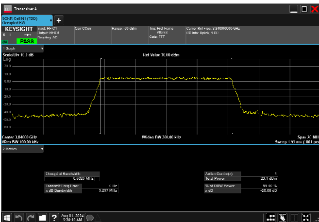
n77_3_10MHz_30kHz_3840MHz_DFT-s-OFDM QPSK_RB24@0 8.562MHz
