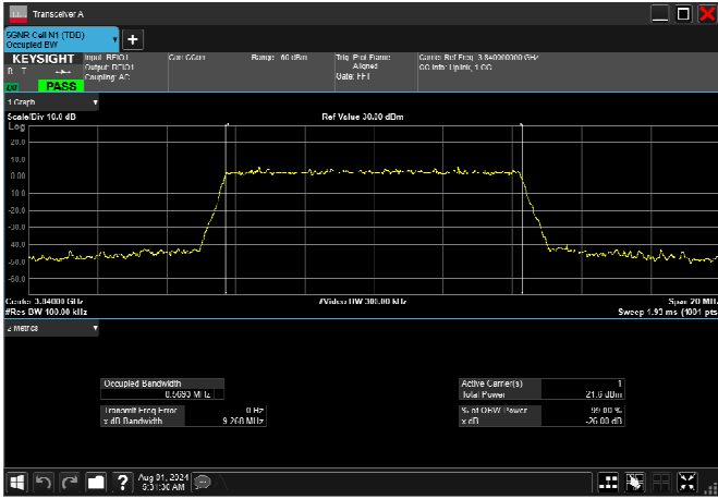
n77_3_10MHz_30kHz_3840MHz_CP-OFDM QPSK_RB24@0 8.566MHz
