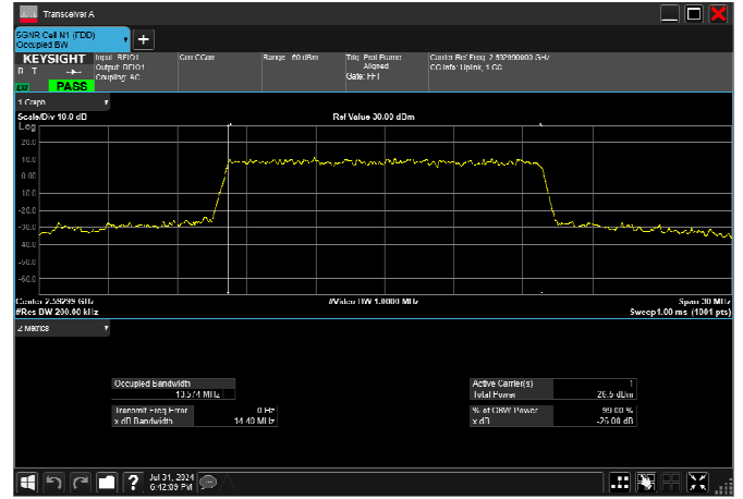
n41_20MHz_30kHz_2592.99MHz_DFT-s-OFDM \pi/2 BPSK_RB50@0 18.098MHz
