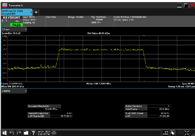
n41_20MHz_30kHz_2592.99MHz_DFT-s-OFDM QPSK_RB50@0 18.030MHz
