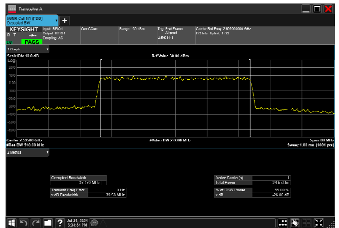
n38_40MHz_30kHz_2595MHz_CP-OFDM QPSK_RB106@0 37.770MHz
