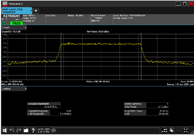
n41_10MHz_30kHz_2592.99MHz_CP-OFDM QPSK_RB24@0 8.539MHz
