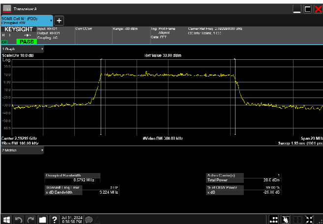
n41_10MHz_30kHz_2592.99MHz_DFT-s-OFDM QPSK_RB24@0 8.579MHz
