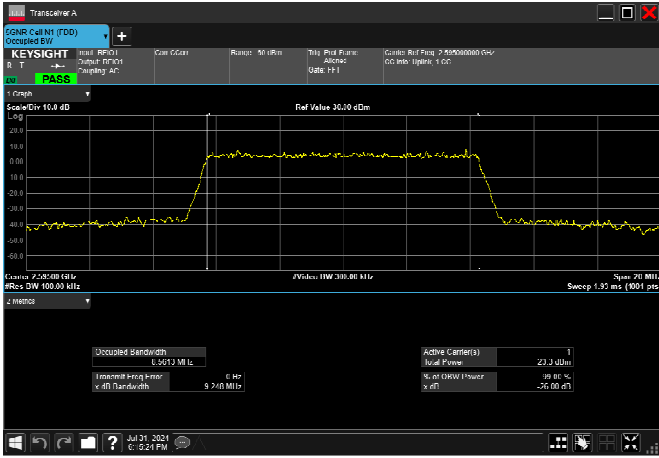
n38_10MHz_30kHz_2595MHz_CP-OFDM QPSK_RB24@0 8.576MHz
