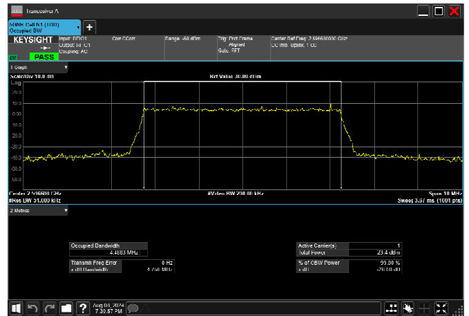
n38_5MHz_15kHz_2595MHz_CP-OFDM QPSK_RB25@0 4.466MHz
