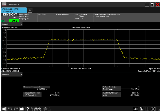
n38_5MHz_15kHz_2595MHz_DFT-s-OFDM 256 QAM_RB25@0 4.463MHz
